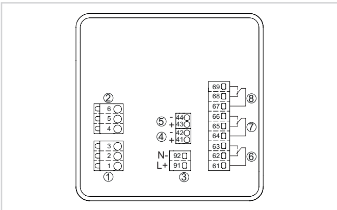
VEGAMET 342 的接线图
