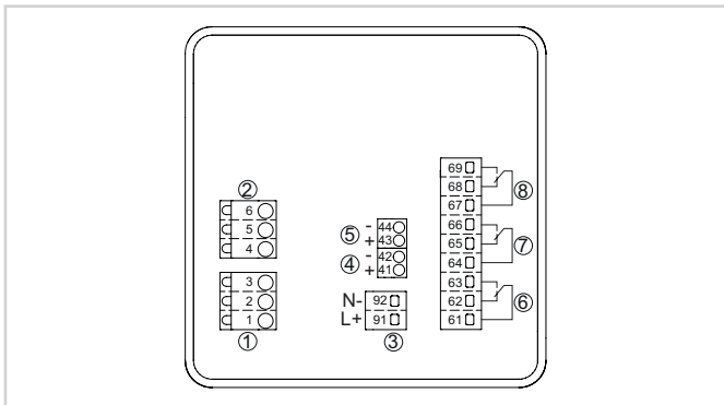
Esquema de ligações VEGAMET 342
