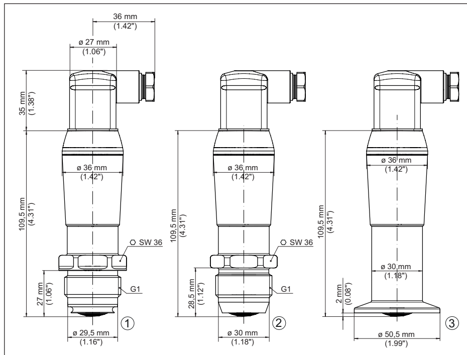
Fig. 21: VEGAPOINT 24, hygiënische uitvoering - schroefdraad met ISO 4400-stekker
