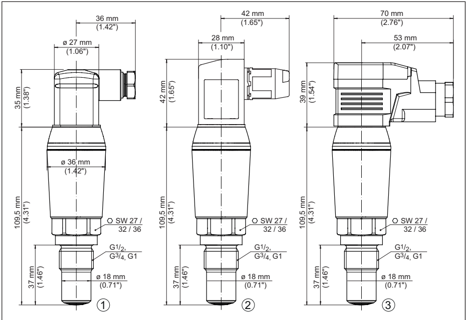
Fig. 20: VEGAPOINT 24, standaarduitvoering - schroefdraad met ventielstekkers conform ISO 4400
