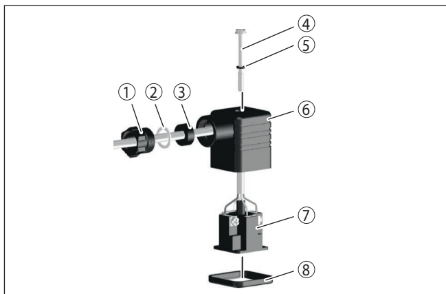
Fig. 9: Aansluiting ventielstekker ISO 4400
