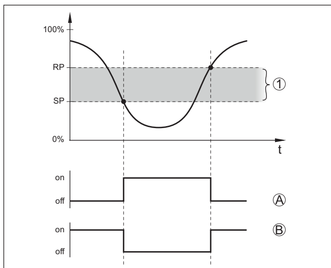
Fig. 14: Hysteresefunctie
