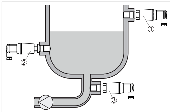
Fig. 4: Inbouwvoorbeelden
