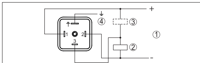
Fig. 13: Aansluitschema stekker ISO 4400 - transistoruitgang driedraads
