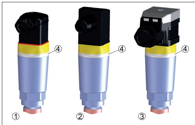
Fig. 8: Stekkeruitvoeringen
