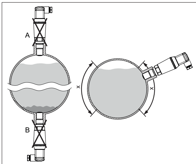
Fig. 6: Montage in horizontale leidingen
