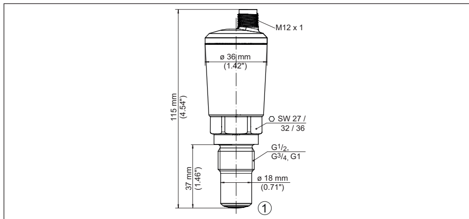
Abb. 15: VEGAPOINT 24, Standardausführung - Gewinde mit M12 x 1-Stecker
