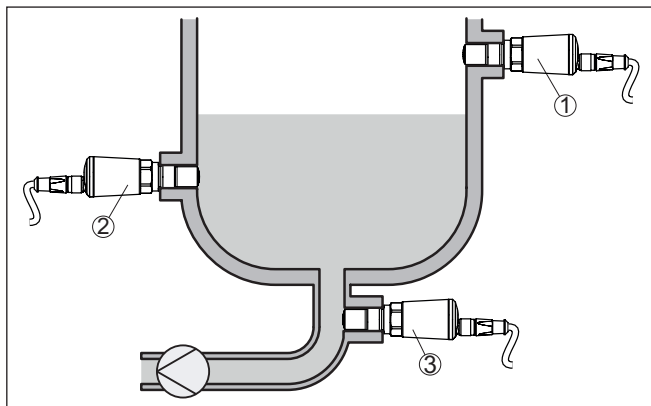
Abb. 3: Einbaubeispiele
