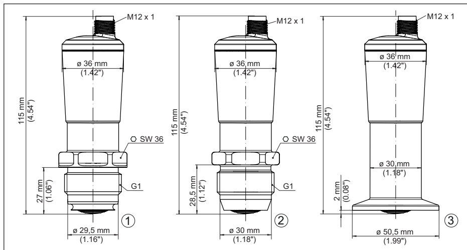
Abb. 16: VEGAPOINT 24, Hygieneausführung - Gewinde, mit M12 x 1-Stecker
