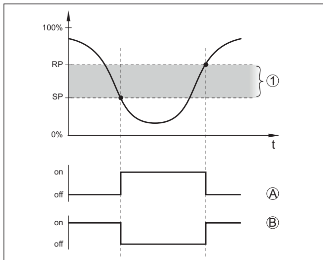
Abb. 9: Hysterese-Funktion
