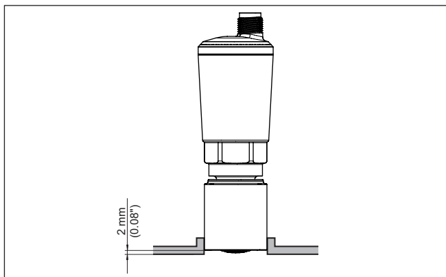
Abb. 6: VEGAPOINT 24 2 mm (0.08 in) rückgesetzt in Lebensmittelanwendung
