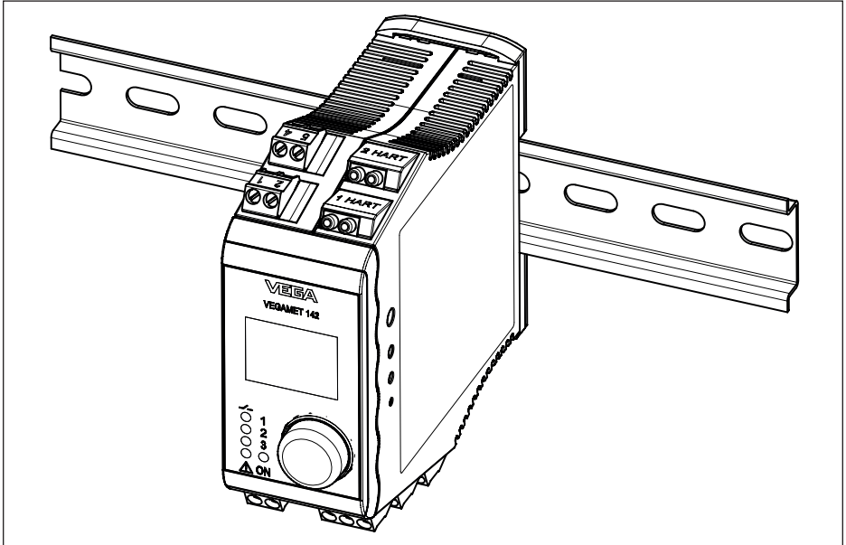
図 1: VEGAMET 141, 142 キャリアレールに取り付け
