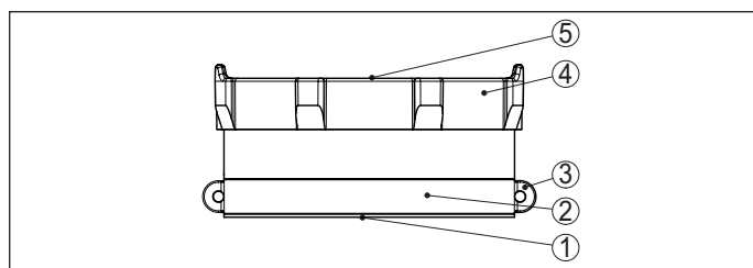
Fig. 5: Composants du capteur VEGAPULS Air (exemple de version avec fixation adhésive)
