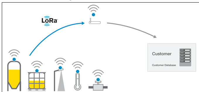
Fig. 19: Draadloze meetwaardeoverdracht
