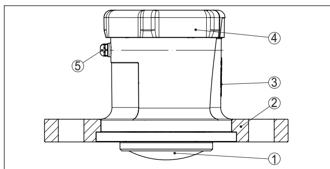
Fig. 7: Componenten van de radarsensor VEGAPULS Air 42 (voorbeeld uitvoering met overschuifflens DN 80)
