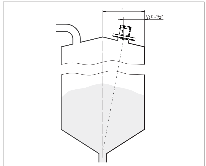
Fig. 11: Montagepositie en uitlijning
