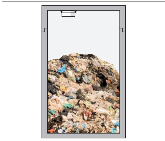
Fig. 13: Niveaumeting met VEGAPULS Air 23 in afvalsilo
