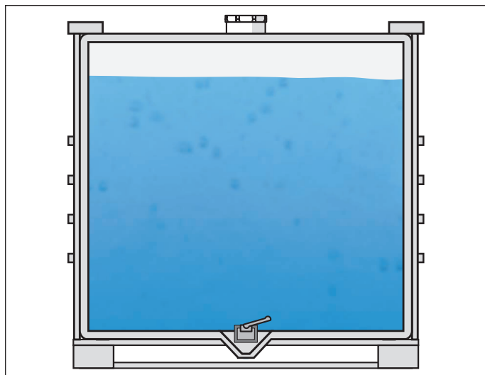
Fig. 12: Niveaumeting met VEGAPULS Air 23 in IBC-container
