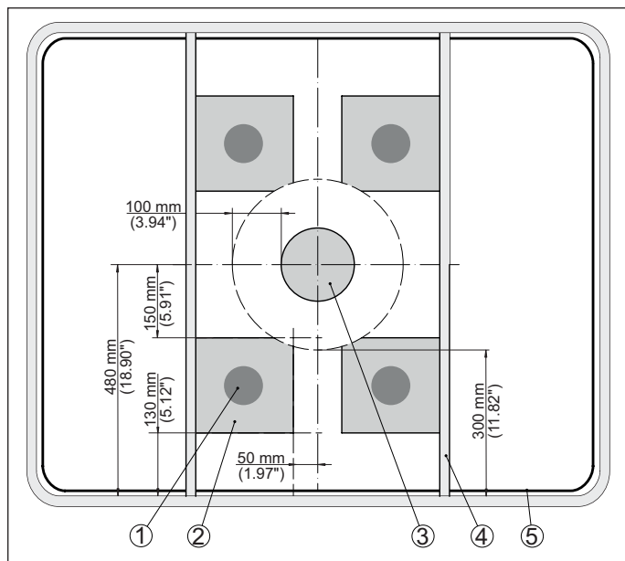
Fig. 8: Posición de montaje sobre la tapa del depósito
