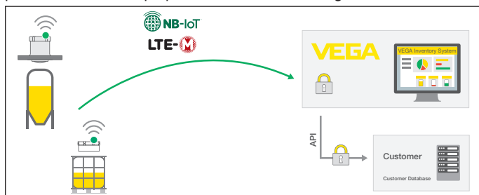
Fig. 16: Transmisión inalámbrica de valores de medición a través de NB-IoT y LTE-M al VEGA Inventory System
