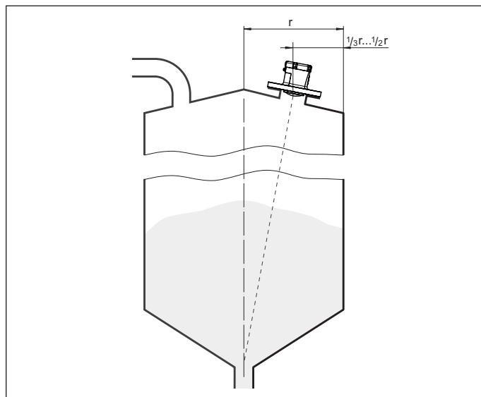
Fig. 11: Posición de montaje y alineación
