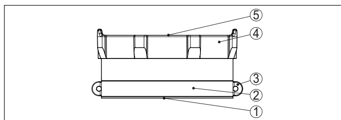
Fig. 5: Componentes del sensor VEGAPULS Air (versión con unión adhesiva como ejemplo)
