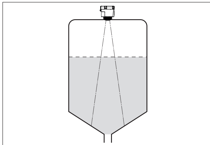
Fig. 10: Montaje del sensor de radar en depósito con fondo cónico
