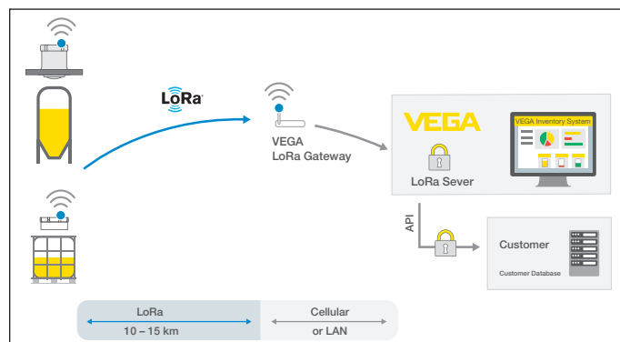
Fig. 17: Transmisión inalámbrica de valores de medición a través de LoRaWAN, servidor LoRa al VEGA Inventory System
