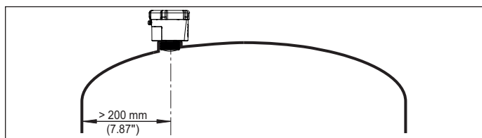
Fig. 9: Montaje del sensor en tapas de depósito redondas
