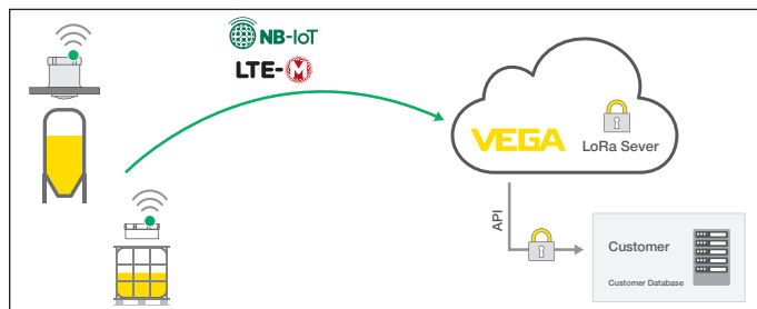
Fig. 18: Transmisión inalámbrica de valores de medición a través de NB-IoT y LTE-M a la nube VEGA
