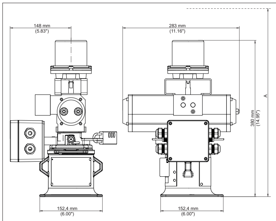
Figura 41: Contenitore di protezione VEGASOURCE 81, esecuzione B - commutazione pneumatica, con interruttori di posizione ON/OFF
