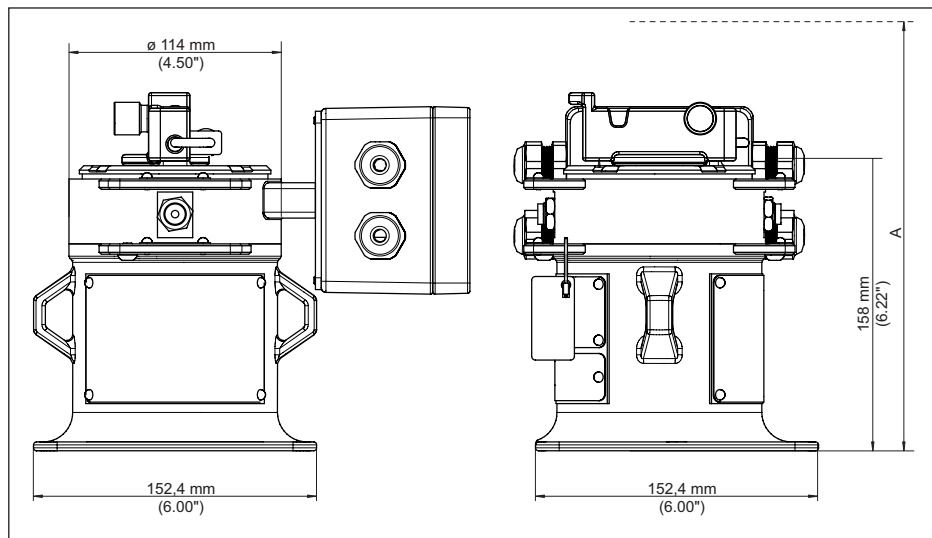
Figura 38: Contenitore di protezione VEGASOURCE 81, esecuzione X, C - commutazione manuale, con interruttori di posizione ON/OFF
