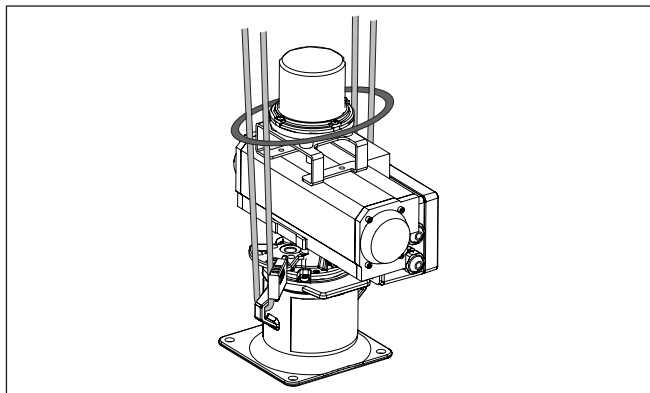
Figura 8: Sollevamento di un contenitore di protezione con commutazione pneumatica
