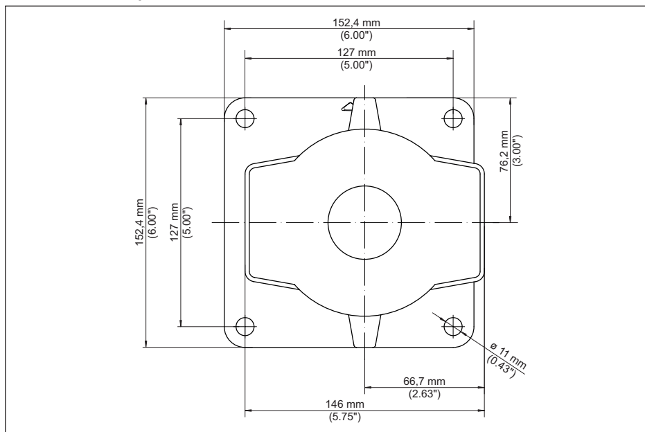
Figura 43: Piastra di base con fori (per es. esecuzione X, C)
