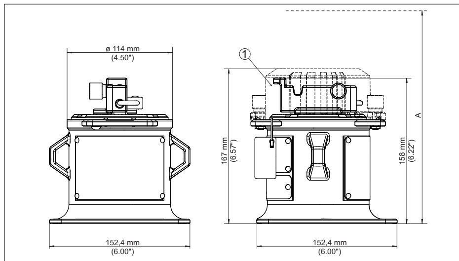
Figura 37: Contenitore di protezione VEGASOURCE 81, esecuzione X, C - commutazione manuale
