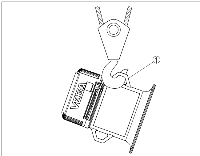
Figura 9: Trasporto con la gru del contenitore di protezione
