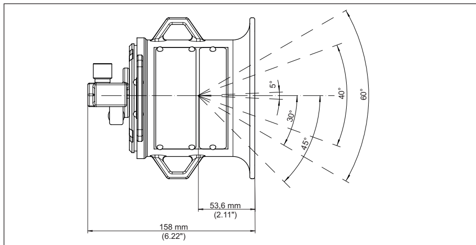
Figura 42: Canale di diffusione dei raggi (per es. esecuzione X, C)
