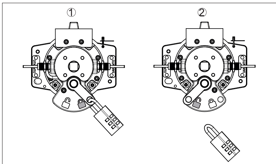
Figura 28: Visualizzazione dello stato di commutazione del VEGASOURCE 81 - esecuzione B - commutazione pneumatica
