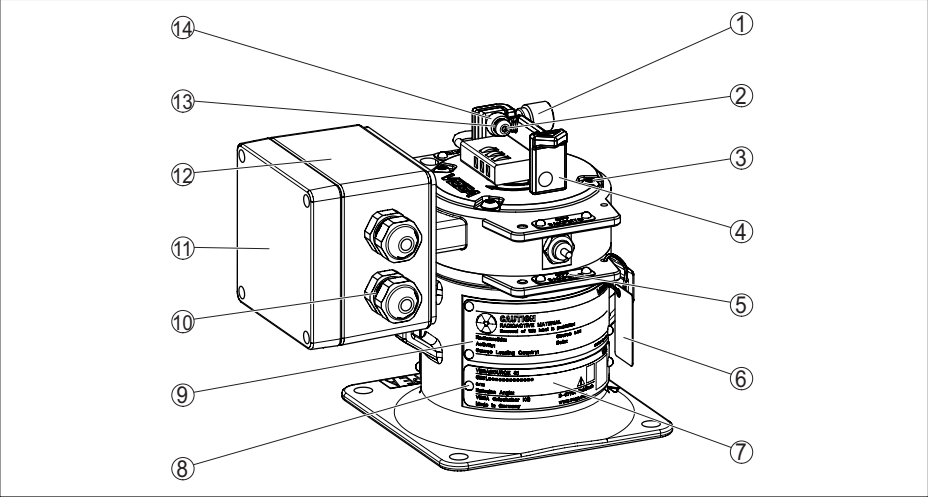
Figura 32: Materiali VEGASOURCE 81 - esecuzione X, C - con interruttori di posizione ON/OFF
