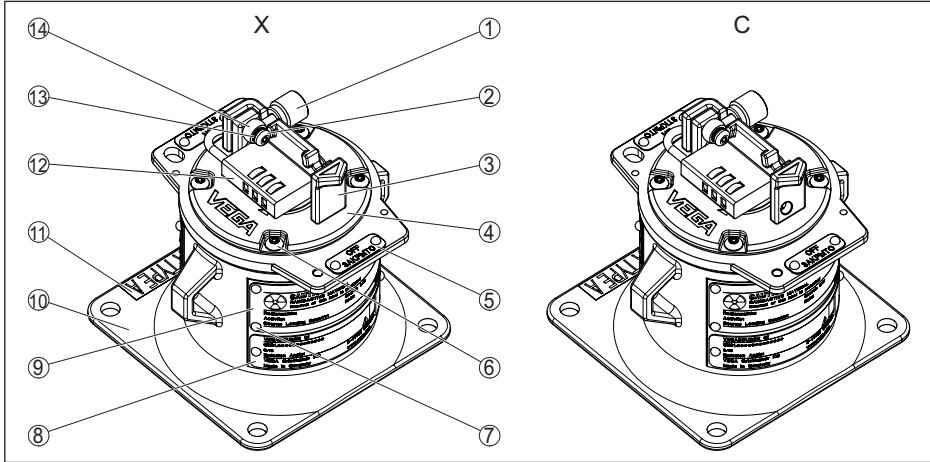
Figura 31: Materiali VEGASOURCE 81 - esecuzione X, C
