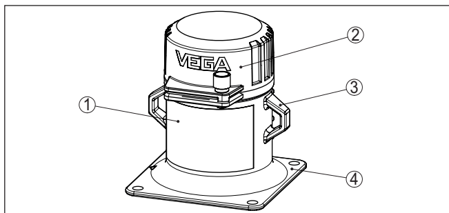
Figura 6: Contenitore di protezione VEGASOURCE 81
