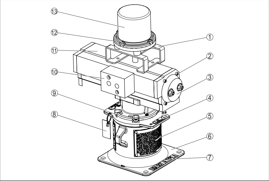
Figura 34: Materiali VEGASOURCE 81 - esecuzione B
