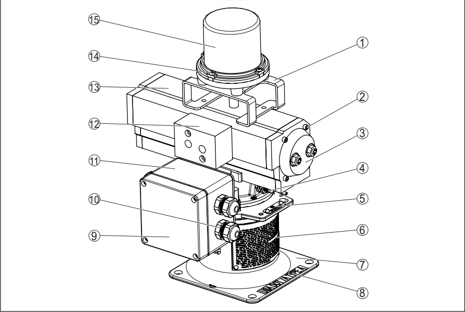
Figura 35: Materiali VEGASOURCE 81 - esecuzione B - con interruttori di posizione ON/OFF
