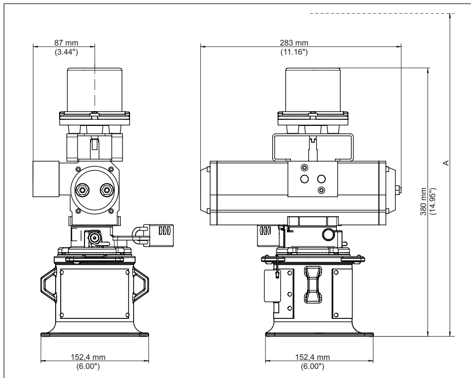
Figura 40: Contenitore di protezione VEGASOURCE 81, esecuzione B - commutazione pneumatica
