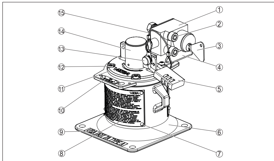
Figura 33: Materiali VEGASOURCE 81 - esecuzione X, C - con interruttore di interblocco
