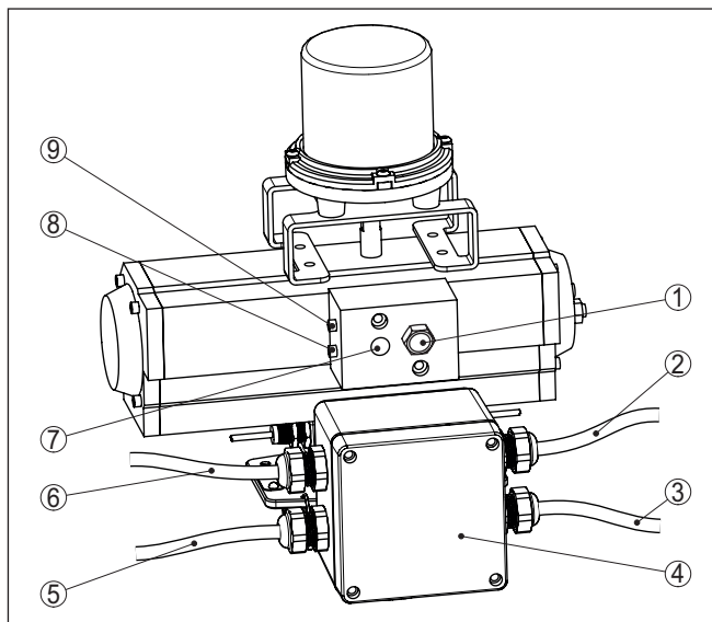
Figura 22: Allacciamento delle condotte dell'aria compressa al VEGASOURCE 81 - esecuzione B
