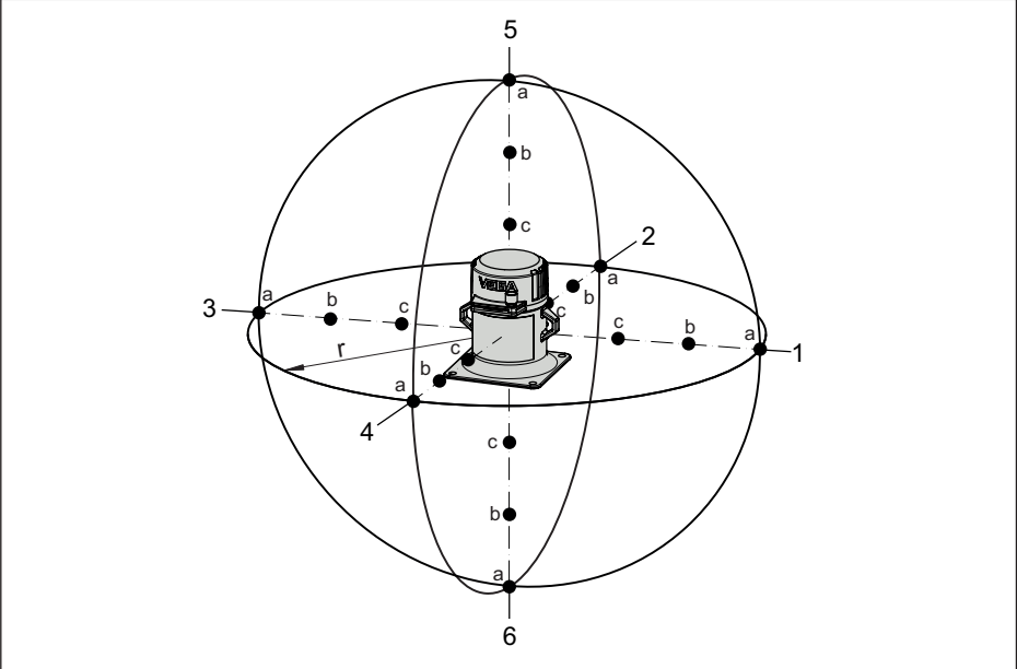
Figura 36: Curva di isodistanza (distanza: 1 m) - esempio: contenitore di protezione VEGASOURCE 81 con Cs-137, 20 mCi (740 MBq)
