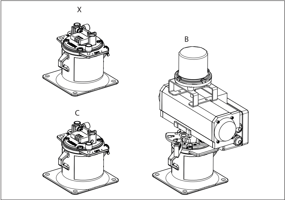
Figura 2: Modelli di VEGASOURCE 81 (panoramica)
