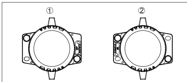
Figura 27: Visualizzazione della posizione con calotta di protezione - VEGA-SOURCE 81 esecuzione X, C
