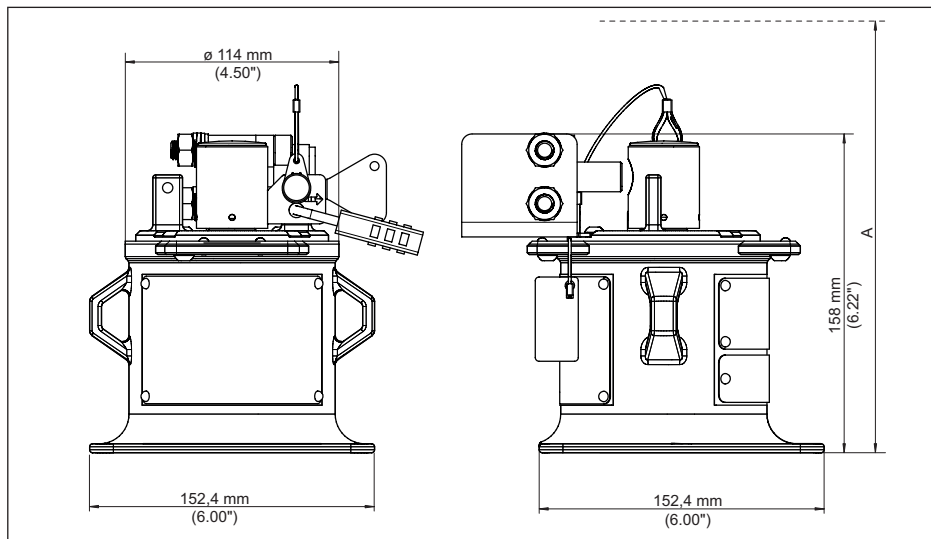
Figura 39: Contenitore di protezione VEGASOURCE 81, esecuzione X, C - commutazione manuale, con interruttore di interblocco
