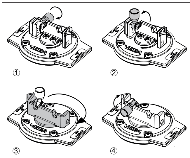
Figura 24: Attivazione dell'irraggiamento - VEGASOURCE 81 esecuzione X, C
