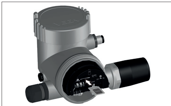
Abb. 17: Mini-SIM-Karte einsetzen
