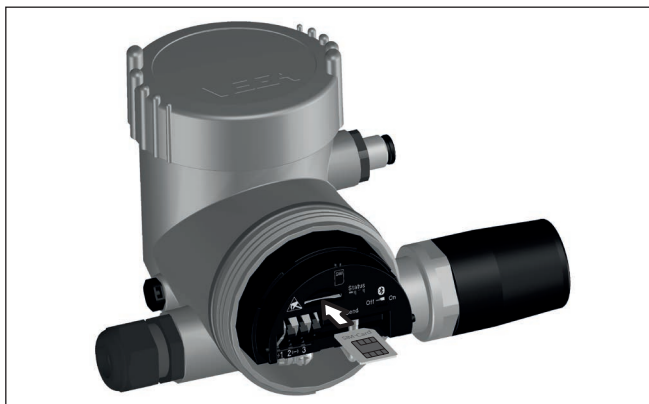
Abb. 17: Mini-SIM-Karte einsetzen
