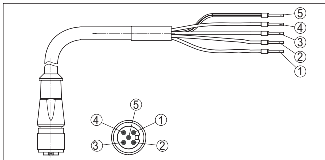
Abb. 9: Anschlussbelegung Sensorverbindungskabel
