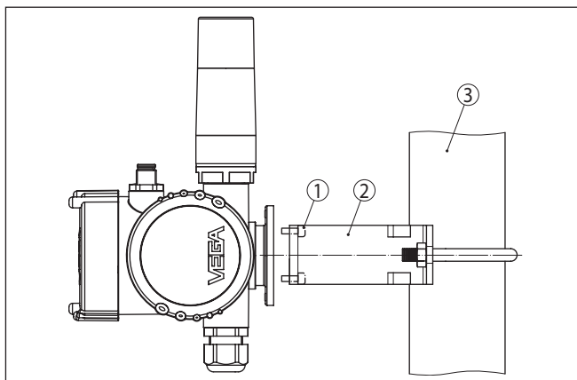
Abb. 4: PLICSMOBILE T81 zur Rohrmontage
