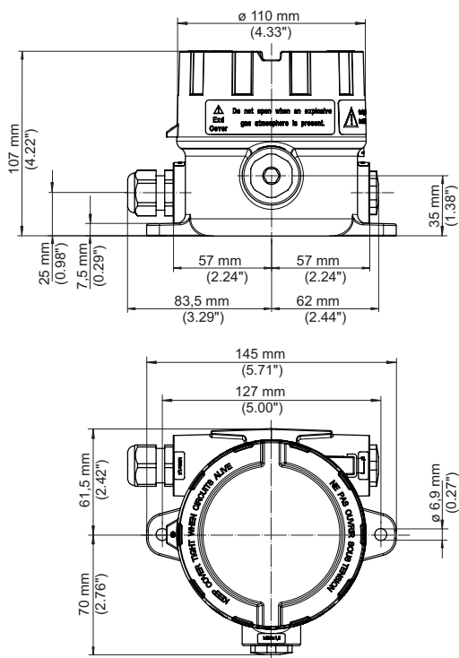
Fig. 21: Afmetingen PLICSMOBILE B81 met aluminium behuizing
