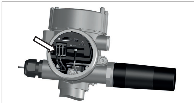
Fig. 5: Aansluitstappen 4 en 5
