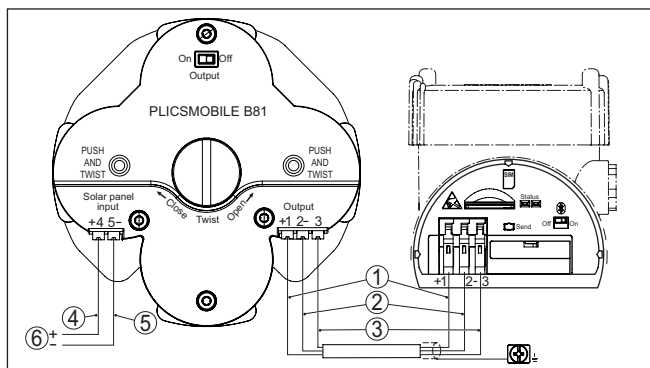
Fig. 12: Aansluiting van de PLICSMOBILE B81/S81
