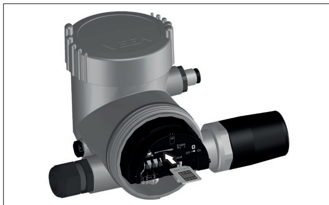
Fig. 17: Mini-SIM-kaart plaatsen
