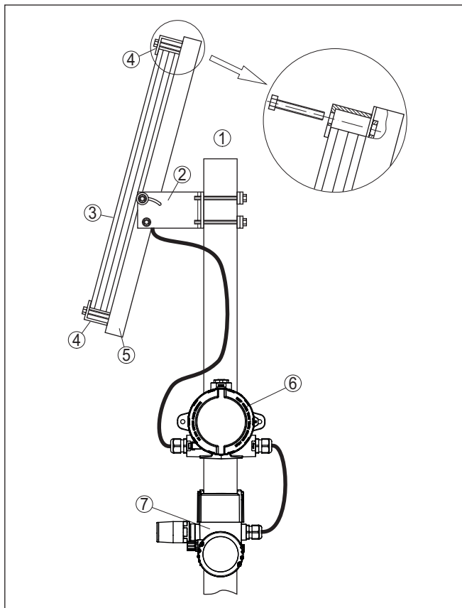
Fig. 13: Pijpmontage PLICSMOBILE met solarmodule
