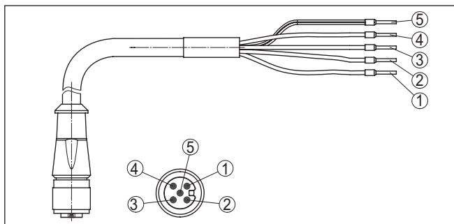
Fig. 9: Aansluitbezetting sensorverbindingskabel
