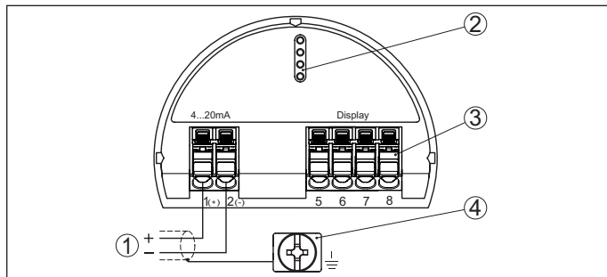
Abb. 5: Elektronik- und Anschlussraum - Einkammergehäuse
