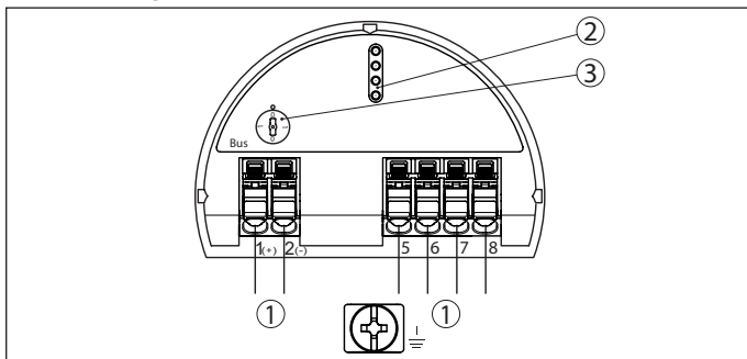
Abb. 18: Elektronik- und Anschlussraum - Einkammergehäuse
