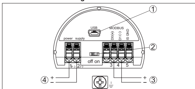
Abb. 21: Anschlussraum - Zweikammergehäuse
