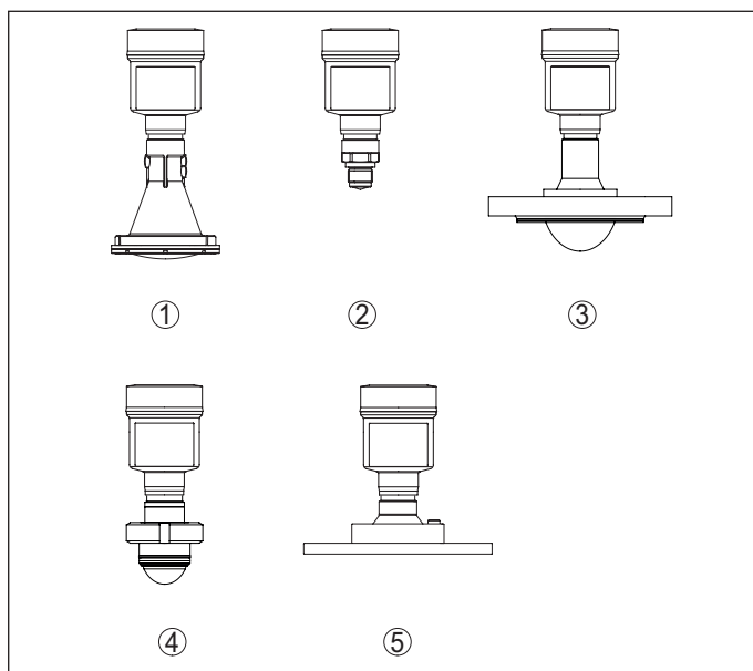
Abb. 3: Antennensysteme VEGAPULS 6X für Standardanwendungen
