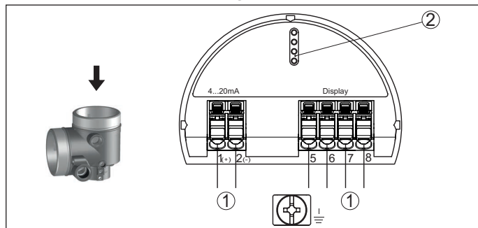
Abb. 12: Elektronikraum - Zweikammergehäuse
