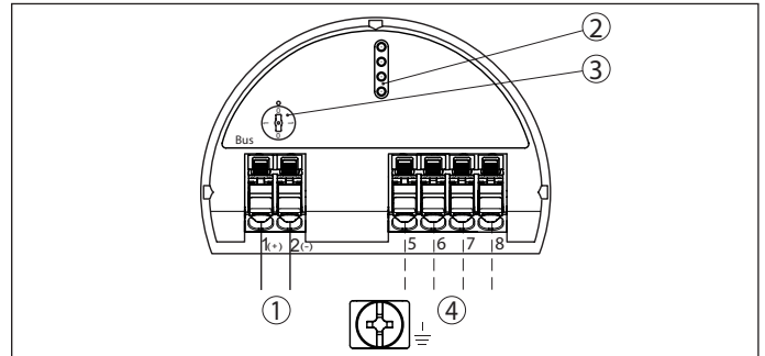
Abb. 19: Elektronikraum - Zweikammergehäuse
