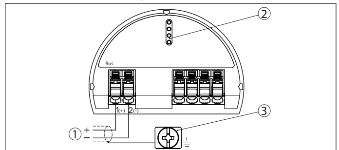
Abb. 20: Anschlussraum - Zweikammergehäuse
