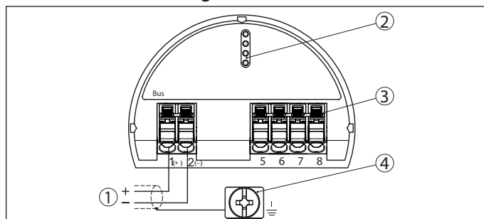
Abb. 17: Anschlussraum Zweikammergehäuse
