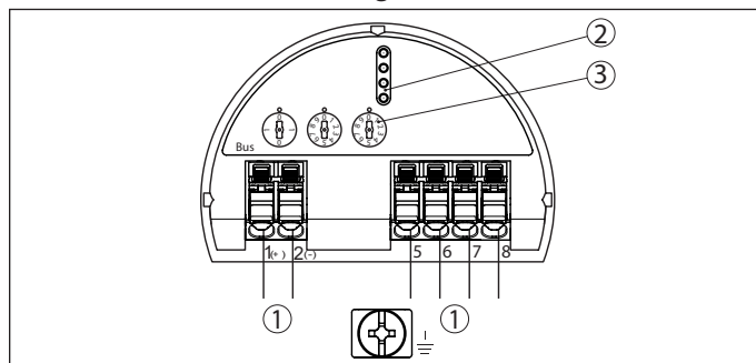
Abb. 16: Elektronikraum - Zweikammergehäuse
