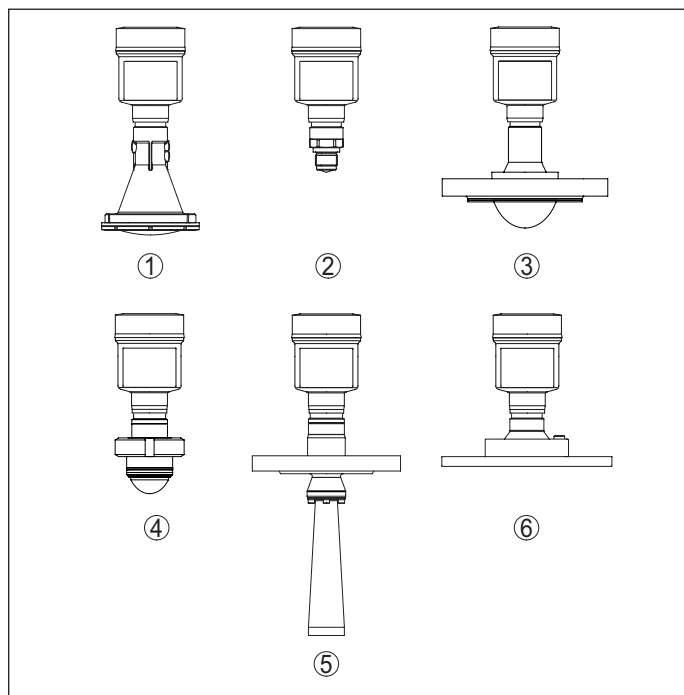
插图 3: 天线系统 VEGAPULS 6X 用于标准应用场合
