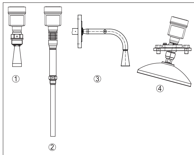
插图 4: 天线系统 VEGAPULS 6X 适用于特殊应用场合
