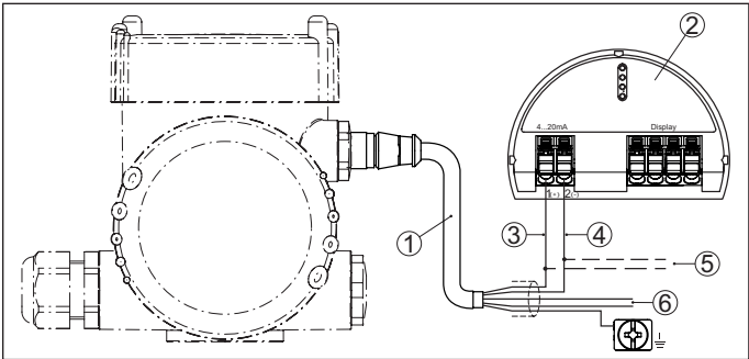
插图 11: 其他 plics® 传感器的连接
