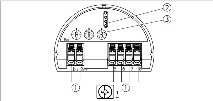
插图. 16: 双腔式外壳的电子部件腔
