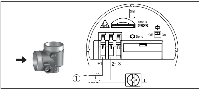
插图 10: 接线腔 - 无线模块 PLICSMOBILE 81
