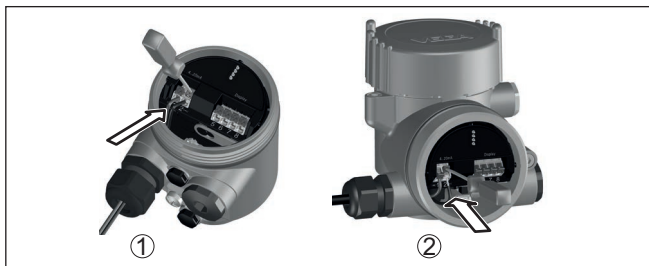
Abb. 6: Anschlusschritte 5 und 6
