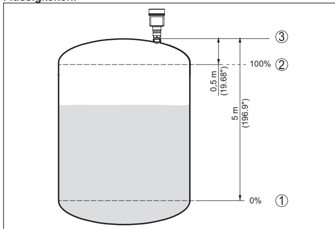
Abb. 10: Parametrierbeispiel Min.-/Max.-Abgleich - Flüssigkeiten
