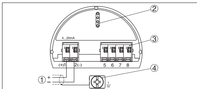
Figura 6: Vano dell'elettronica e di connessione - custodia a una camera
