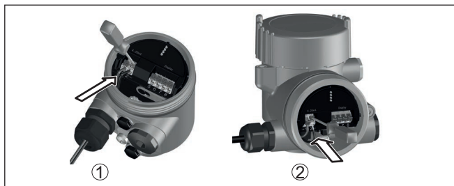
Figura 5: Operazioni di collegamento 5 e 6
