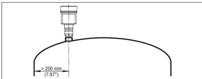
Fig. 2: Montage van de radarsensor op ronde tankdaken
