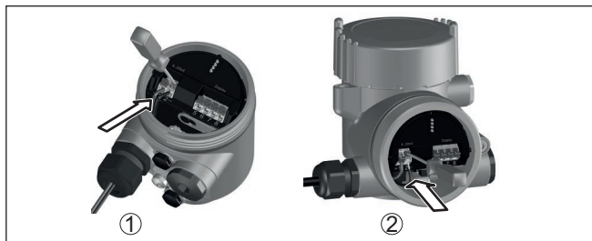
Fig. 5: Aansluitstappen 5 en 6
