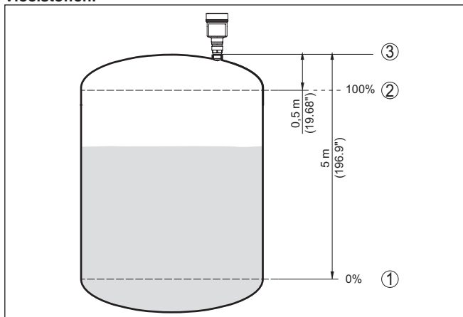
Fig. 9: Parametreervoorbeeld min.-/max.-inregeling - vloeistoffen
