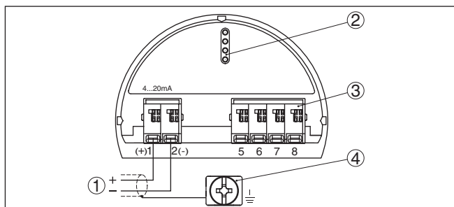
Fig. 6: Elektronica- en aansluitruimte - eenkamerbehuizing
