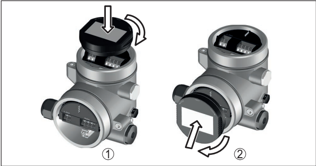
插图. 9: 将显示和调整模块装到双腔式壳体上
