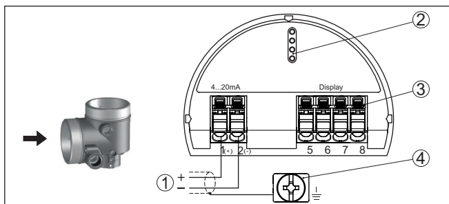
插图. 8: 双腔式外壳的接线腔
