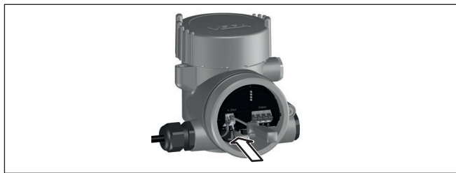
插图. 6: 接线步骤5和6
