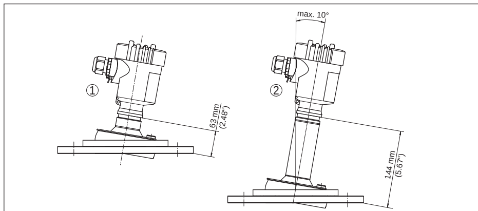
插图. 104: VEGAPULS 6X, 带有透镜天线和万向节的法兰
