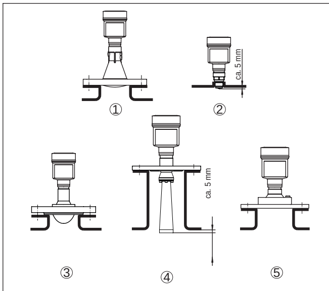
插图. 25: 对于不同版本的 VEGAPULS 6X 的安装管接头的推荐参数
