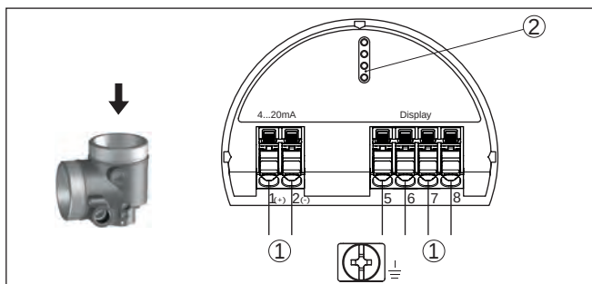
插图. 48: 双腔式外壳的电子部件腔
