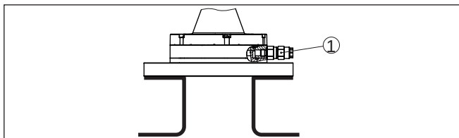
插图. 41: 带适配法兰的塑料号角天线
