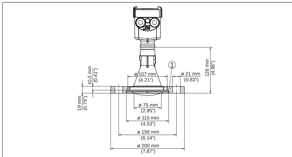
插图. 86: 雷达传感器，带有锁紧法兰，适用于 3" 150 lbs, DN 80, PN 16
