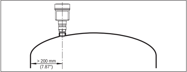
插图. 18: 将雷达传感器安装在圆形容器盖上
