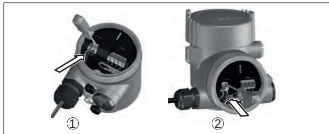
插图. 46: 接线步骤5和6
