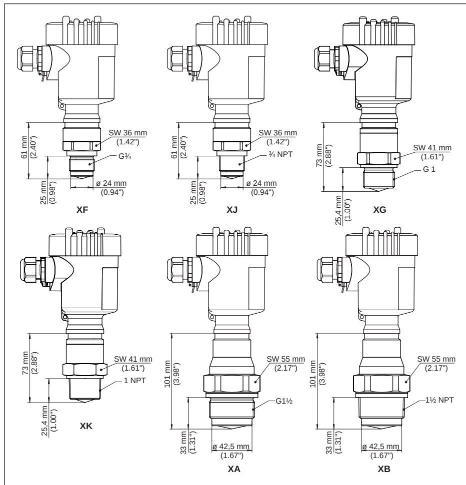
插图 92: VEGAPULS 6X, 带有内置天线系统的螺纹, 至 +150 °C (+302 °F)
