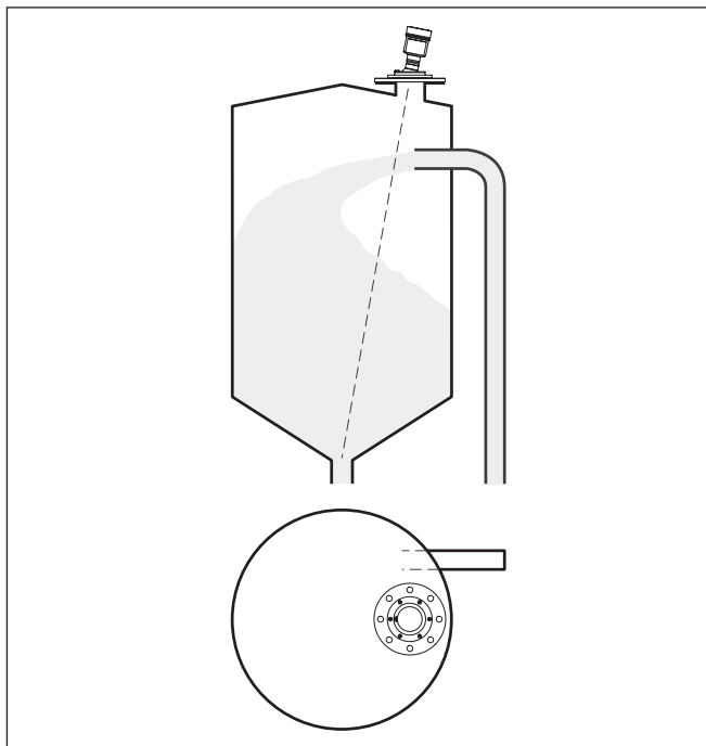
插图. 24: 当从侧面充填介质时雷达传感器的安装
