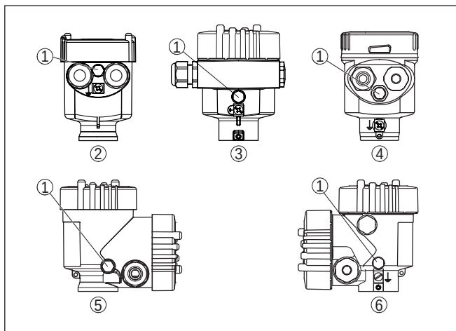
插图. 6: 过滤元件的位置视壳体而定
