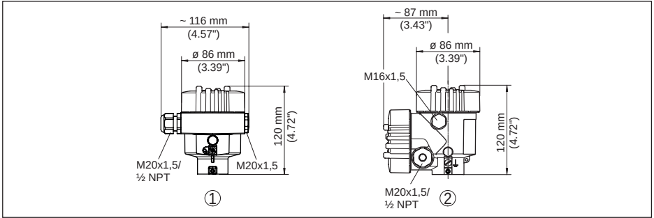
插图. 82: 采用防护等级达 IP66/IP68 (0.2 bar) 的壳体版本，(内装显示和调整模块后，壳体高度增加了18 mm/0.71 in)
