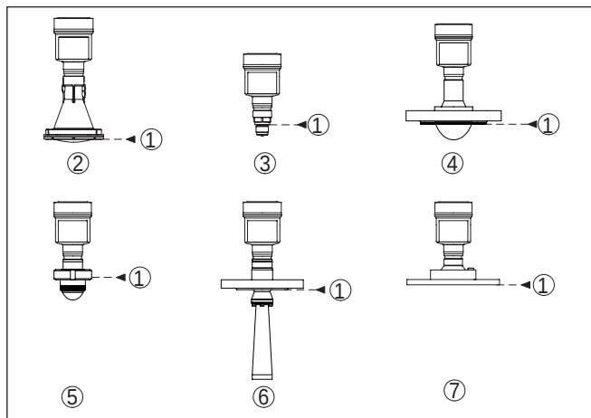
插图. 21: 基准面的位置
