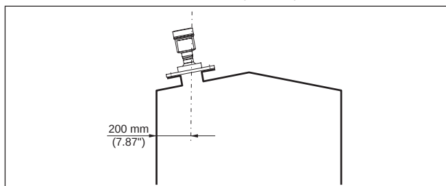
插图. 20: 将雷达传感器安装在容器盖上
