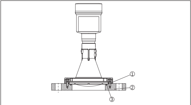
插图. 16: 适配法兰
