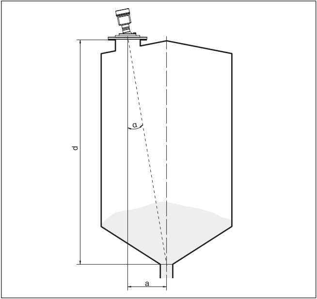
插图. 34: 测定倾斜角度以瞄准 VEGAPULS 6X
