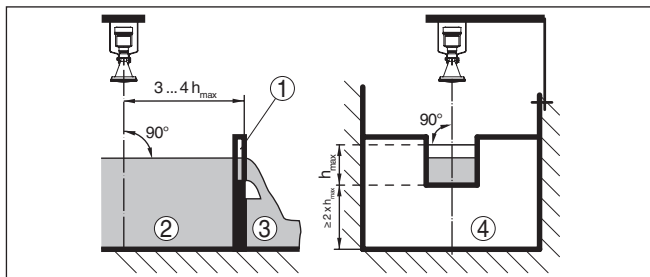
插图. 44: 用矩形槽测量流量: h_{\max} = 矩形槽的最大注水高度
