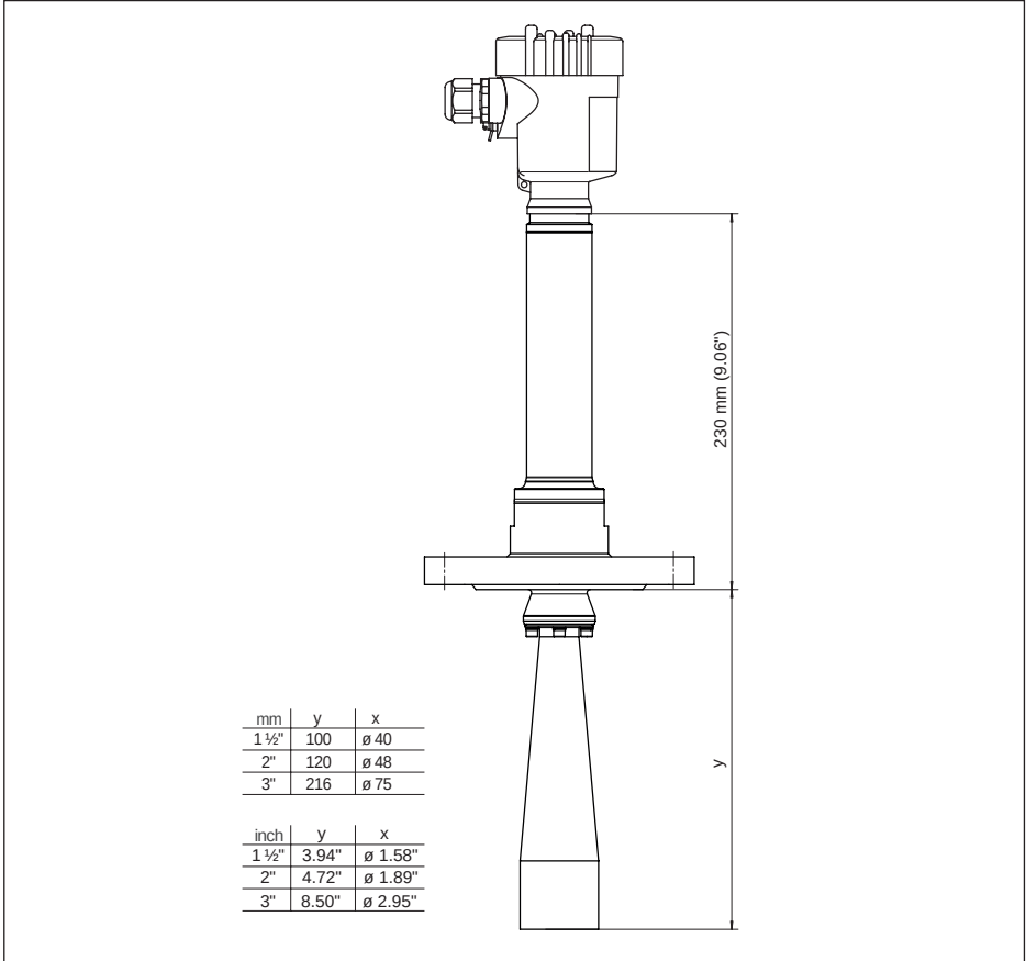
插图. 96: VEGAPULS 6X, 带有号角天线的法兰, 450 °C 型
