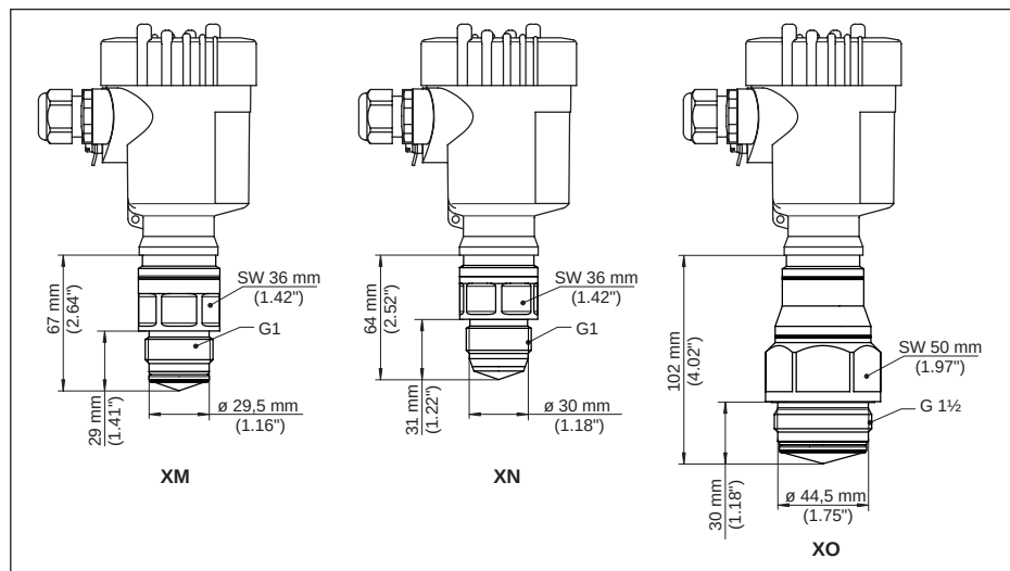
插图. 99: VEGAPULS 6X, 用于卫生型适配器的螺纹
