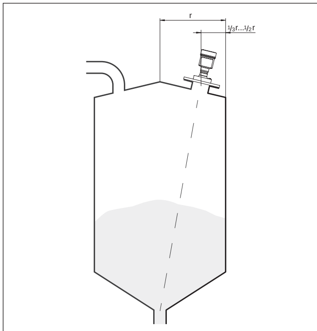
插图. 33: 安装位置和校准
