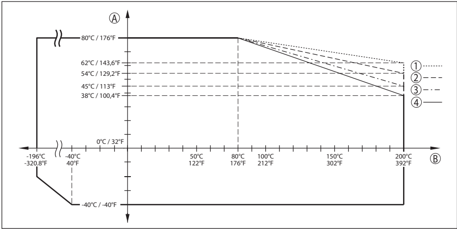
插图. 77: 环境温度降额, 带密封天线系统的法兰 -196 ... +200 °C (-320.8 ... +392 °F)
