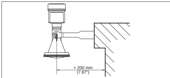
插图. 13: 用长度为 170 毫米的龙门框将仪表水平安装在墙壁上
