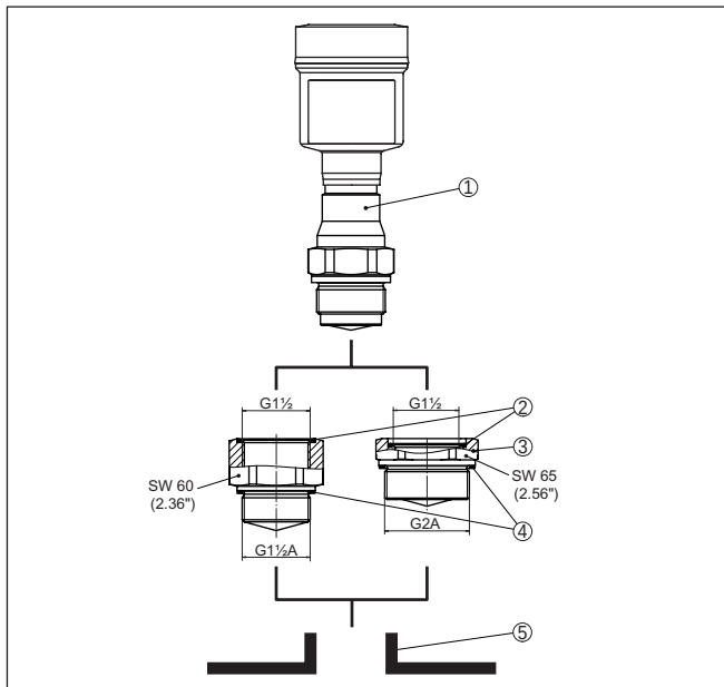
插图. 29: VEGAPULS 6X 带有 PTFE 螺纹适配器 (范例 VEGAPULS 6X 带螺纹 G1½)
