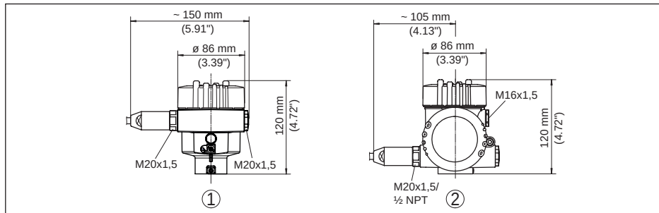
插图 83: 采用防护等级达 IP66/IP68 (1 bar) 的壳体版本 (内装显示和调整模块后, 壳体高度增加了18 mm/0.71 in)
