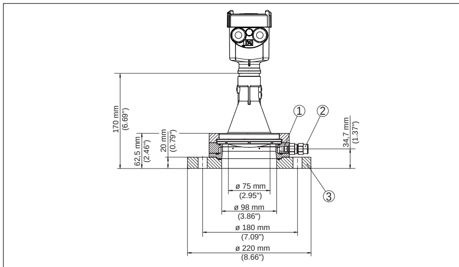
插图. 89: VEGAPULS 6X，适配法兰和吹气接口 DN 100 PN 6
