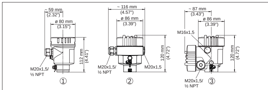
插图 84: 采用防护等级达 IP66/IP68 (0.2 bar) 的壳体版本, (内装显示和调整模块后, 壳体高度增加了18 mm/0.71 in)
