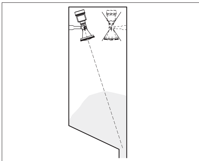
插图. 39: 在多腔式料仓中进行安装和校准
