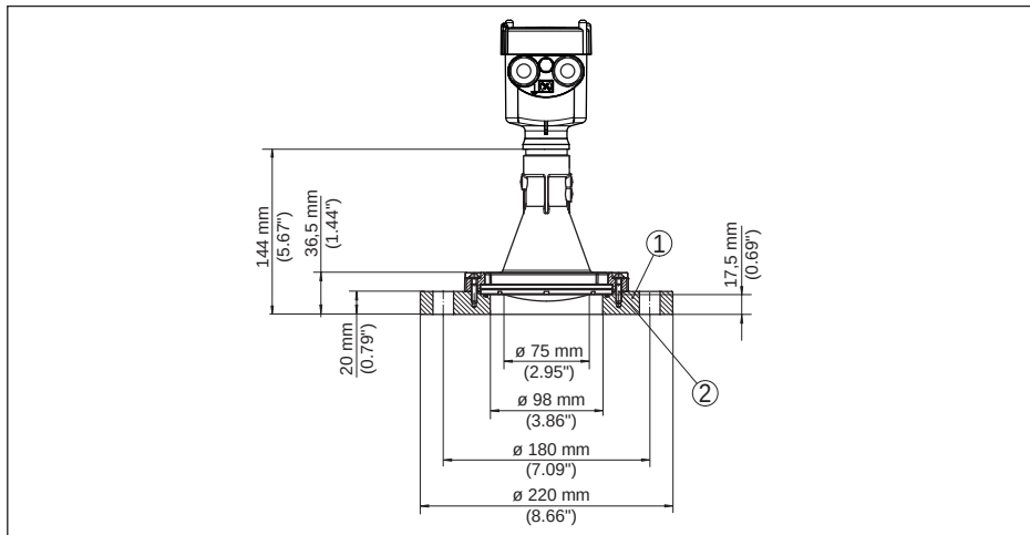
插图. 88: 雷达传感器，带有适配法兰 DN 100 PN 6
