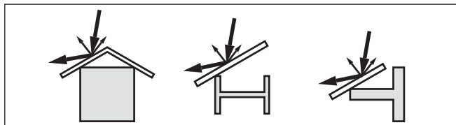
插图. 31: 用散射挡板来覆盖光滑的型材
