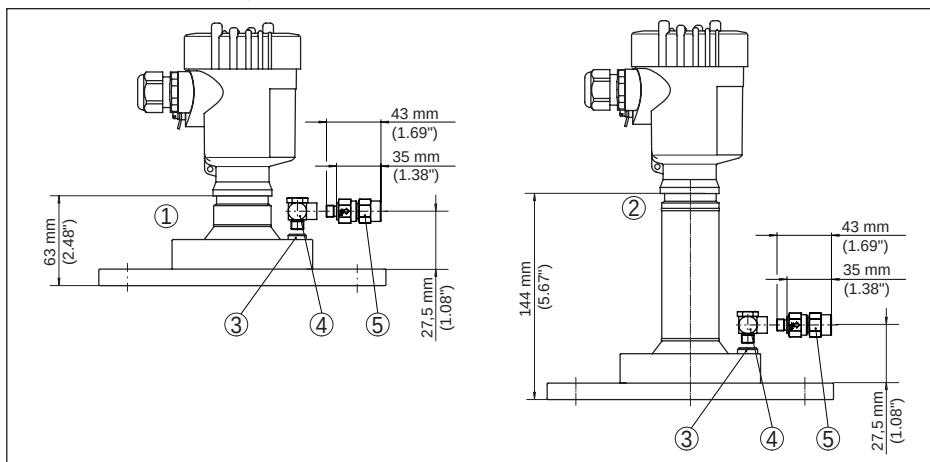
插图. 103: VEGAPULS 6X, 带有透镜天线和吹气接口的法兰
