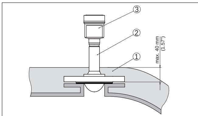
插图. 30: 将仪表安装在绝缘容器上。
