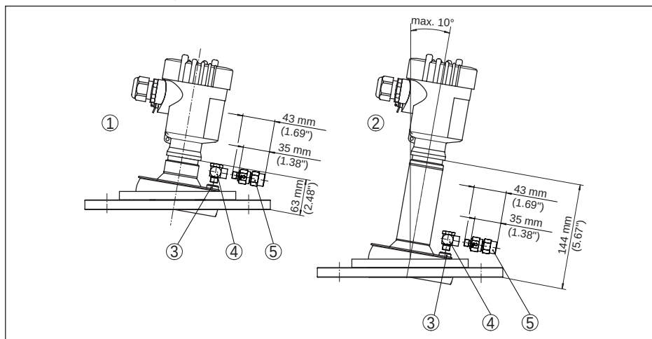
插图. 105: VEGAPULS 6X, 带有透镜天线、万向节和吹气接口的法兰
