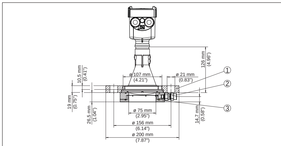
插图. 87: 雷达传感器，带有锁紧法兰和吹气接口，适用于 3" 150 lbs, DN 80 PN 16
