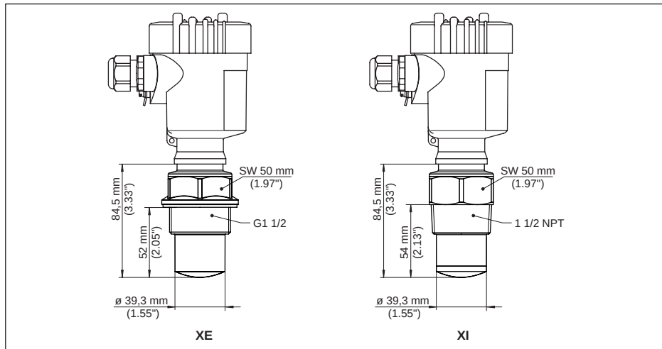
插图. 91: VEGAPULS 6X, 带有内置天线系统的螺纹, 至 +80 °C (+176 °F)
