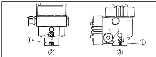
插图. 7: 止动螺钉的位置取决于壳体
