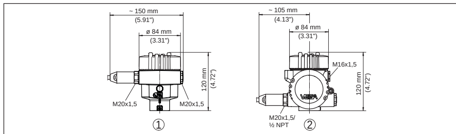
插图 85: 采用防护等级达 IP66/IP68 (1 bar) 的壳体版本 (内装显示和调整模块后, 壳体高度增加了18 mm/0.71 in)
