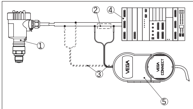
插图. 5: 将电脑与信号线路相连接
