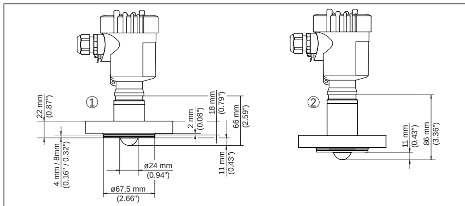
插图: 97: VEGAPULS 6X, 封装天线系统 DN 25 PN 40
