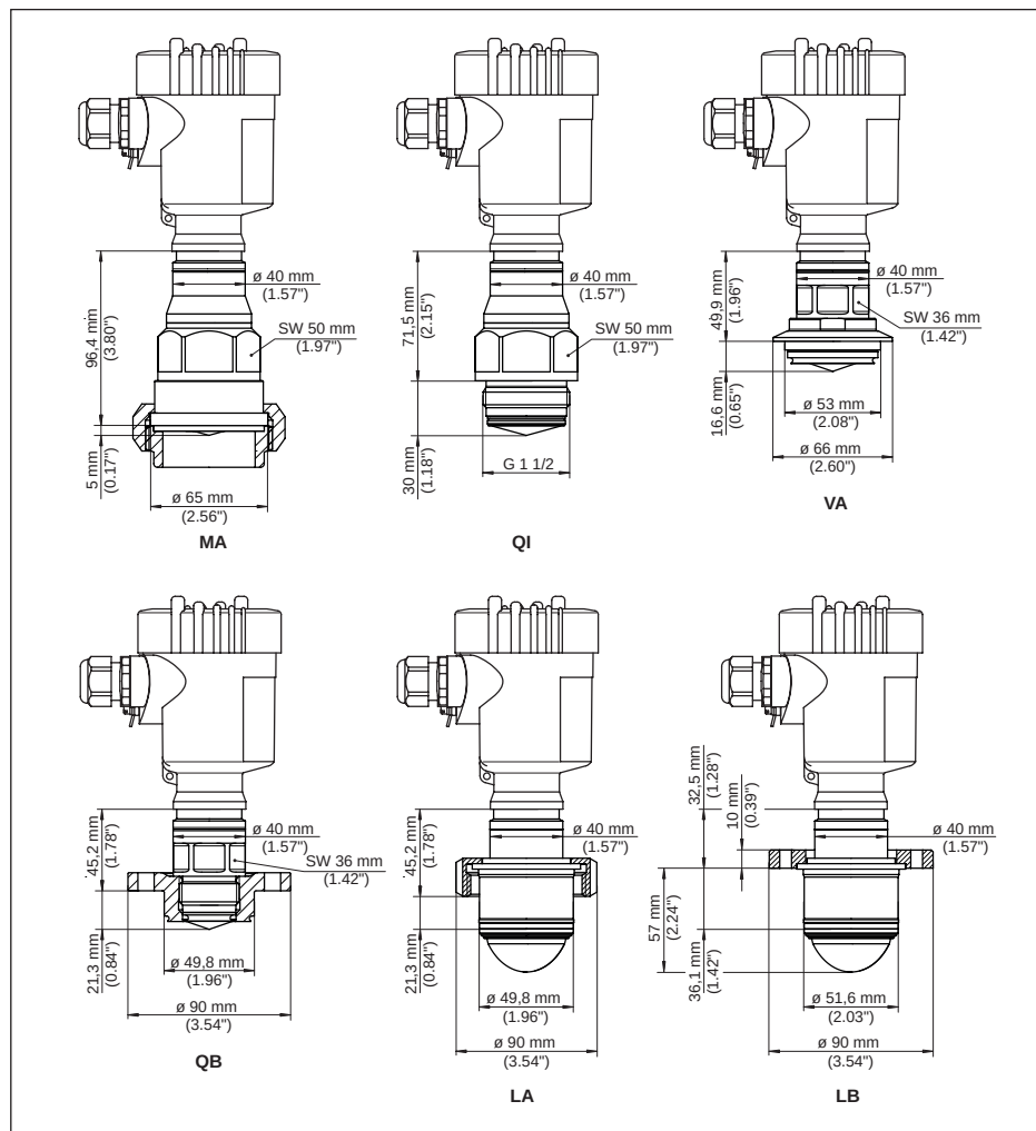
插图. 101: VEGAPULS 6X, 卫生型接口
