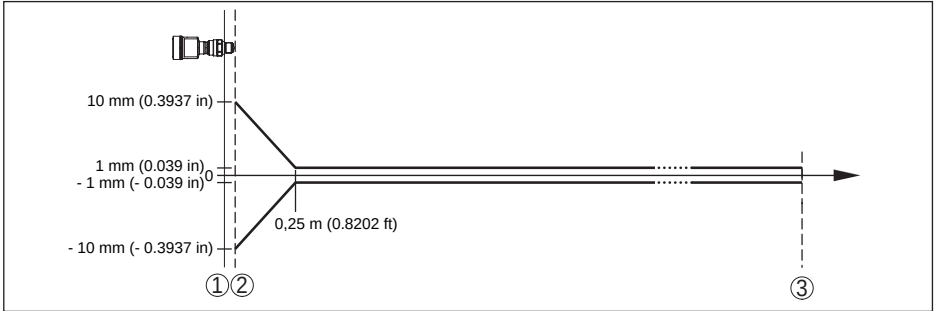
插图 69: 基准条件下的测量误差 (以带有内置天线系统的螺纹为例，相应地适用于所有版本)
