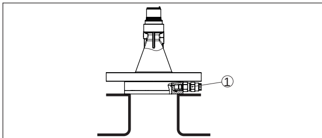
插图. 40: 塑料号角天线, 带锁紧法兰
