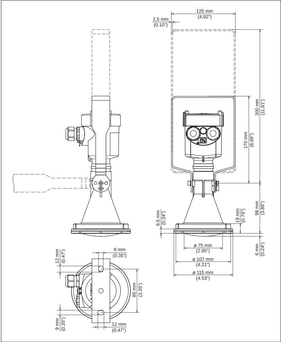
插图. 90: VEGAPULS 6X, 塑料号角天线，龙门框，长度为 170 或 300 mm
