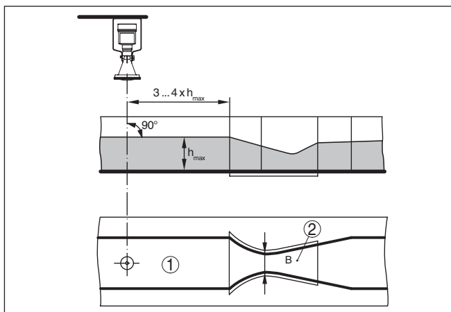
插图. 45: 用卡发基-文丘里槽来测量流量: h_{\max} = 水槽的最大灌装量; B = 水槽的最大收缩率
