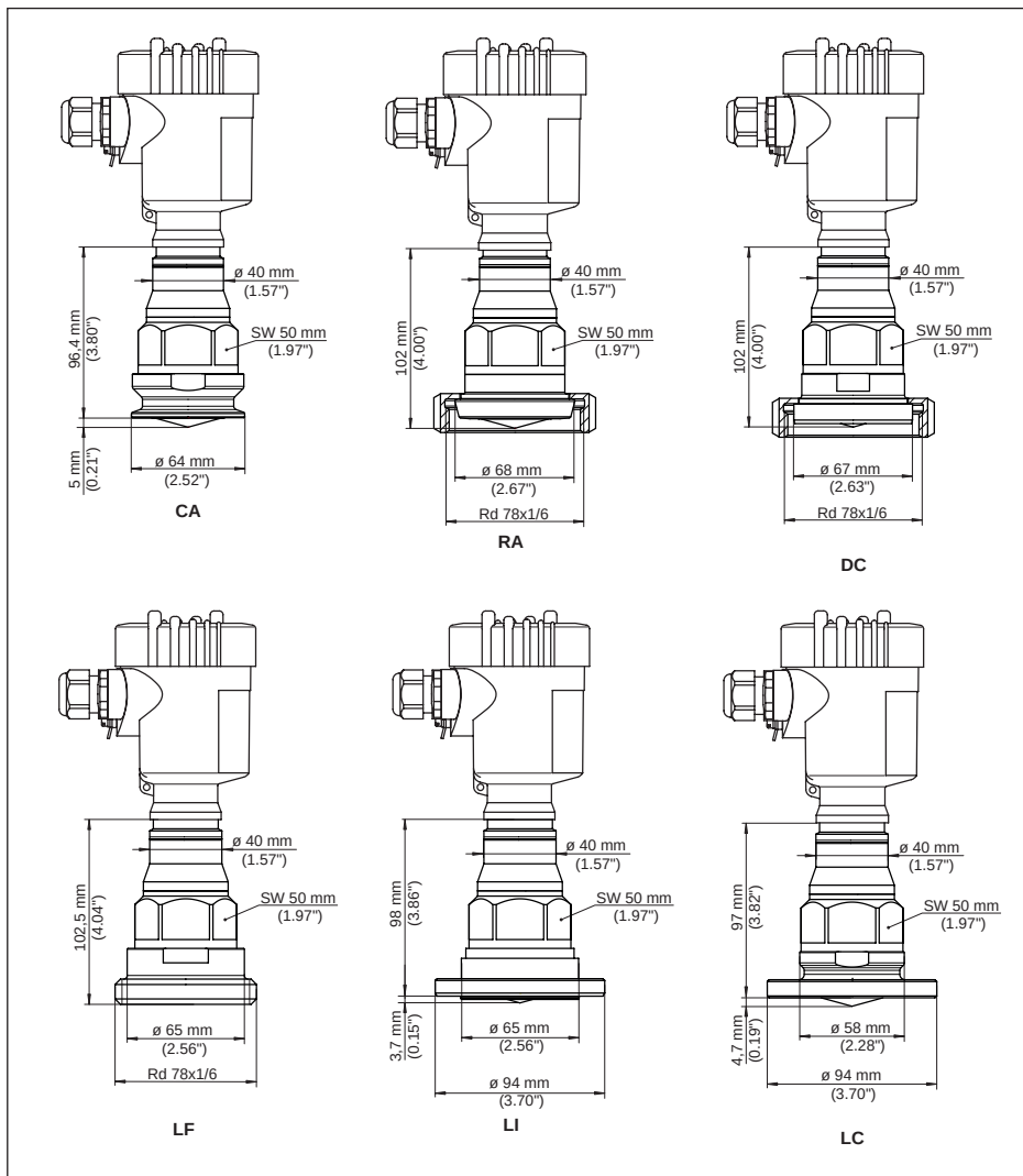
插图 100: VEGAPULS 6X, 卫生型接口
