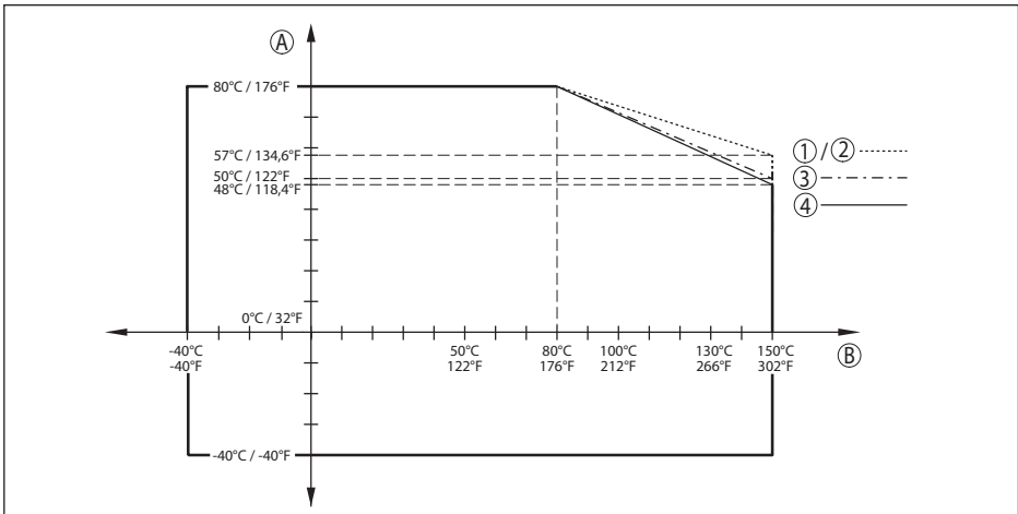
插图. 74: 环境温度的降额, 带有塑封天线的法兰, 卫生型接口至 +150 °C (+302 °F)
