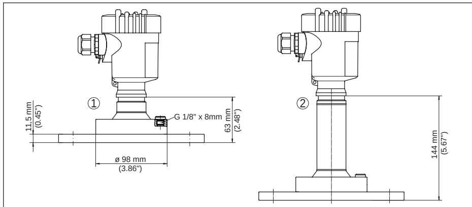
插图. 102: VEGAPULS 6X, 带有透镜天线的法兰 (法兰厚度参见图纸, 法兰尺寸根据 DIN, ASME, JIS)
