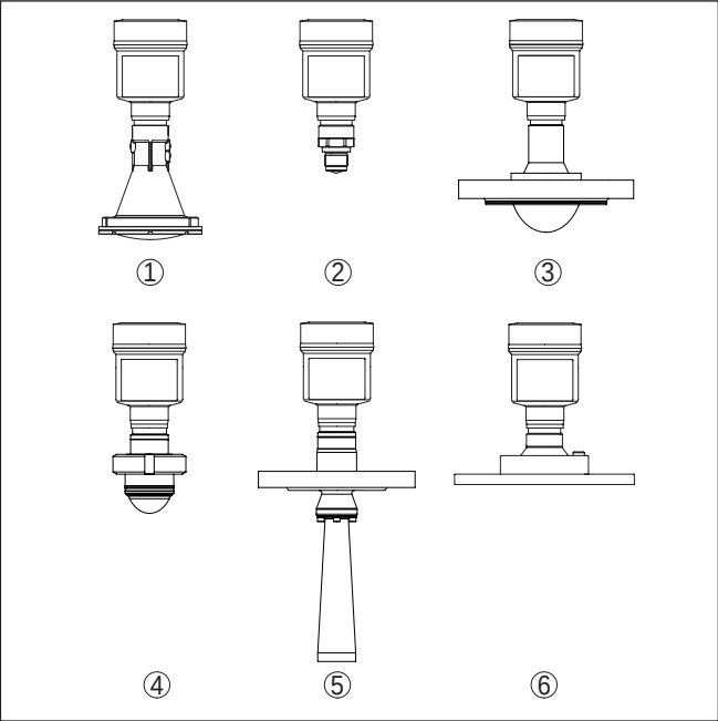
插图. 3: 天线系统 VEGAPULS 6X
