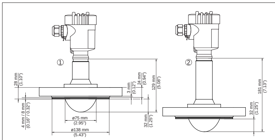
插图: 98: VEGAPULS 6X, 封装天线系统 DN 80 PN 40
