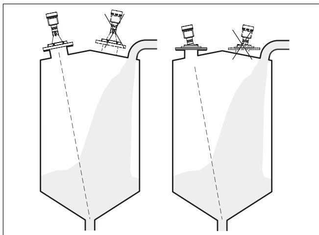
插图. 23: 当从上面充填介质时雷达传感器的安装
