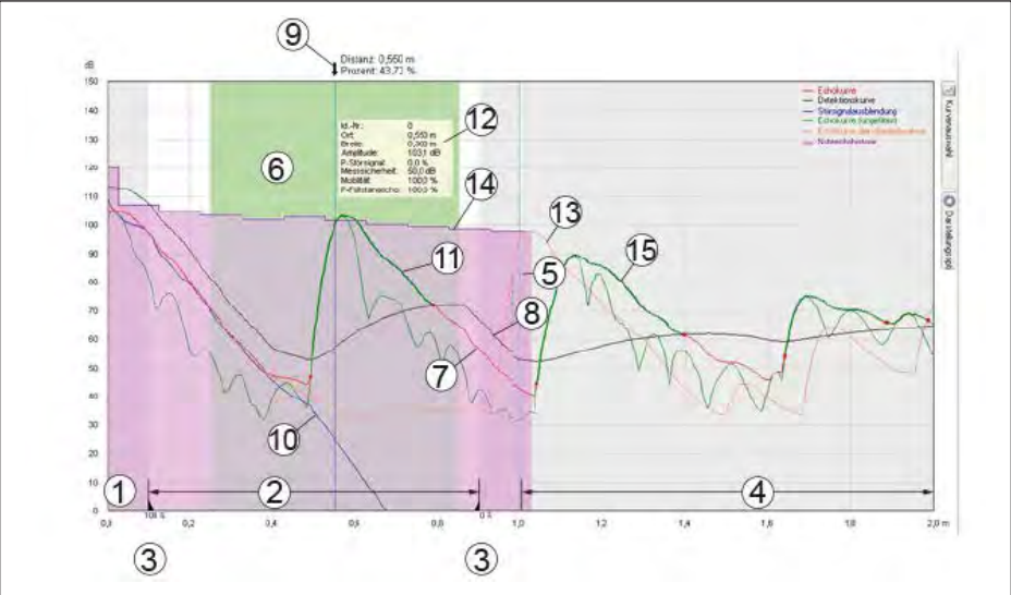
插图. 65: 回波曲线窗口内的范围
