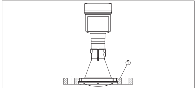
插图. 15: 组合式锁紧法兰
