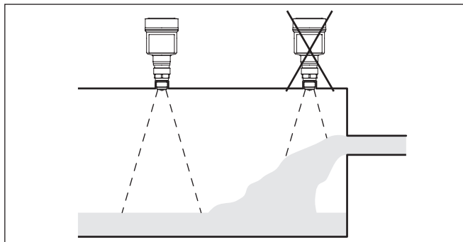
插图. 22: 流入介质时安装雷达传感器
