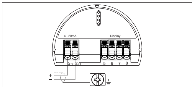
插图. 47: 单腔式外壳的电子部件和接线腔
