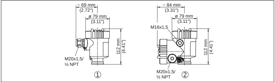
插图. 81: 采用防护等级为 IP66/IP67 的外壳版本 (内装显示和调整模块后，外壳高度增加了 9 mm/0.35 in)
