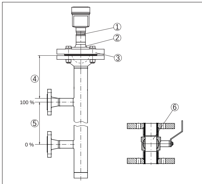
插图. 43: 旁路的构造
