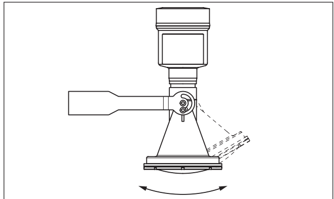
插图. 10: 水平安装在墙上时可以调节倾角
