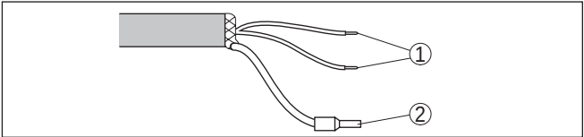
插图. 50: 固定连接的连接电缆的芯线分布
