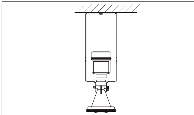
插图. 12: 用长度为 300 毫米的龙门框将仪表安装到天花板上
