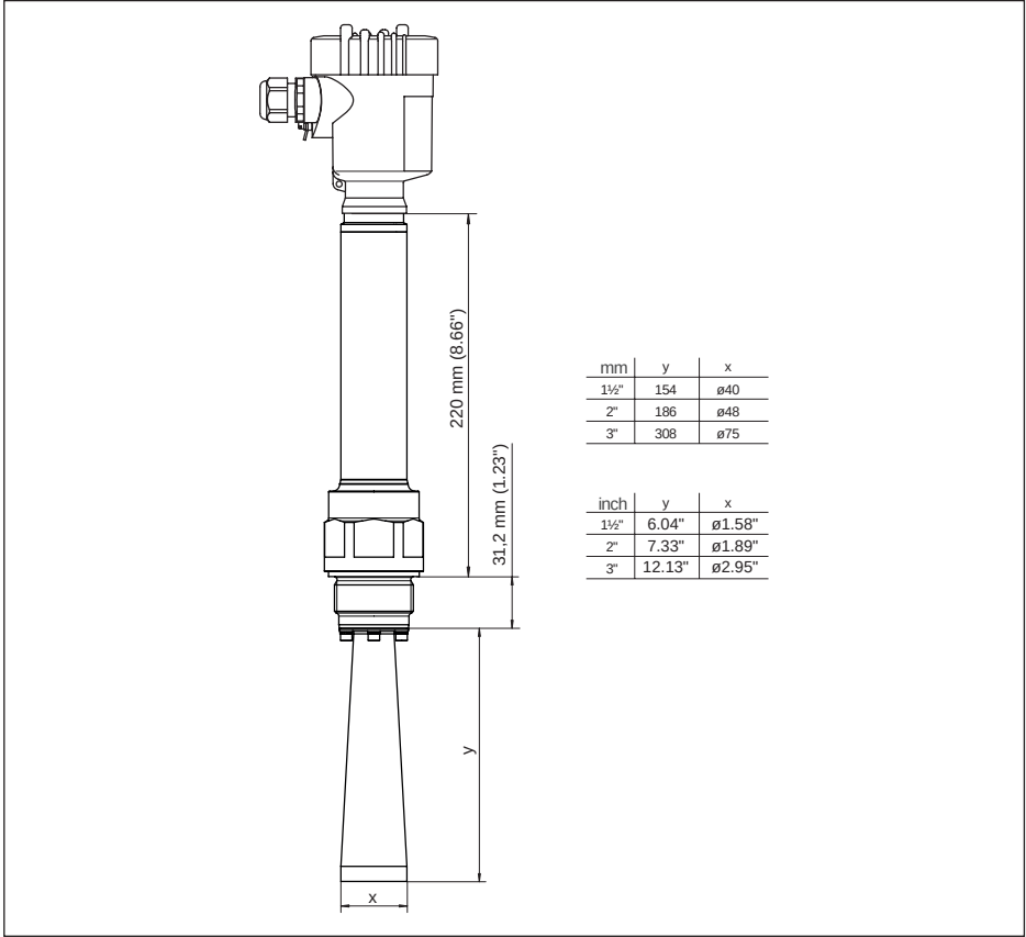
插图. 95: VEGAPULS 6X, 带有号角天线的螺纹, 450 °C 型
