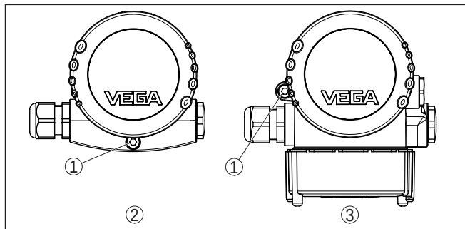
插图. 8: 防松螺钉的位置取决于外壳
