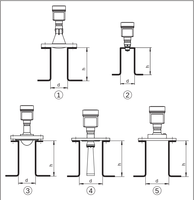
插图. 26: 在不同版本的 VEGAPULS 6X 上, 管接头尺寸有别时管接头的安装
