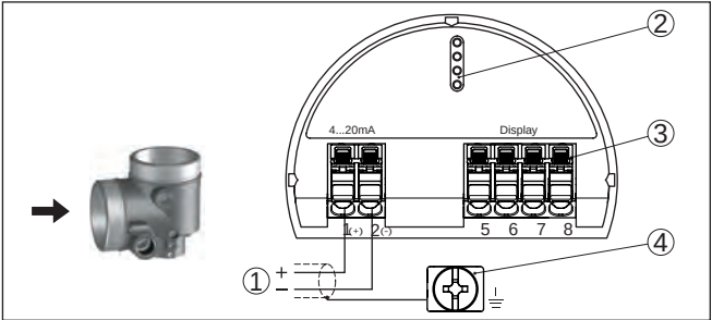
插图. 49: 双腔式外壳的接线腔
