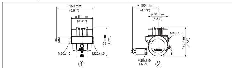
Fig. 90: Huisuitvoeringen in beschermingsklasse IP66/IP68 (1 bar), (met ingebouwde display- en bedieningsmodule wordt het huis 18 mm/0.71 in hoger)
