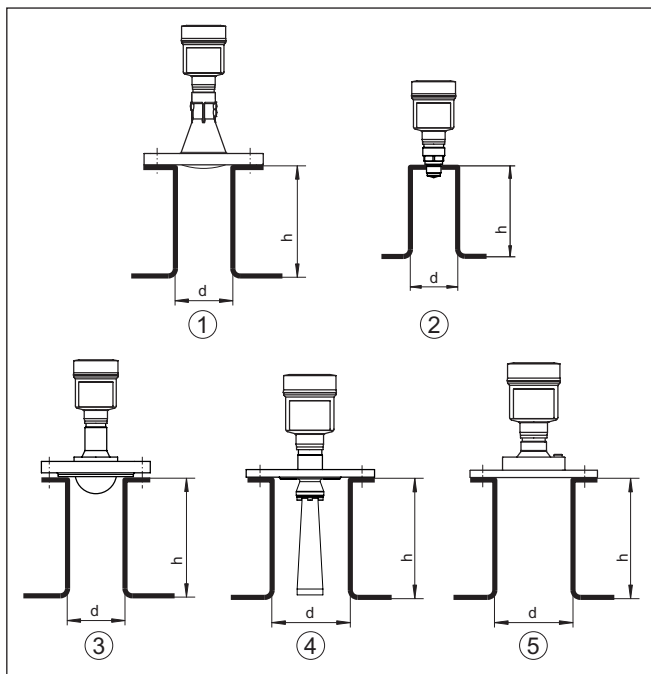
Fig. 26: Buissteunmontage bij afwijkende buissteunmaten bij verschillende uitvoeringen van de VEGAPULS 6X
