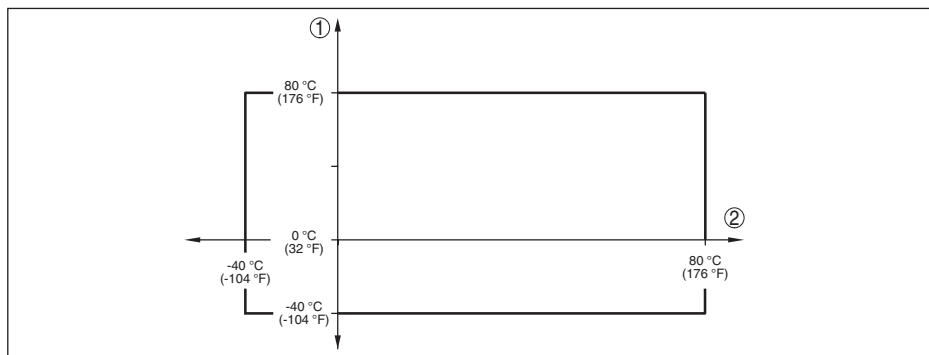
Fig. 71: Derating omgevingstemperatuur, kunststofhoornantenne
