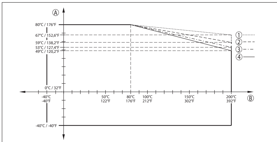
Fig. 73: Derating omgevingstemperatuur, schroefdraad met geïntegreerd antennesysteem tot +200 °C (+392 °F)
