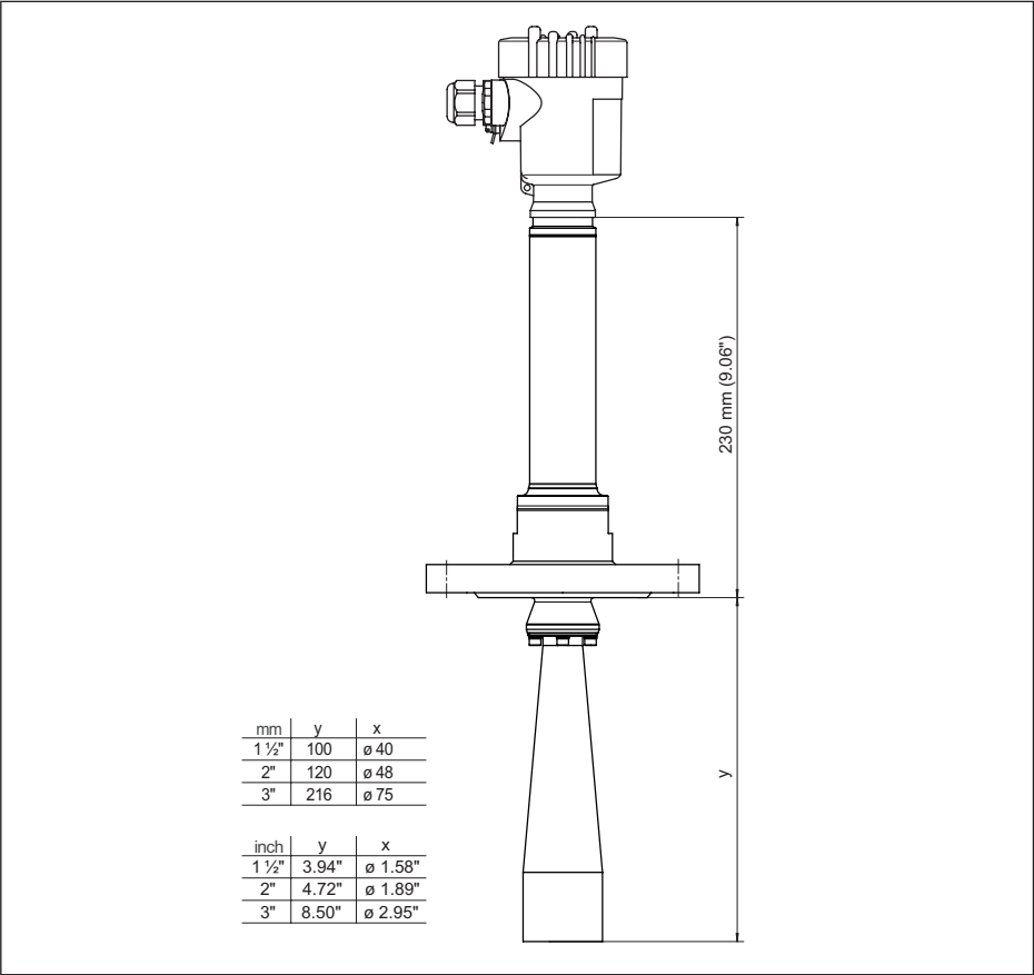
Fig. 101: VEGAPULS 6X, flens met hoornantenne 450 °C-uitvoering
