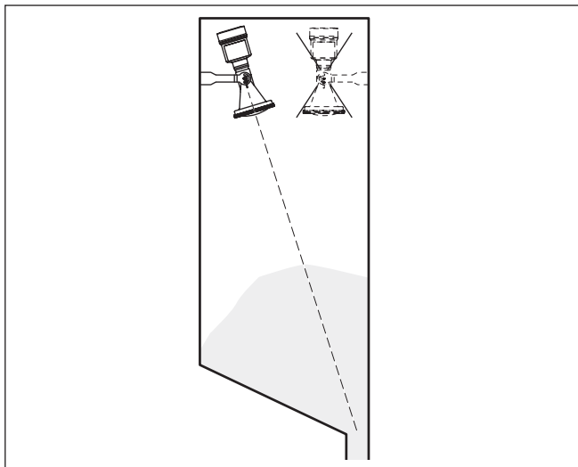
Fig. 39: Inbouw en uitrichting in meerkamersilo's
