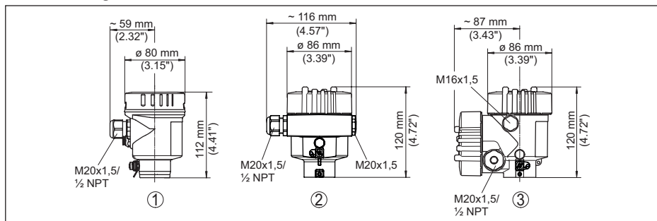
Fig. 89: Huisuitvoeringen in beschermingsklasse IP66/IP68 (0,2 bar), (met ingebouwde display- en bedieningsmodule wordt het huis 18 mm hoger)
