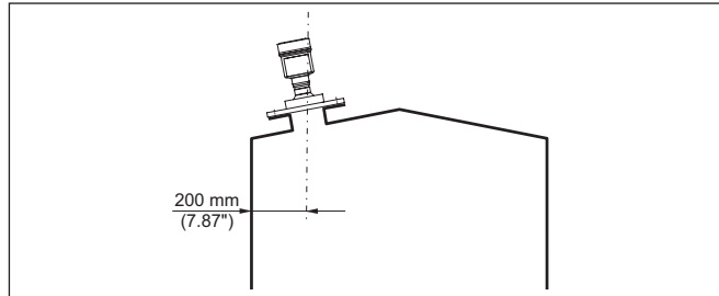
Fig. 20: Montage van de radarsensor op het tankdak
