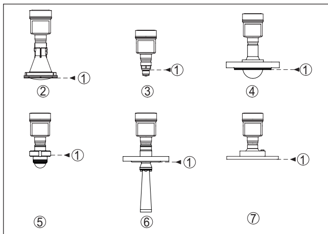
Fig. 21: Positie van het referentievlak
