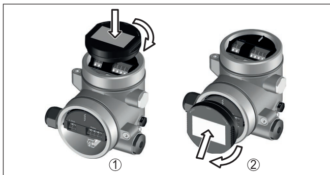
Fig. 52: Plaatsen van de display- en bedieningsmodule bij de tweekamerbehuizing
