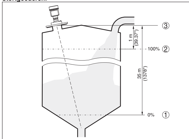
Fig. 56: Parametrevoorbeeld min.-/max.-inregeling - stortgoed
