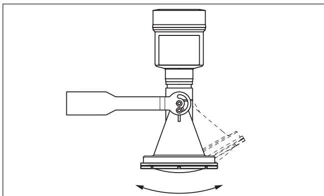
Fig. 10: Verstelling van de hoek bij horizontale montage aan de muur
