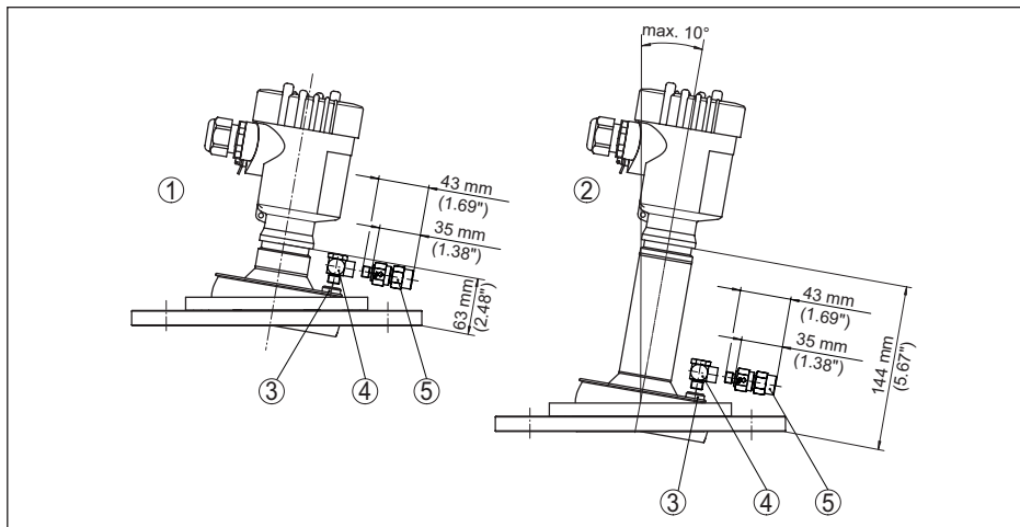
Fig. 110: VEGAPULS 6X, flens met lensantenne, zwenkhouter en spoelluchtaansluiting
