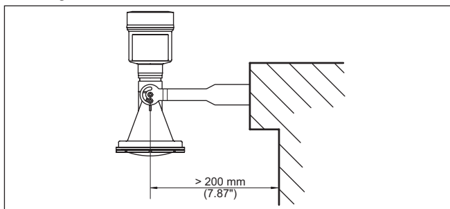
Fig. 13: Wandmontage horizontaal via de montagebeugel met lengte 170 mm
