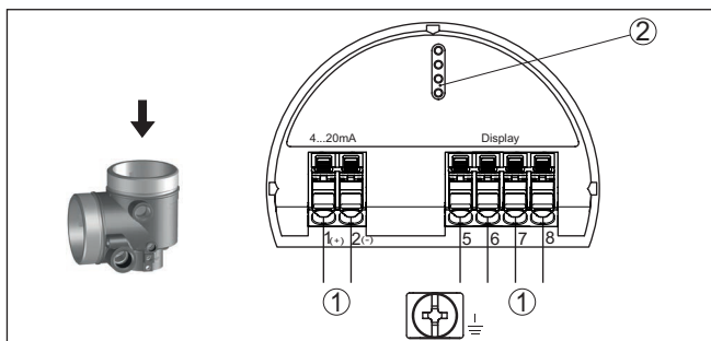
Fig. 48: Elektronicar ruimte - tweekamerbehuizing
