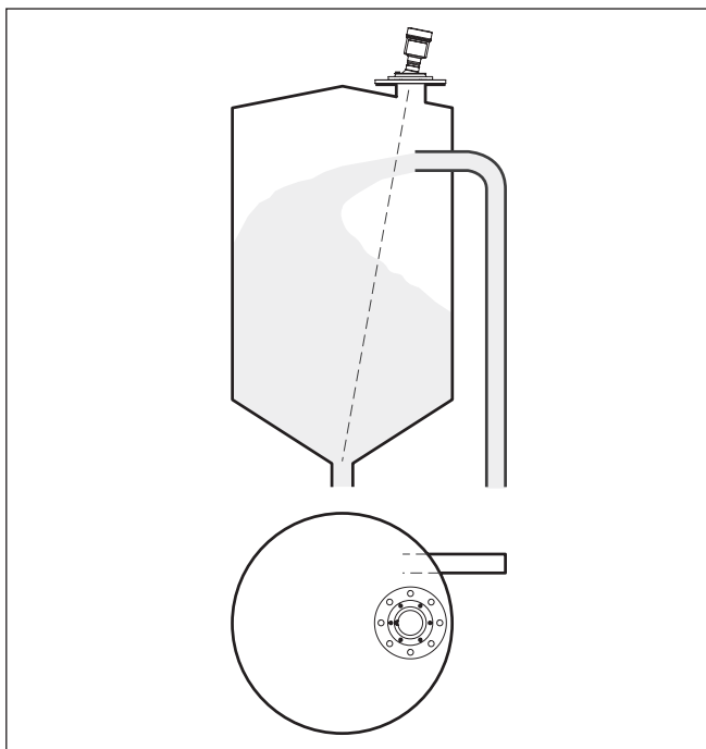
Fig. 24: Montage van de radarsensor bij instromend medium – vullen vanaf de zijkant
