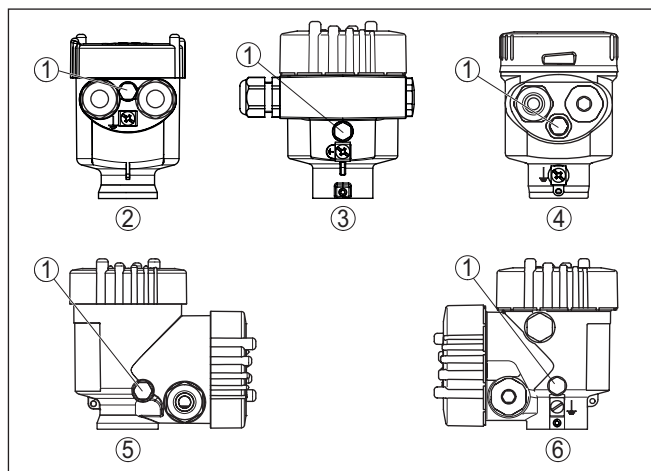
Fig. 6: Positie van het filterelement afhankelijk van de behuizing
