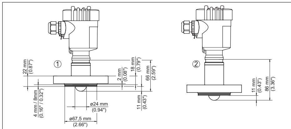
Fig. 102: VEGAPULS 6X, gekapseld antennesysteem DN 25 PN 40
