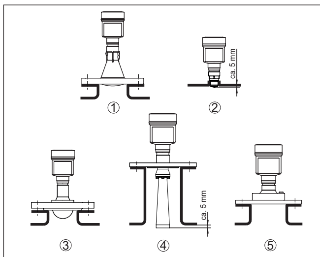
Fig. 25: Geadviseerde buissteunmontage bij verschillende uitvoeringen van de VEGAPULS 6X
