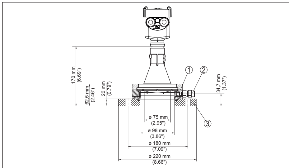
Fig. 94: VEGAPULS 6X, adapterflens en spoelluchtaansluiting DN 100 PN 6
