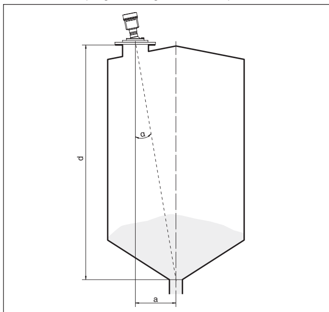
Fig. 34: Bepalen van de hellinghoek voor het uitlijnen van de VEGAPULS 6X
