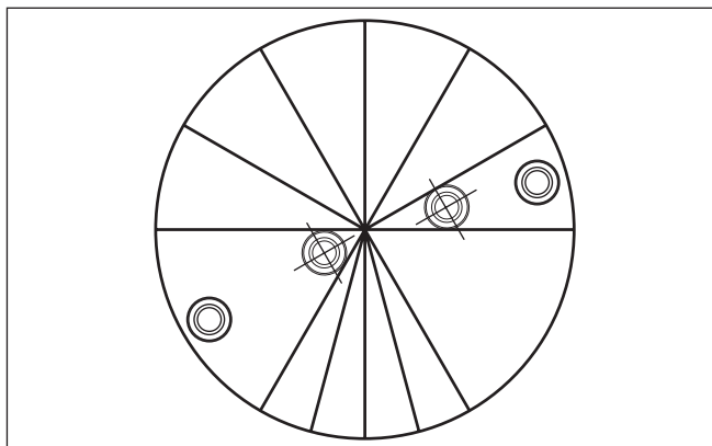
Fig. 38: Inbouw en uitrichting in meerkamersilo's
