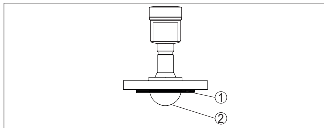
Fig. 27: VEGAPULS 6X met flens en gekapseld antennesysteem
