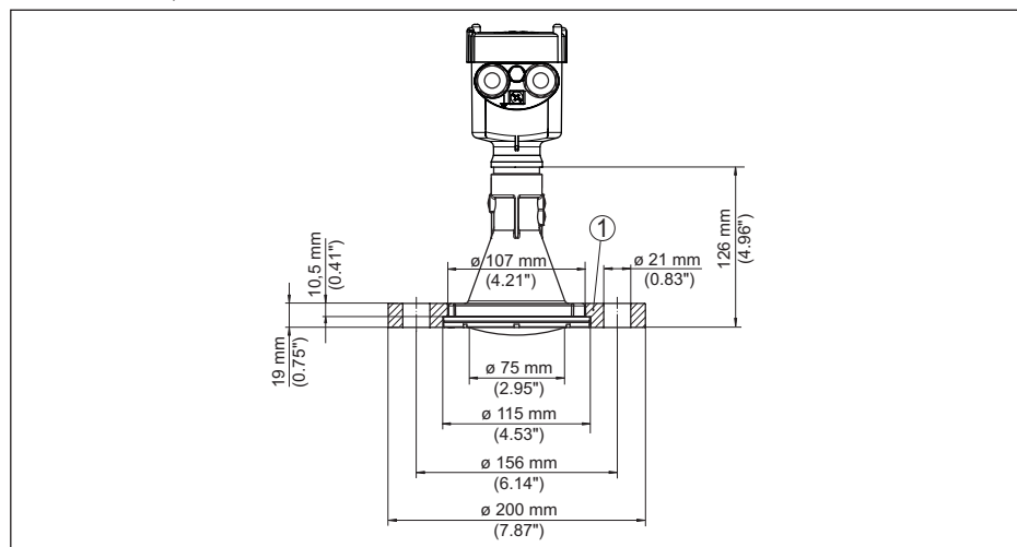
Fig. 91: VEGAPULS 6X met overschuifflens passend voor 3" 150 lbs, DN 80 PN 16
