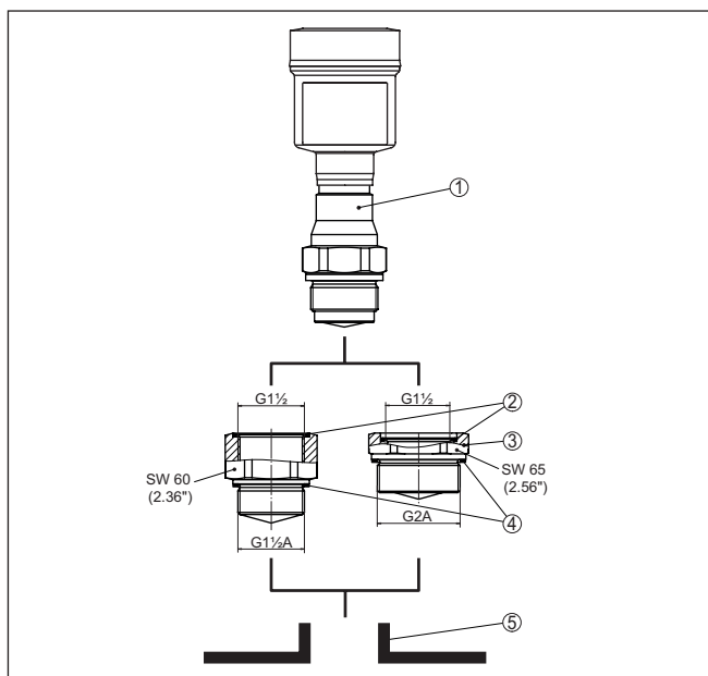
Fig. 29: VEGAPULS 6X met PTFE-schroefdraadadapter (voorbeeld VEGAPULS 6X met schroefdraad G1½)
