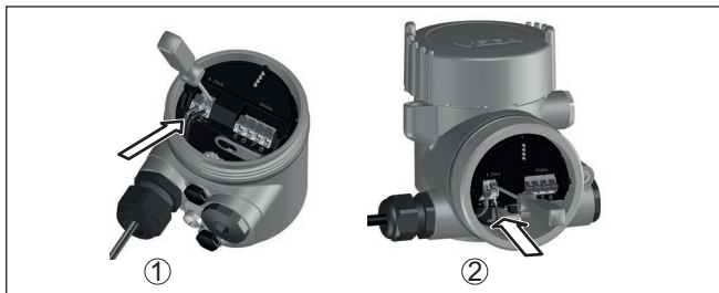
Fig. 46: Aansluitstappen 5 en 6
