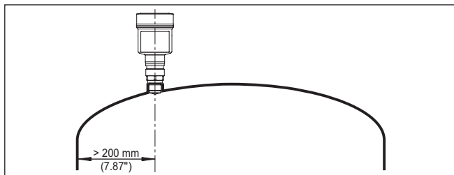
Fig. 18: Montage van de radarsensor op ronde tankdaken
