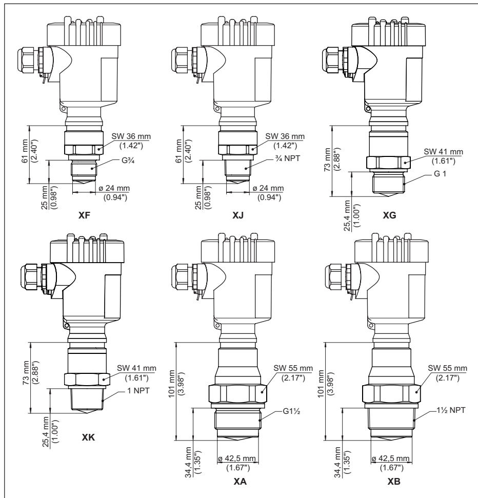
Fig. 97: VEGAPULS 6X, schroefdraad met geïntegreerd antennesysteem tot +150 °C (+302 °F)
