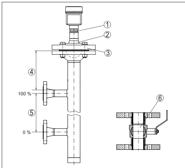
Fig. 43: Opbouw bypass
