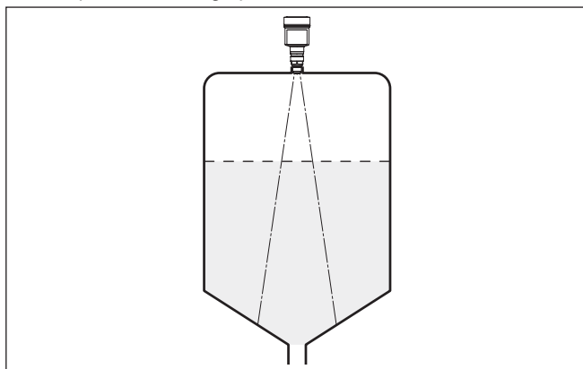
Fig. 19: Montage van de radarsensor op tanks met conische bodem
