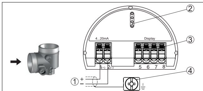
Fig. 49: Aansluitruimte - tweekamerbehuizing
