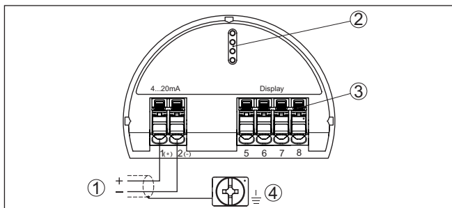
Fig. 47: Elektronica- en aansluitruimte - eenkamerbehuizing
