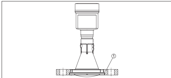
Fig. 15: Combi-overschuifflens
