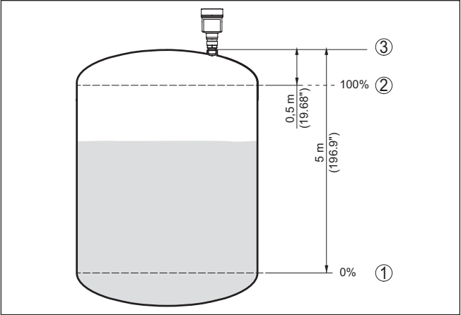
Fig. 55: Parametreervoorbeeld min.-/max.-inregeling - vloeistoffen
