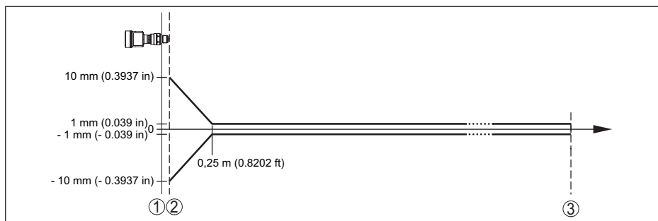
Fig. 70: Meetafwijking onder referentieomstandigheden (voorbeeld schroefdraad met geïntegreerd antennesysteem, geldt overeenkomstig voor alle uitvoeringen) 27)
