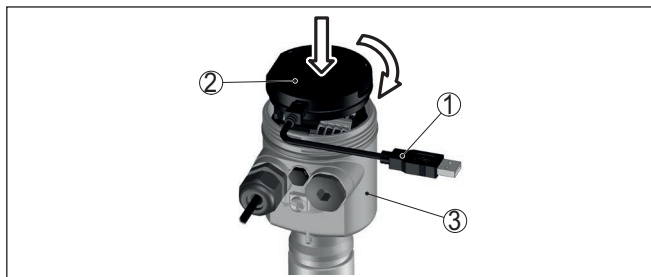
Fig. 62: Aansluiting van de PC via interface-adapter direct op de sensor
