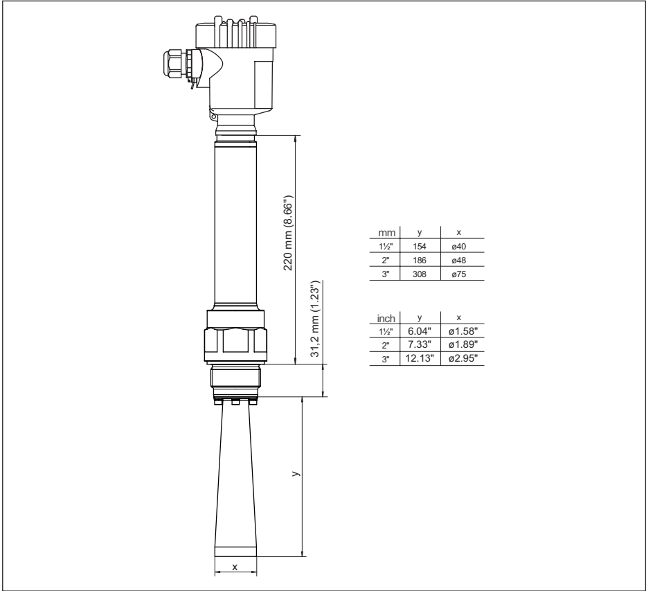
Fig. 100: VEGAPULS 6X, schroefdraad met hoornantenne 450 °C-uitvoering
