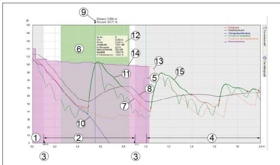
Fig. 66: Gebieden in het echocurvevenster
