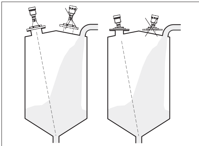
Fig. 23: Montage van de radarsensor bij instromend medium – vullen van bovenaf.
