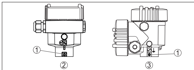
Fig. 7: Positie van de borgschroef afhankelijk van de behuizing
