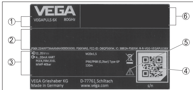
Fig. 2: Opbouw van de typeplaat (voorbeeld)
