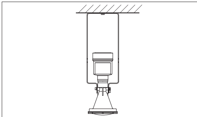
Fig. 12: Plafondmontage via de montagebeugel met lengte 300 mm
