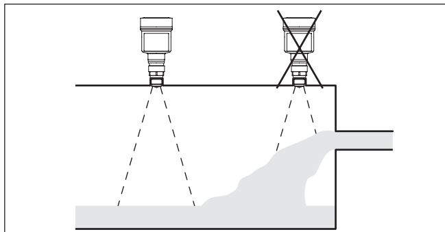
Fig. 22: Montage van de radarsensor bij instromend product
