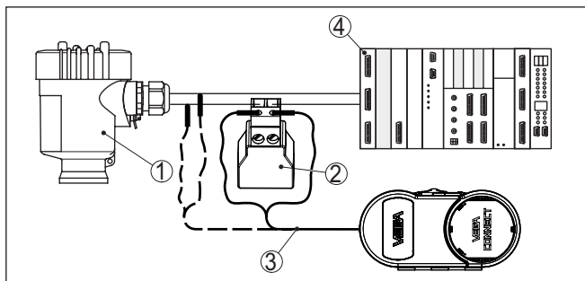
Fig. 63: Aansluiting van de PC via HART op de signaalkabel
