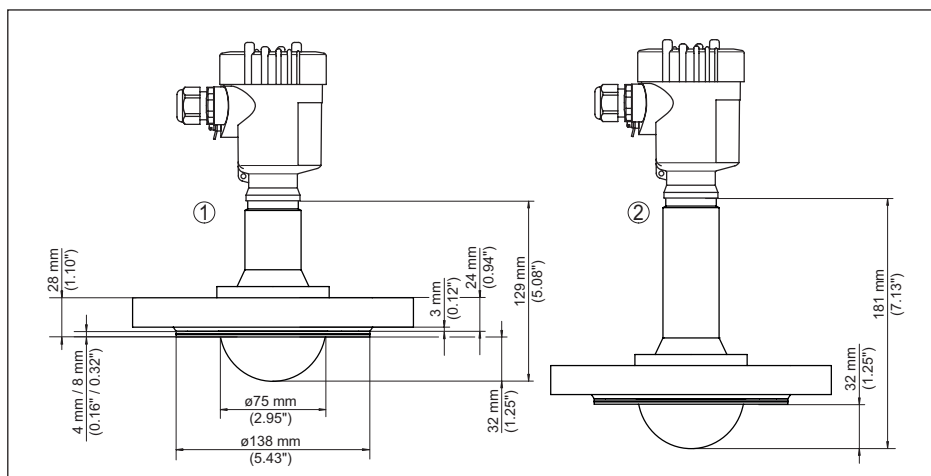
Fig. 103: VEGAPULS 6X, gekapseld antennesysteem DN 80 PN 40
