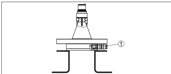
Fig. 40: Kunststofhoornantenne met overschuifflens
