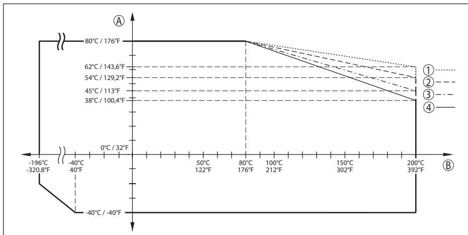
Fig. 78: Derating omgevingstemperatuur, flens met ingekapseld antennesysteem -196 ... +200 °C (-320,8 ... +392 °F)
