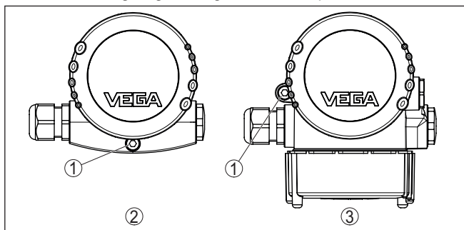
Fig. 8: Positie van de borgschroef afhankelijk van de behuizing
