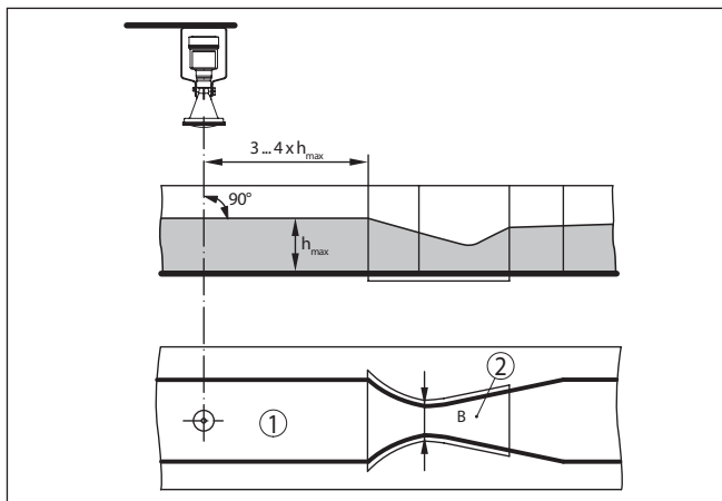
Fig. 45: Flowmeting met Khafagi-venturigoot: h_{max} = max. peil in de goot; B = maximale insnoering van de goot
