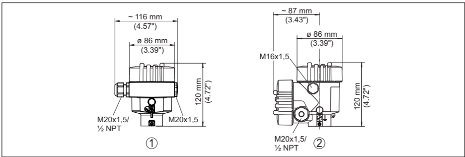
Fig. 87: Huisuitvoeringen in beschermingsklasse IP66/IP68 (0,2 bar), (met ingebouwde display- en bedieningsmodule wordt het huis 18 mm hoger)
