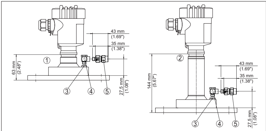
Fig. 108: VEGAPULS 6X, flens met lensantenne en spoelluchtaansluiting
