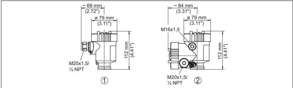
Fig. 86: Huisuitvoeringen in beschermingsklasse IP66/IP67 (met ingebouwde aanwijs- en bedieningsmodule wordt het huis 9 mm hoger)
