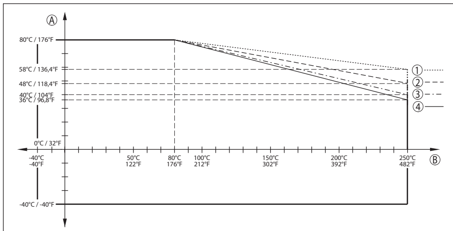
Fig. 74: Derating omgevingstemperatuur, schroefdraad met geïntegreerd antennesysteem tot +250 °C (+482 °F)
