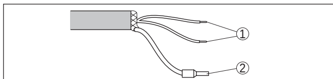
Fig. 50: Aderbezetting vast aangesloten aansluitkabel
