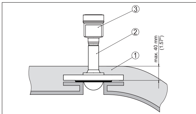
Fig. 30: Montage van het instrument in geïsoleerde tanks
