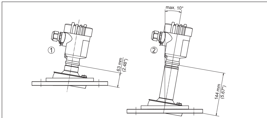
Fig. 109: VEGAPULS 6X, flens met lensantenne en zwenkhouter
