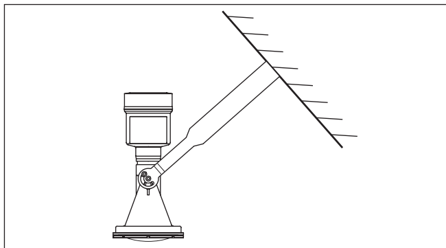
Fig. 14: Wandmontage met schuine wand met de montagebeugel met lengte 300 mm
