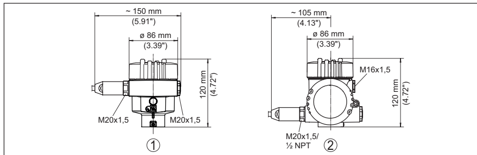
Fig. 88: Huisuitvoeringen in beschermingsklasse IP66/IP68 (1 bar), (met ingebouwde display- en bedieningsmodule wordt het huis 86 mm/0.71 in hoger)
