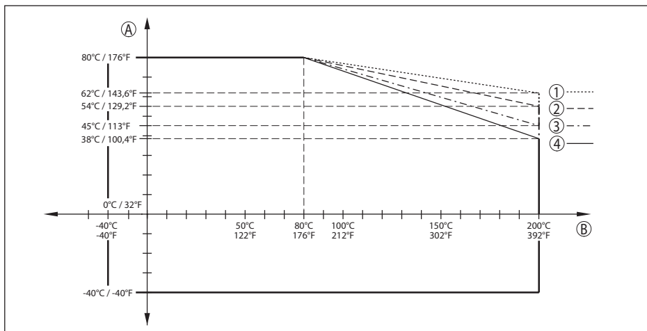
Fig. 77: Derating omgevingstemperatuur, flens met ingekapseld antennesysteem tot +200 °C (+392 °F)
