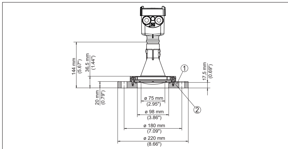
Fig. 93: VEGAPULS 6X met adapterflens DN 100 PN 6
