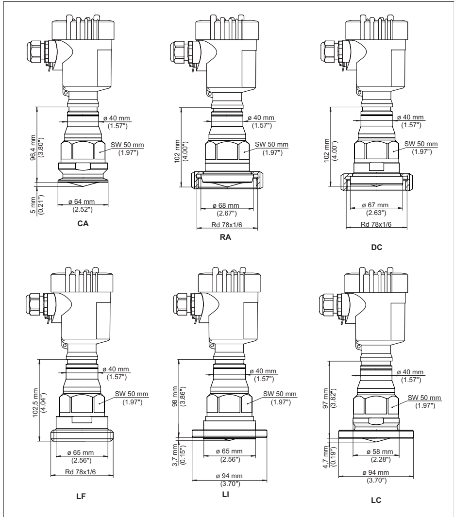
Fig. 105: VEGAPULS 6X, aseptische aansluiting
