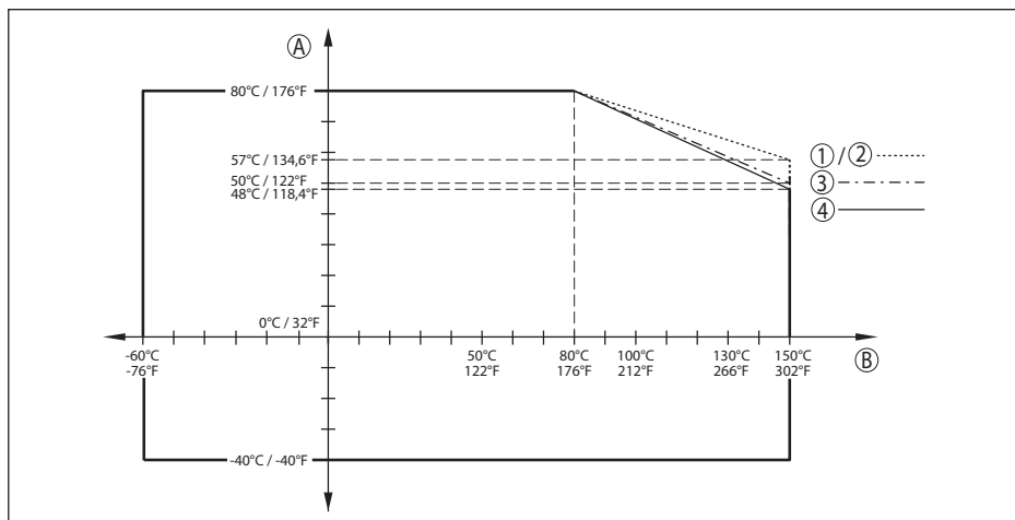
Fig. 76: Derating omgevingstemperatuur, flens met ingekapseld antennesysteem -60 ... +150 °C (-76 ... +302 °F)
