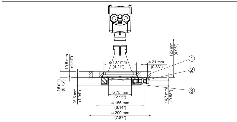
Fig. 92: VEGAPULS 6X met overschuifflens en spoelluchtaansluiting passend voor 3" 150 lbs, DN 80 PN 16
