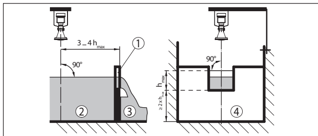
Fig. 44: Flowmeting met rechthoekig overstortschot: h_{max} = max. vulling van het rechthoekig overstortschot
