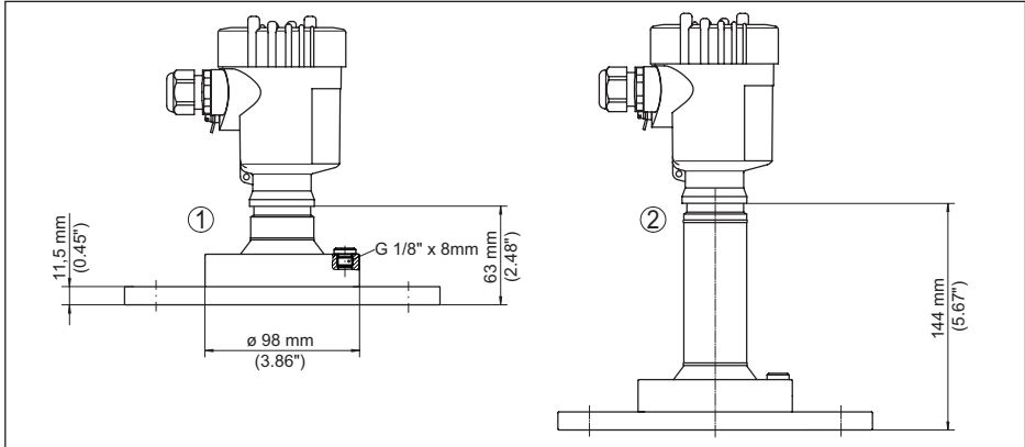
Fig. 107: VEGAPULS 6X, Flens met lensantenne (flensdikte zie tekening, flensmaten conform DIN, ASME, JIS)
