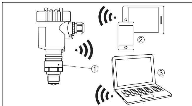
Fig. 4: Draadloze verbinding met standaard bedieningsapparaten met geïntegreerde Bluetooth LE
