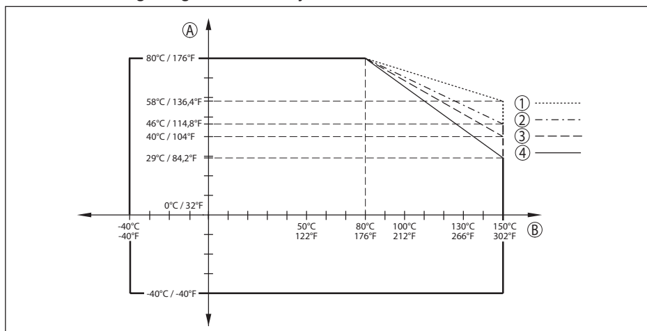
Fig. 72: Derating omgevingstemperatuur, schroefdraad met geïntegreerd antennesysteem tot +150 °C (+302 °F)
