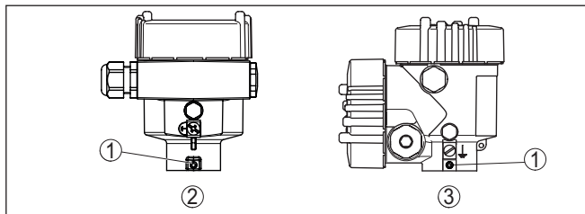
插图. 6: 止动螺钉的位置取决于壳体
