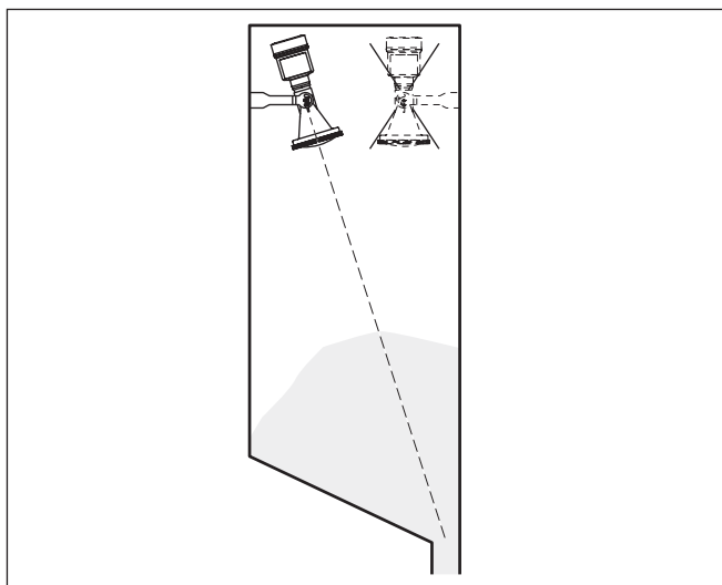
插图. 38: 在多腔式料仓中进行安装和校准
