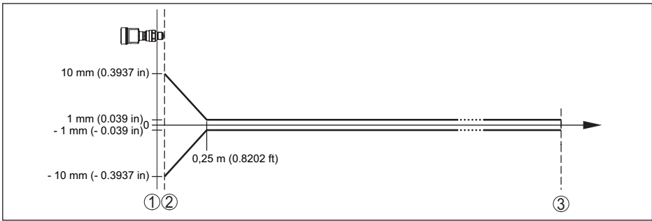
插图. 66: 基准条件下的测量误差 (以带有内置天线系统的螺纹为例, 相应地适用于所有版本) 27)
