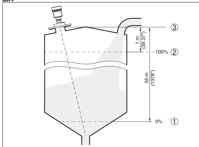
插图. 52: 参数调整举例：最小/最大调整 - 固料
