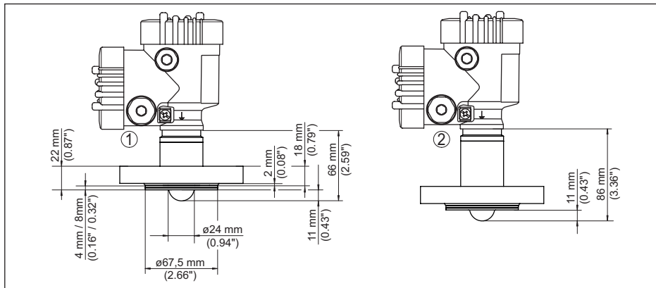
插图 94: VEGAPULS 6X, 封装天线系统 DN 25 PN 40
