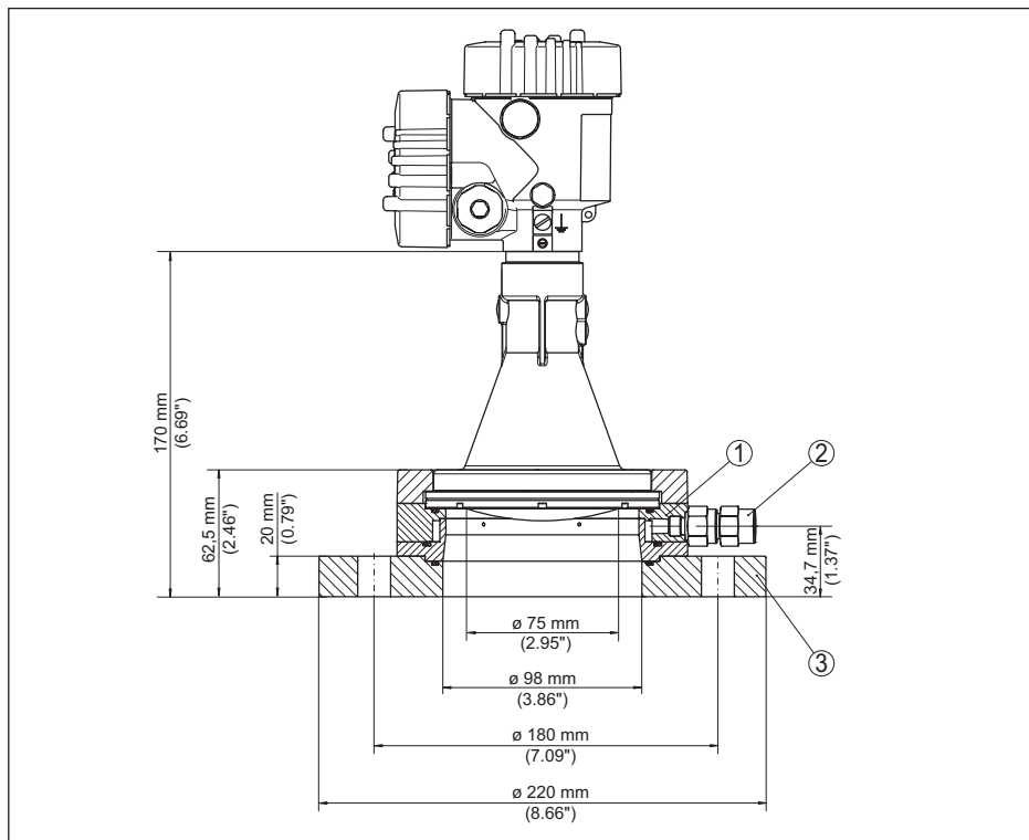
插图. 86: VEGAPULS 6X, 适配法兰和吹气接口 DN 100 PN 6
