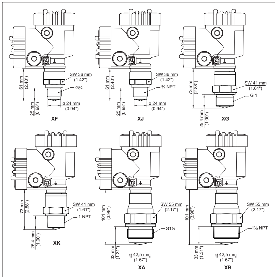
插图. 89: VEGAPULS 6X, 带有内置天线系统的螺纹, 至 +150 °C (+302 °F)
