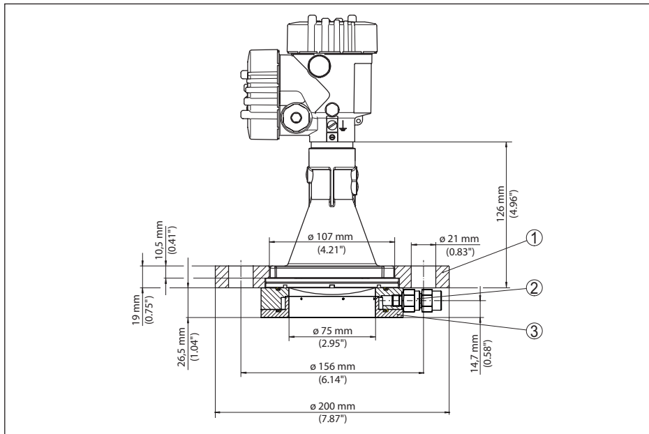
插图. 84: VEGAPULS 6X, 带有锁紧法兰和吹气接口, 适用于 3" 150 lbs, DN 80 PN 16
