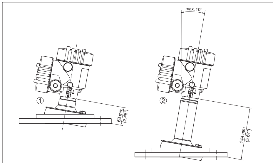
插图. 101: VEGAPULS 6X, 带有透镜天线和万向节的法兰
