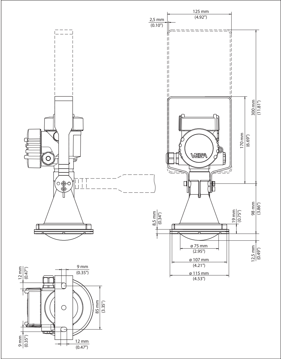
插图. 87: VEGAPULS 6X, 塑料号角天线, 龙门框, 长度为 170 或 300 mm
