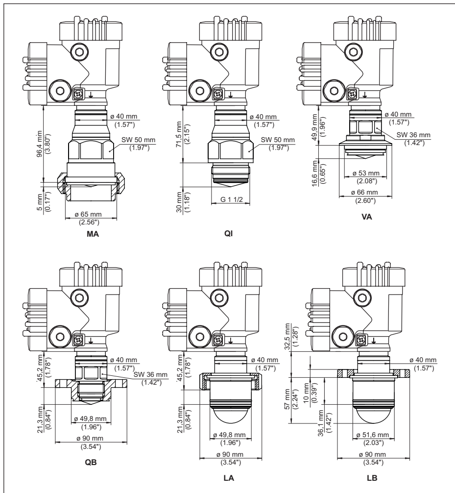
插图 98: VEGAPULS 6X, 卫生型接口
