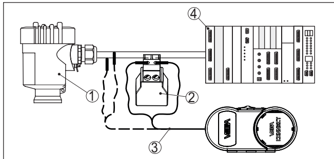
插图. 59: 通过 HART 将电脑与信号线路相连
