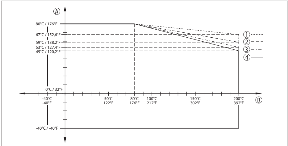
插图. 80: 环境温度降额, 带喇叭口天线的法兰, 至 +200 °C (+392 °F)
