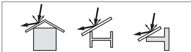
插图. 30: 用散射挡板来覆盖光滑的型材
