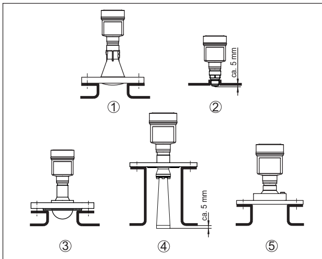
插图. 24: 对于不同版本的 VEGAPULS 6X 的安装管接头的推荐参数
