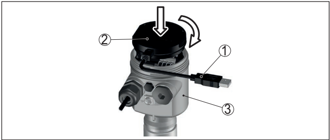
插图. 58: 通过接口适配器将电脑直接与传感器相连
