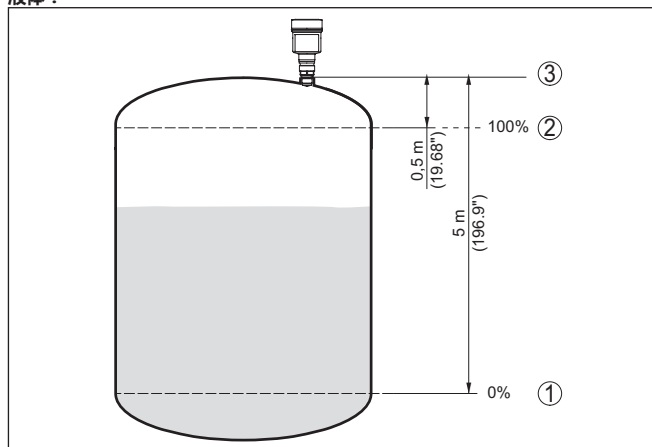
插图. 51: 参数调整举例：最小/最大调整 - 液体
