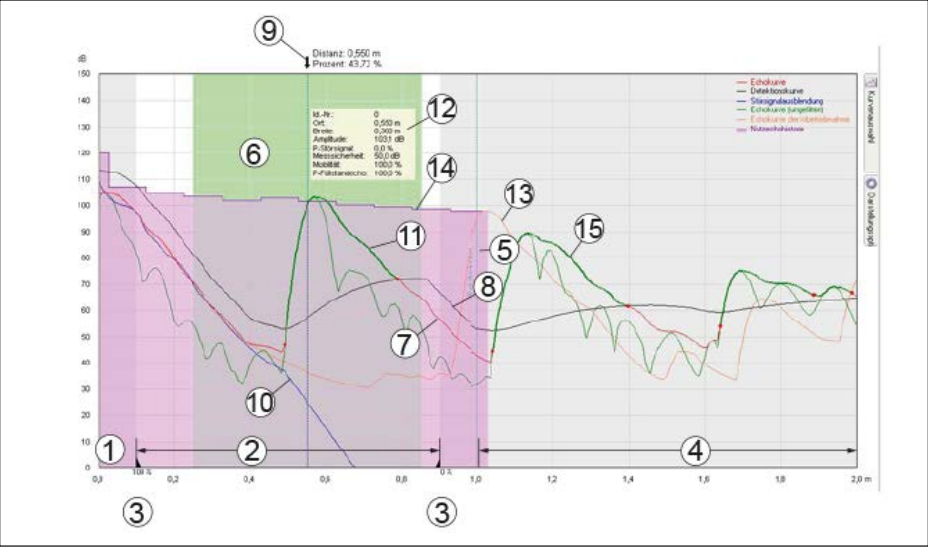
插图. 62: 回波曲线窗口内的范围 1 传感器基准面 (0 m)/扩展了的显示范围 2 测量范围 3 调整范围 4 测量范围终端的安全范围 5 容器高度 6 聚焦范围 7 回波曲线 8 检测曲线 9 距离和百分比值箭头 10 干扰信号抑制 11 检测出的回波连同起点和终点 12 所选回波的回波参数 13 调试时获得的回波曲线 14 有效回波的历史记录 15 回波曲线未经过滤
