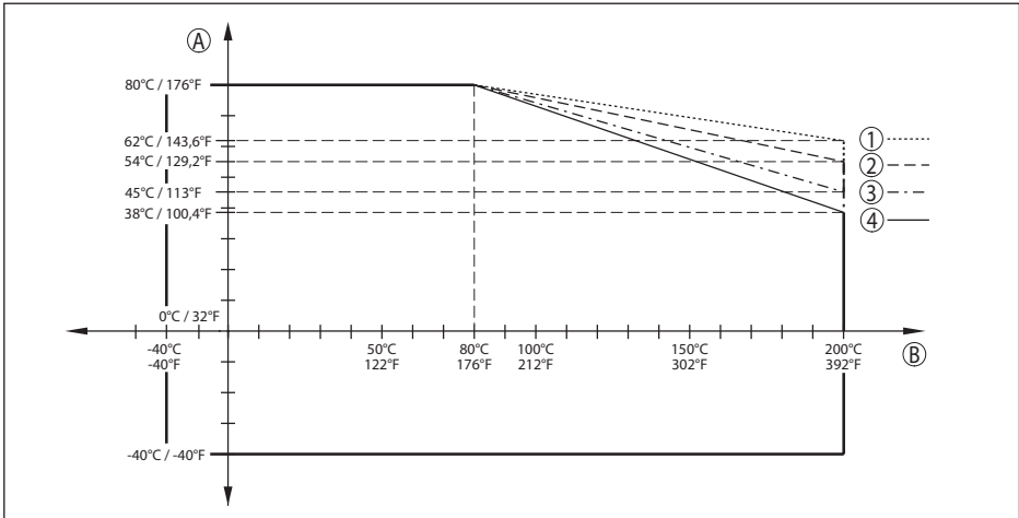
插图. 73: 环境温度降额, 带塑料天线系统的法兰, 至 +200 °C (+392 °F)
