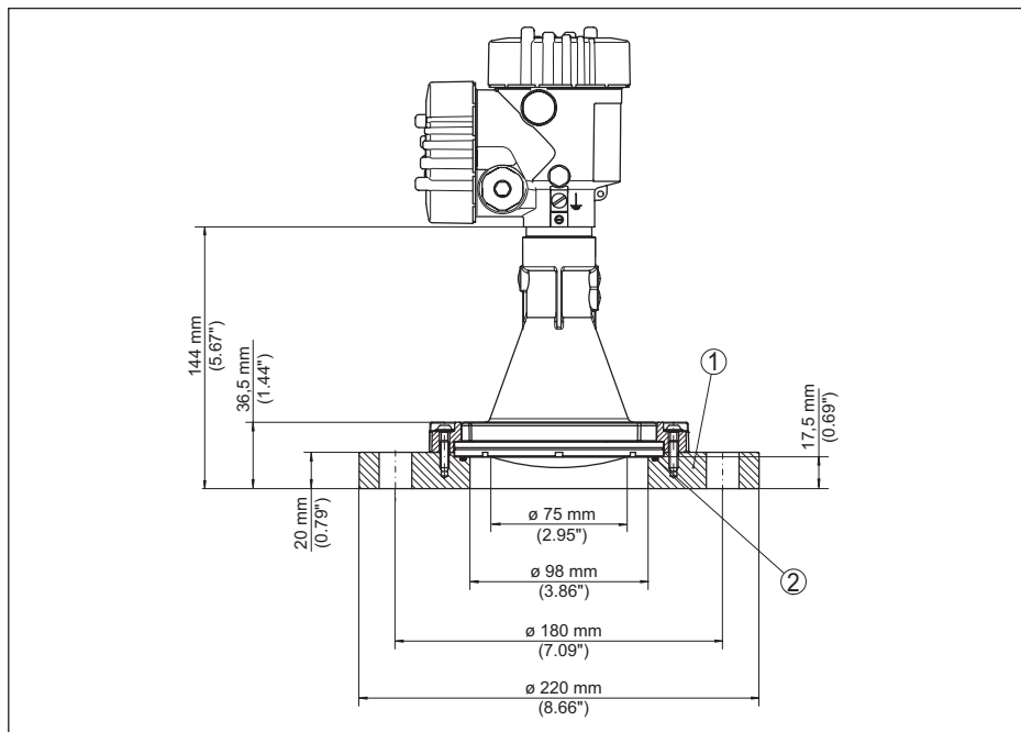
插图. 85: VEGAPULS 6X, 带适配法兰 DN 100 PN 6
