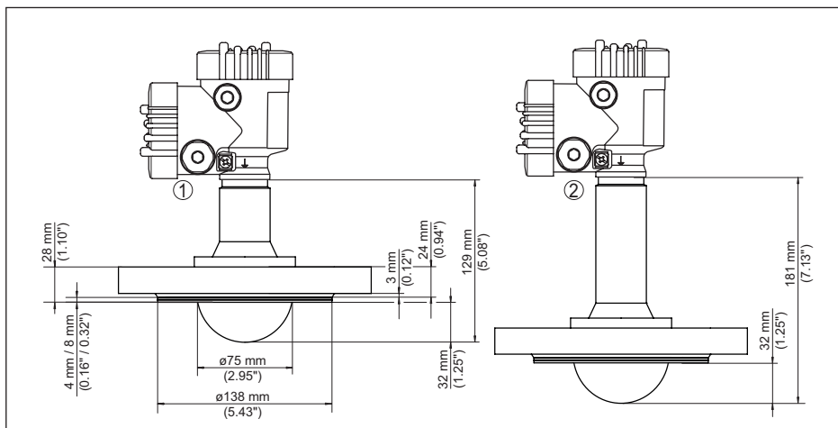
插图 95: VEGAPULS 6X, 封装天线系统 DN 80 PN 40
