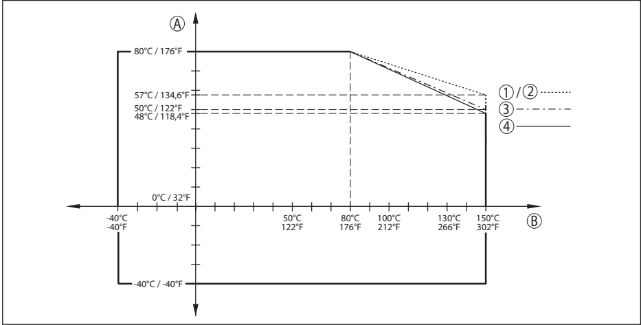
插图. 71: 环境温度降额，带塑封天线系统的法兰，至 +150 °C (+302 °F)
