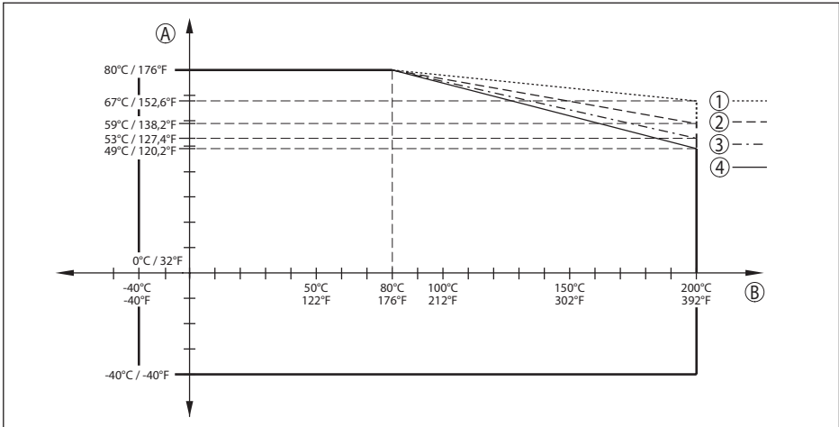
插图. 69: 环境温度降额, 带内置天线系统的螺纹, 至 +200 °C (+392 °F)
