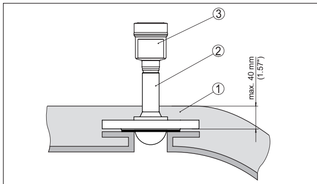
插图. 29: 将仪表安装在绝缘容器上
