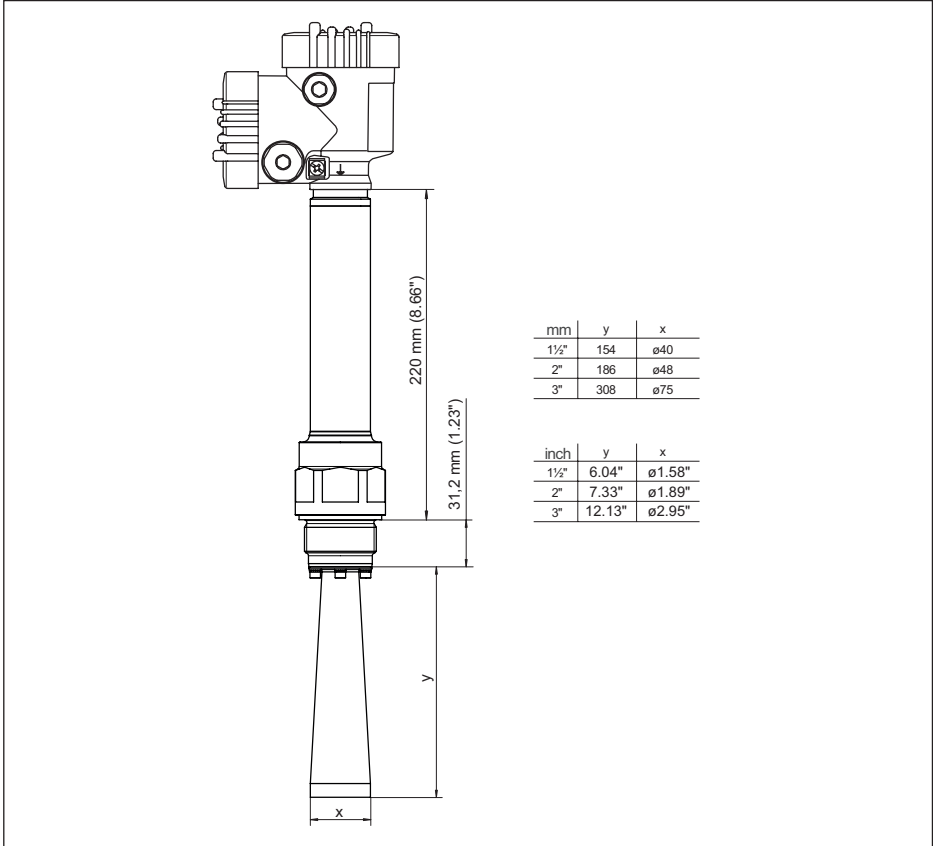
插图. 92: VEGAPULS 6X, 带有号角天线的螺纹, 450 °C 型
