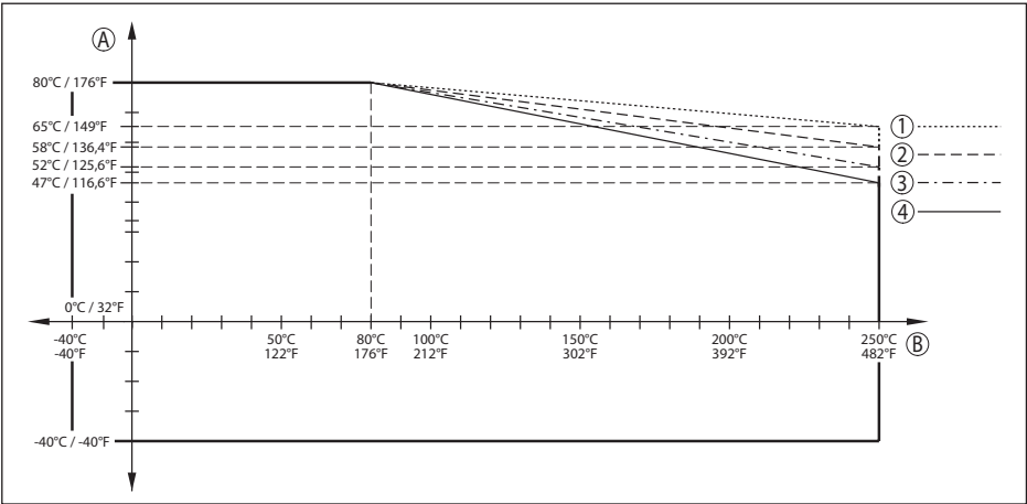
插图. 77: 环境温度降额, 带透镜天线的法兰, 至 +250 °C (+482 °F)
