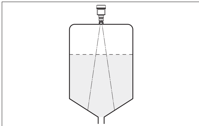
插图. 18: 将雷达传感器安装到带有锥形底部的容器上
