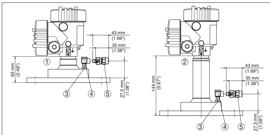
插图. 100: VEGAPULS 6X, 带有透镜天线和吹气接口的法兰
