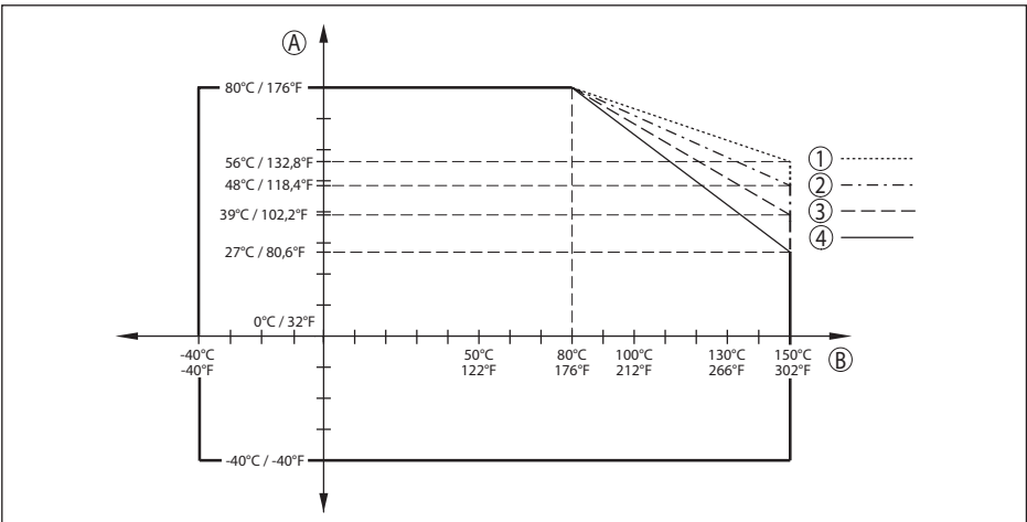
插图. 78: Derating Umgebungstemperatur, Hygieneanschluss bis +150 °C (+302 °F)
