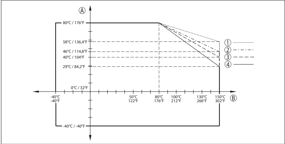
插图. 79: 环境温度降额, 带喇叭口天线的法兰, 至 +150 °C (+302 °F)
