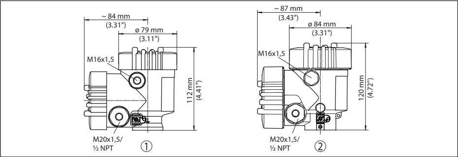
插图. 82: 采用防护等级达 IP66/IP67 和 IP66/IP68 (0.2 bar) 的壳体时，(内装显示和调整模块后，壳体高度将增加 9 mm/0.35 in 或 18 mm/0.71 in)
