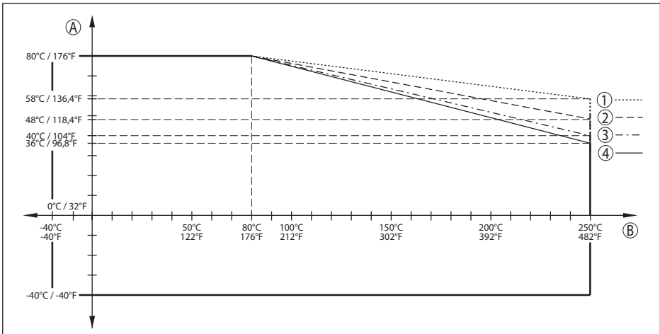
插图. 70: 环境温度降额, 带内置天线系统的螺纹, 至 +250 °C (+482 °F)
