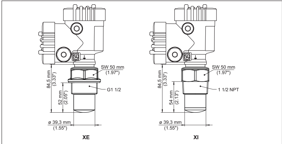
插图. 88: VEGAPULS 6X, 带有内置天线系统的螺纹, 至 +80 °C (+176 °F)
