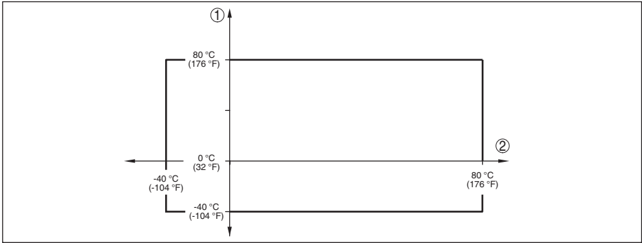
插图. 67: 环境温度降额，塑料号角天线
