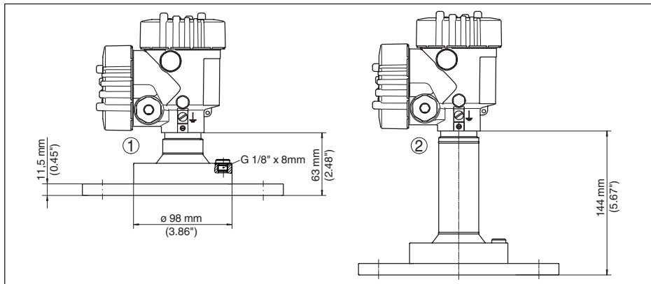
插图. 99: VEGAPULS 6X, 带有透镜天线的法兰 (法兰厚度参见图纸, 法兰尺寸根据 DIN, ASME, JIS)
