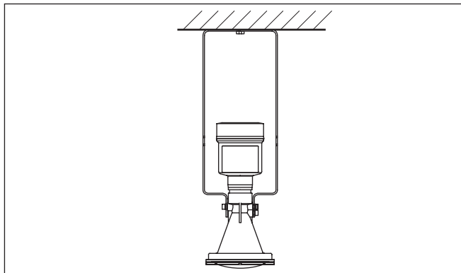
插图. 11: 用长度为 300 毫米的龙门框将仪表安装到天花板上
