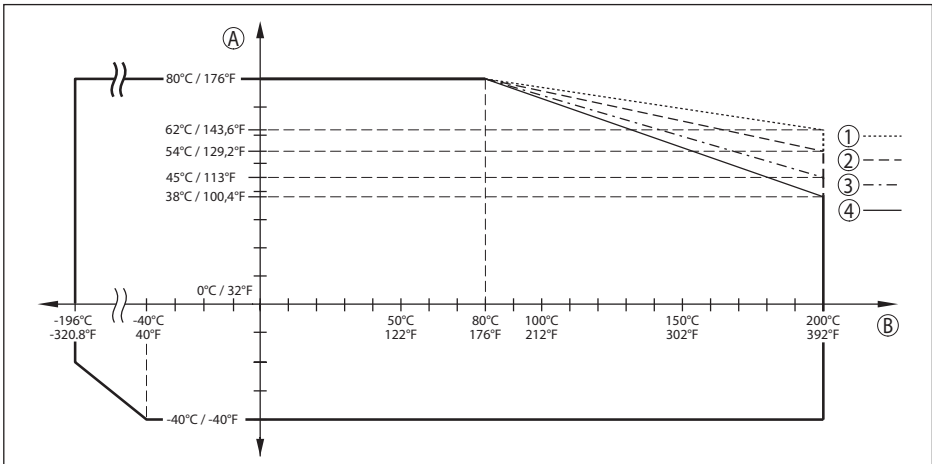
插图. 74: 环境温度降额, 带塑料天线系统的法兰 -196 ... +200 °C (-320.8 ... +392 °F)
