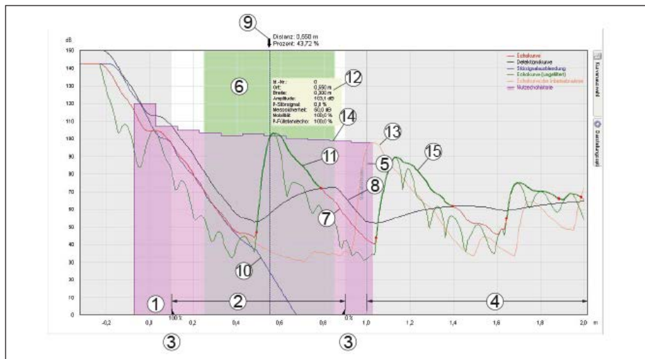
插图. 63: 在回波曲线窗口内的范围连同具有“扩展的显示区域”的显示选项
