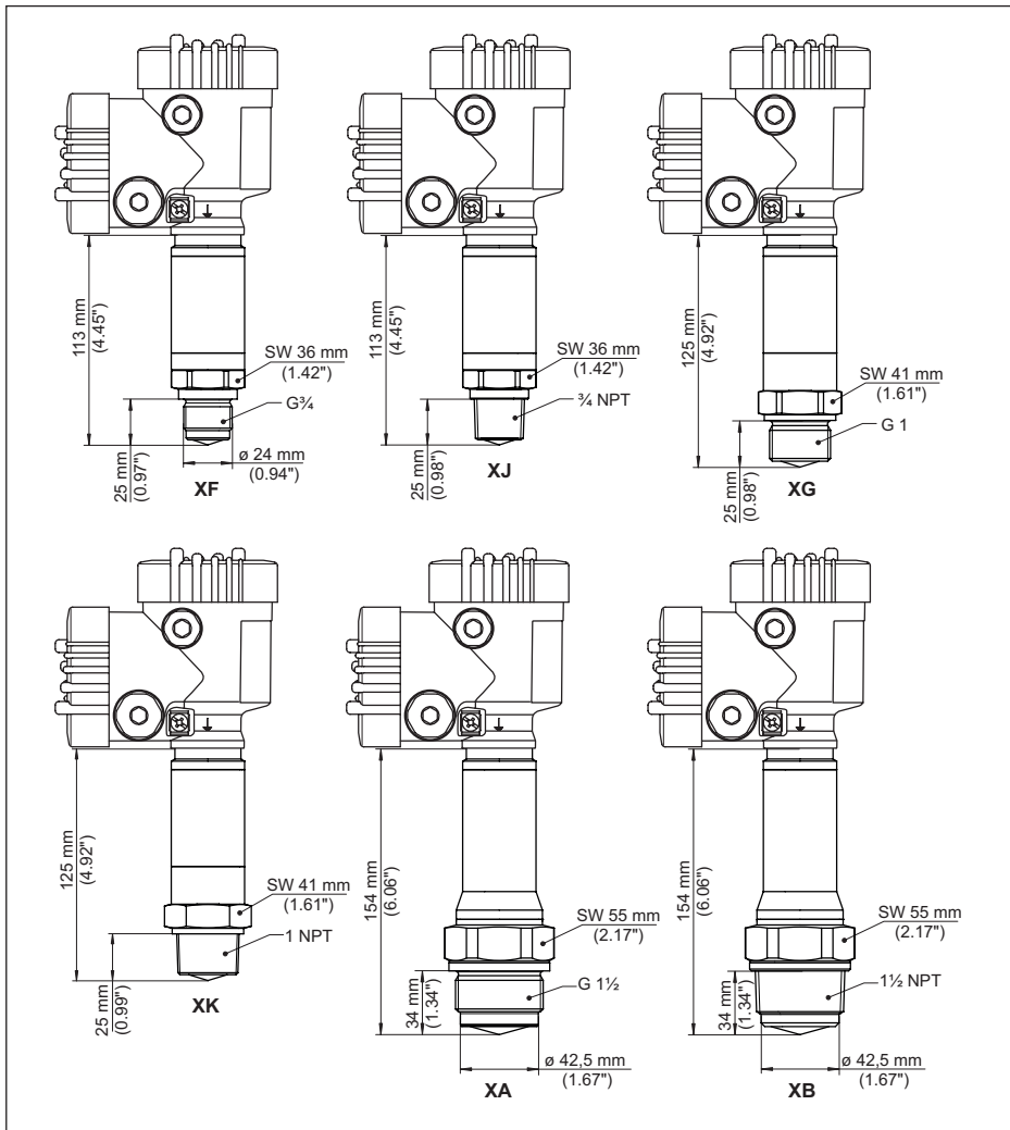
插图 90: VEGAPULS 6X, 带有内置天线系统的螺纹至 +200 °C (+392 °F) 和 +250 °C (+482 °F)
