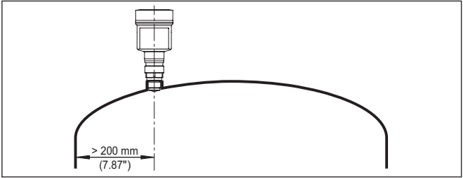
插图. 17: 将雷达传感器安装在圆形容器盖上
