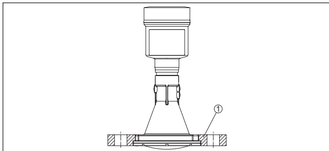
插图. 14: 组合式锁紧法兰
