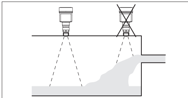
插图. 21: 流入介质时安装雷达传感器
