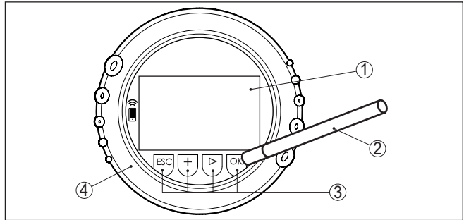
插图. 50: 显示和调整元件 - 拥有磁笔操作功能
