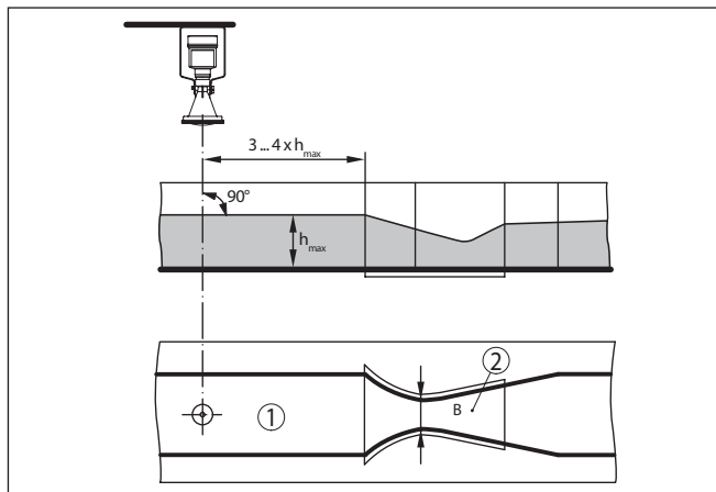
插图. 44: 用卡发基-文丘里槽来测量流量: h_{\max} = 水槽的最大灌装量; B = 水槽的最大收缩率
