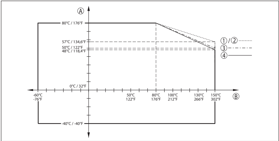
插图. 72: 环境温度降额，带塑封天线系统的法兰 -60 ... +150 °C (-76 ... +302 °F)
