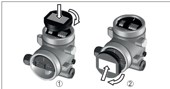
插图. 48: 将显示和调整模块装到双腔式壳体上
