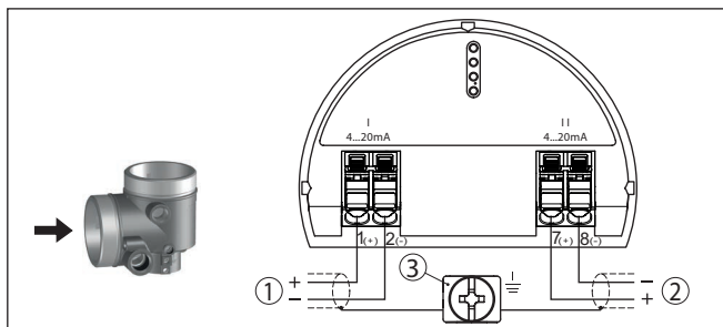
插图. 47: 双腔式壳体的接线腔
