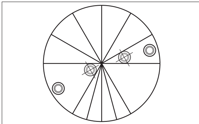
插图. 37: 在多腔式料仓中进行安装和校准
