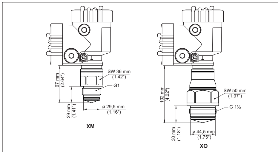
插图. 96: VEGAPULS 6X，用于卫生型适配器的螺纹
