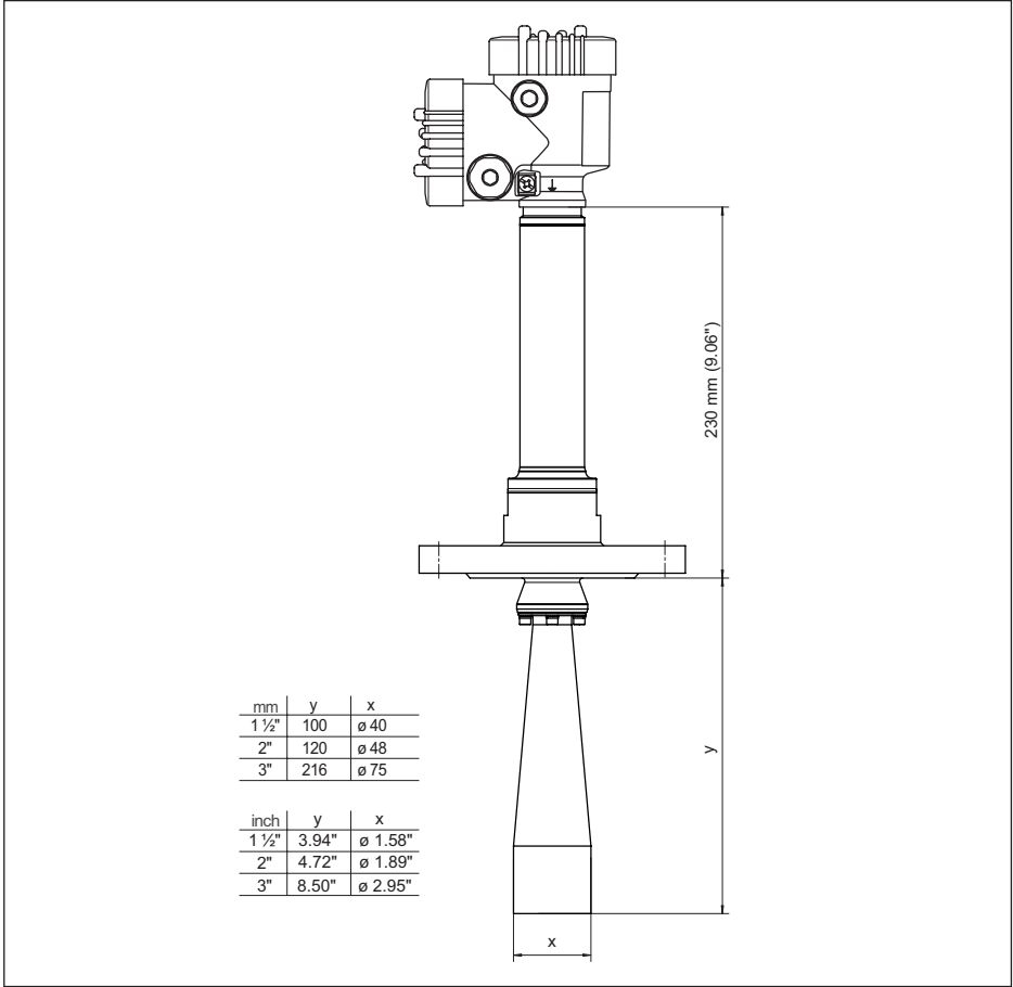
插图. 93: VEGAPULS 6X, 带有号角天线的法兰, 450 °C 型
