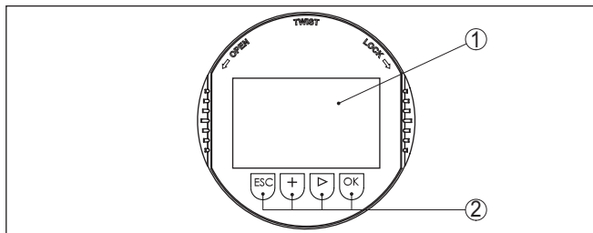
插图. 49: 显示和调整元件
