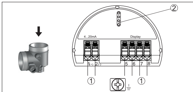
插图. 46: 双腔式外壳的电子部件腔
