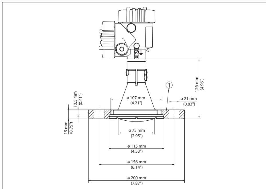
插图. 83: VEGAPULS 6X 带有锁紧法兰，适用于法兰 3" 150 lbs, DN 80 PN 16
