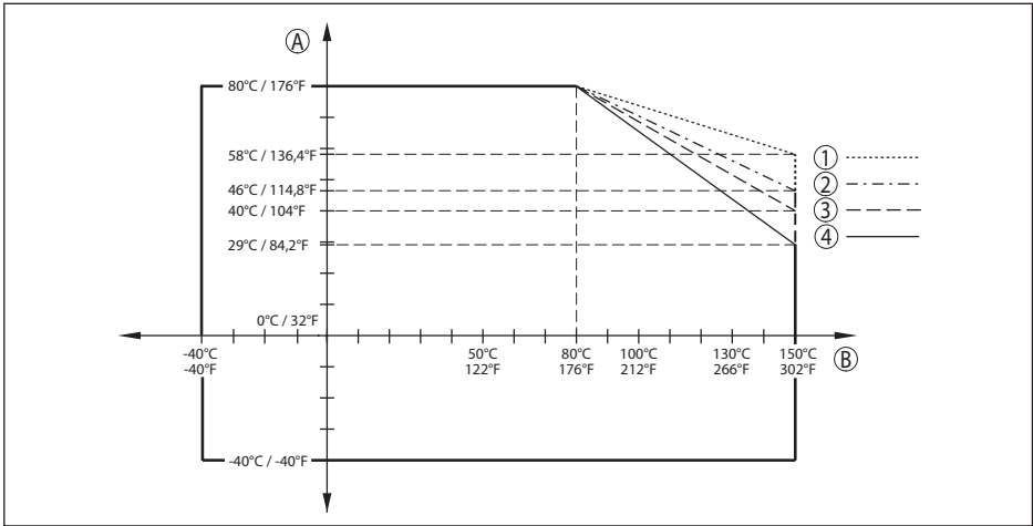
插图. 68: 环境温度降额，带内置天线系统的螺纹，至 +150 °C (+302 °F)
