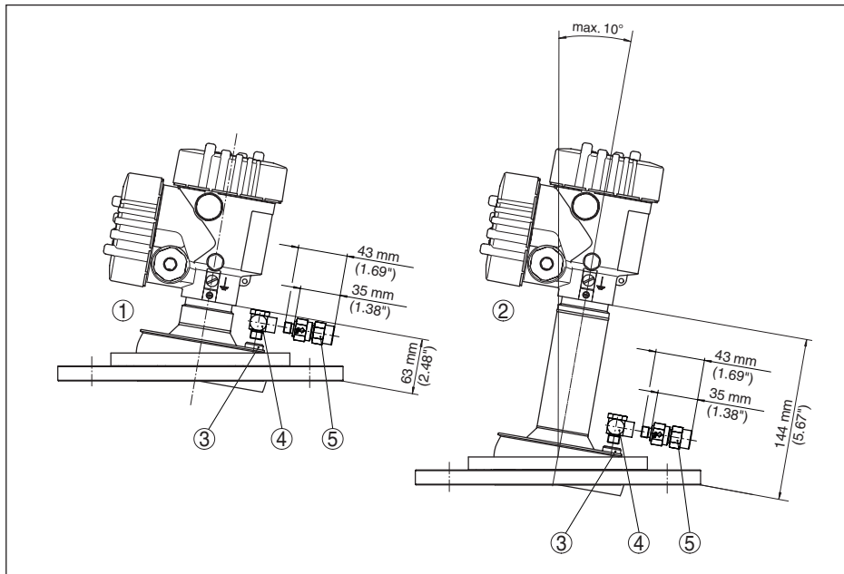
插图. 102: VEGAPULS 6X, 带有透镜天线、万向节和吹气接口的法兰
