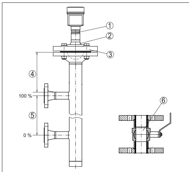
插图. 42: 旁路的构造
