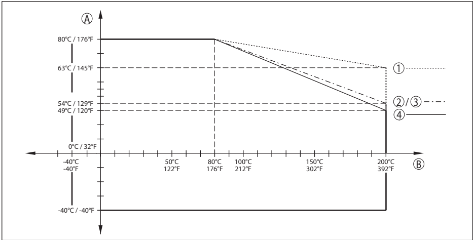
插图. 76: 环境温度降额, 带透镜天线的法兰, 至 +200 °C (+392 °F)
