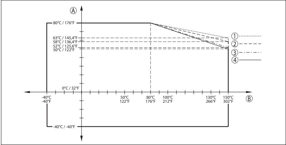
插图. 75: 环境温度降额, 带透镜天线的法兰, 至 +150 °C (+302 °F)
