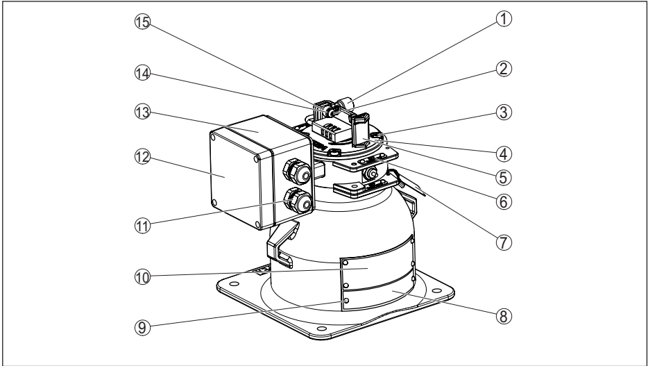
Fig. 34: Matériaux VEGASOURCE 82 - Version X, C - avec commutateurs de position ON/OFF
