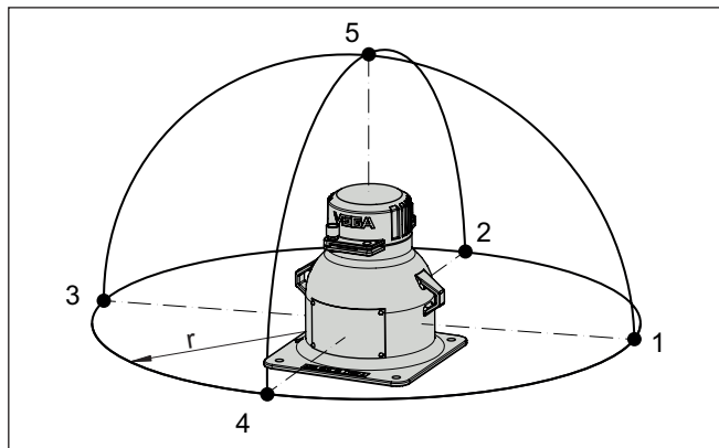
Fig. 31: Points de mesure pour la mesure de débit de dose locale
