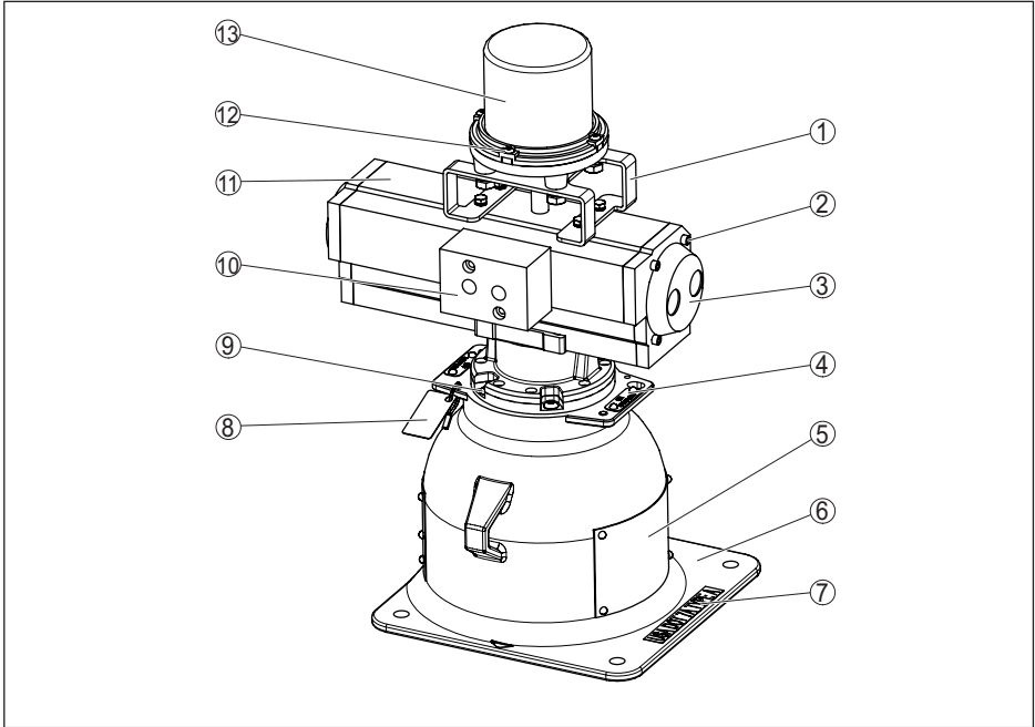
Fig. 36: Matériaux VEGASOURCE 82 - version B
