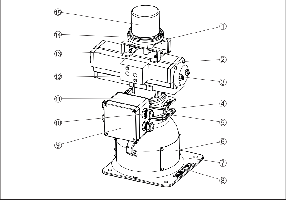
Fig. 37: Matériaux VEGASOURCE 82 - Version B - avec commutateurs de position ON/OFF
