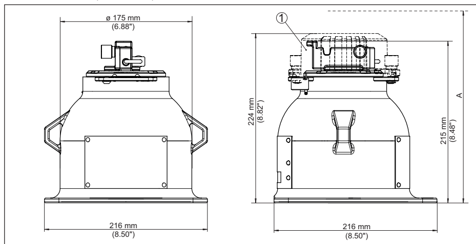
Fig. 38: Conteneur blindé VEGASOURCE 82, version X, C - commutation MARCHE/ARRÊT manuelle
