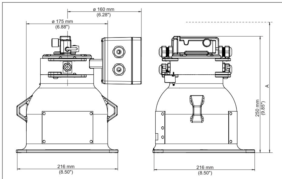
Fig. 39: Conteneur blindé VEGASOURCE 82, version X, C - Commutation MARCHÉ/ARRÊT manuelle avec commutateurs de position MARCHÉ/ARRÊT
