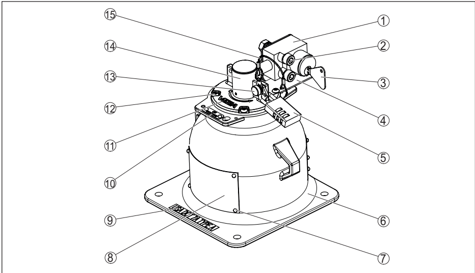
Fig. 35: Matériaux VEGASOURCE 82 - Version X, C - avec commutateur Interlock
