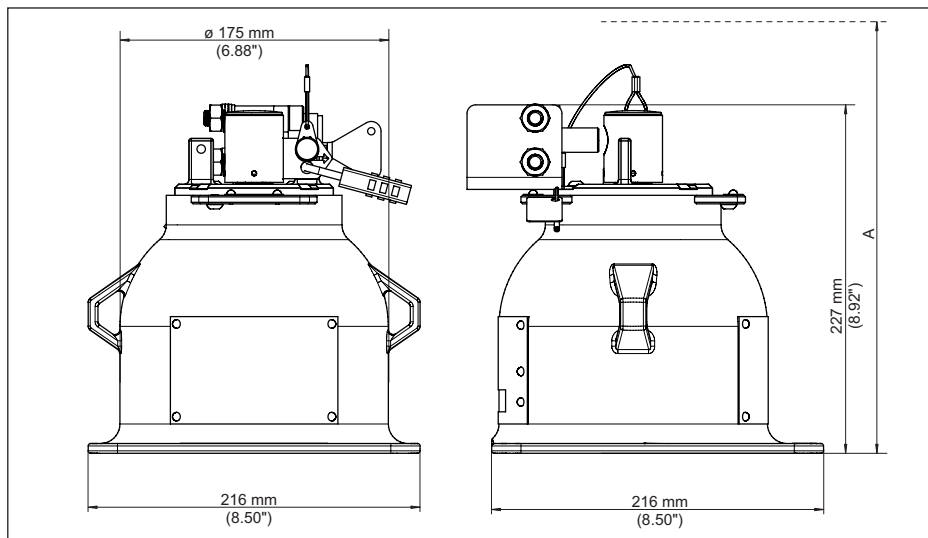
Fig. 40: Conteneur blindé VEGASOURCE 82, version X, C - Commutation MARCHÉ/ARRÊT manuelle avec commutateurs Interlock
