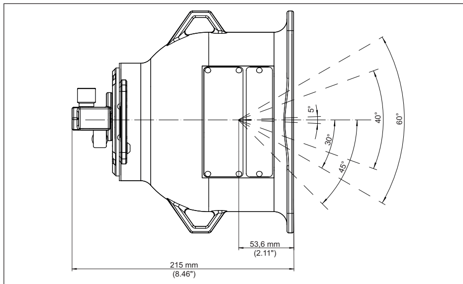
Fig. 43: Canal de sortie des rayonnements (par ex. version X, C)
