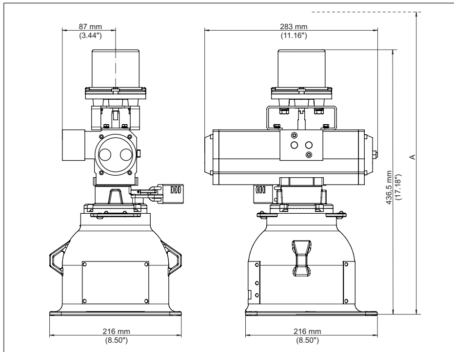
Fig. 41: Conteneur blindé VEGASOURCE 82, version B - Commutation MARCHE/ARRÊT pneumatique
