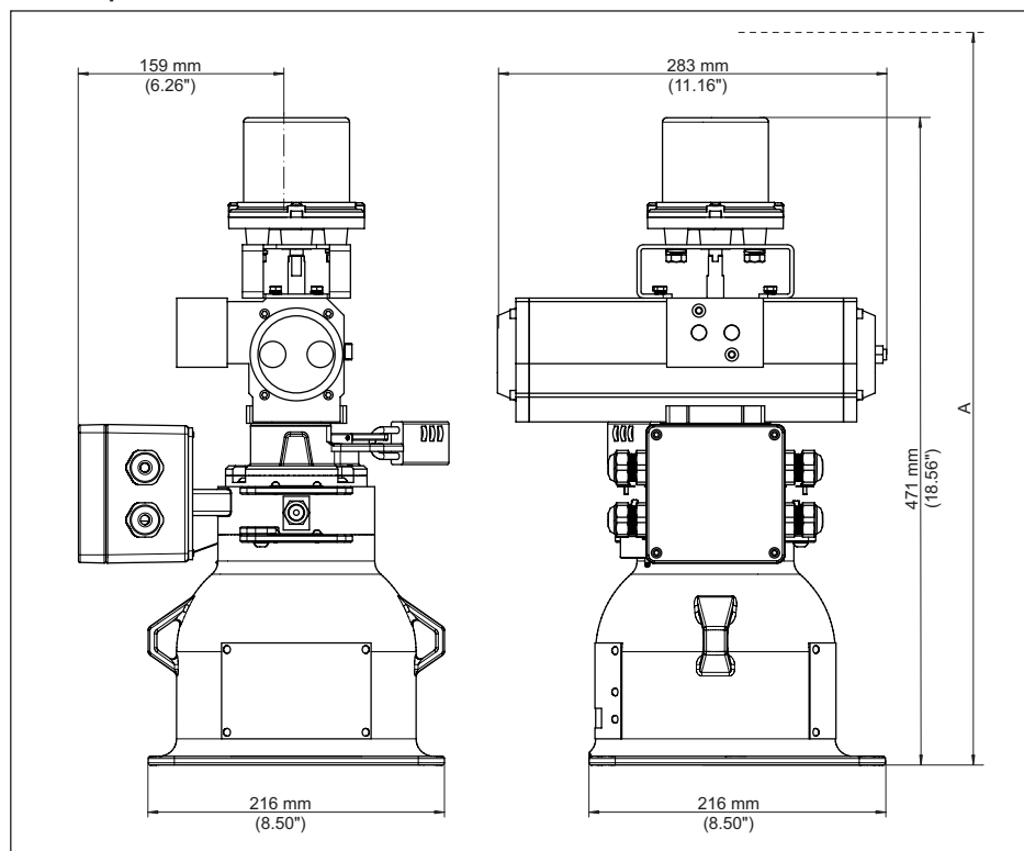
Fig. 42: Conteneur blindé VEGASOURCE 82, version B - Commutation MARCHE/ARRÊT pneumatique avec commutateurs MARCHE/ARRÊT
