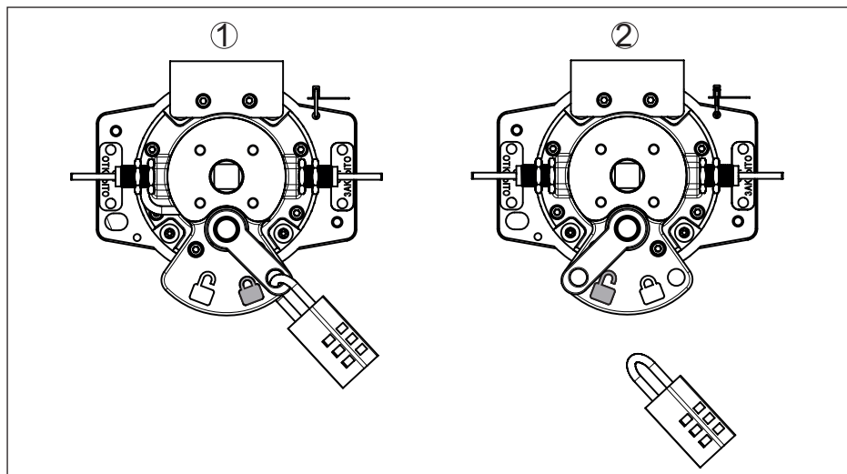
Fig. 30: Affichage de l'état de commutation sur VEGASOURCE 82 - Version B - Commutation MARCHE/ARRÊT pneumatique
