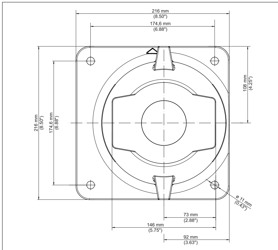
Fig. 43: Basisplaat met boringen (bijv. uitvoering X, C)
