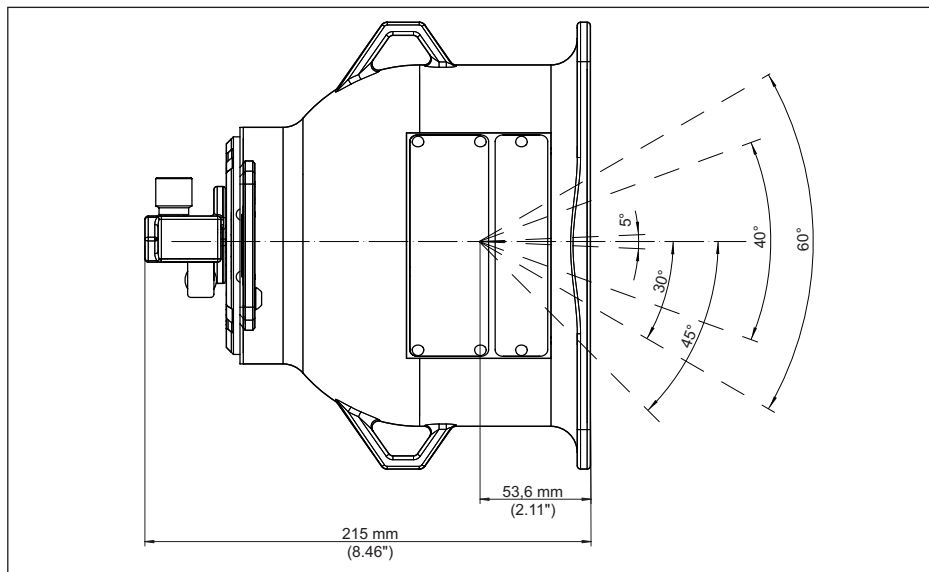
Fig. 42: Stralingskanaal (bijv. uitvoering X, C)
