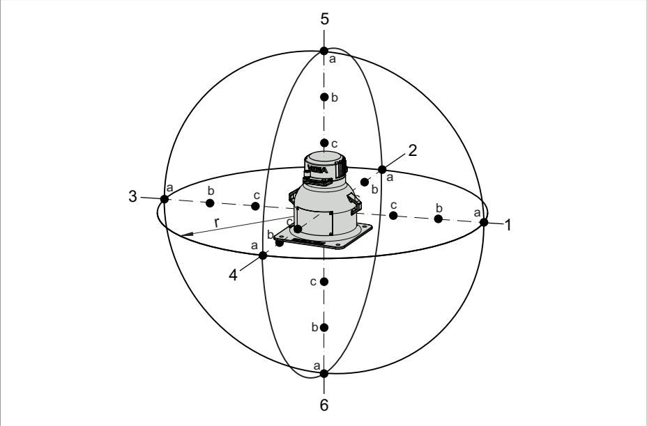
Fig. 36: Iso-afstandscurve (afstand: 1 m) - voorbeeld: bronhouder VEGASOURCE 82 met Cs-137, 200 mCi (7,4 GBq)
