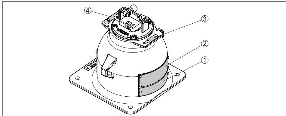
Fig. 3: Positie van de typeplaten, bijv. uitvoering X, C, handmatige omschakeling
