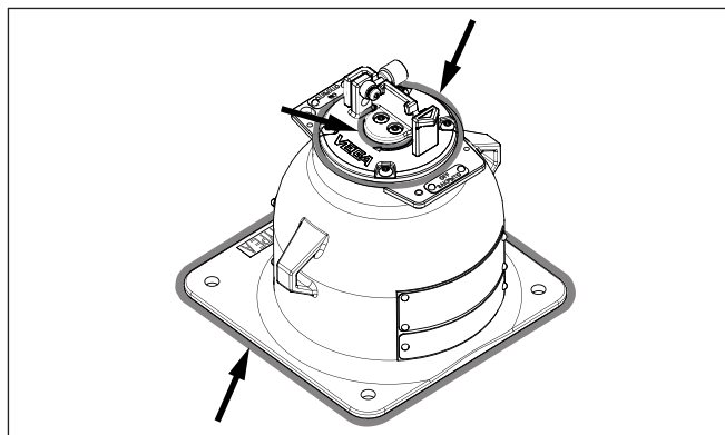
Fig. 30: Veegvlakken voor de dichtheidstest - uitvoering X, C
