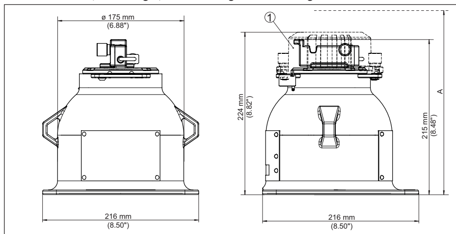
Fig. 37: Bronhouder VEGASOURCE 82, uitvoering X, C - handmatige omschakeling
