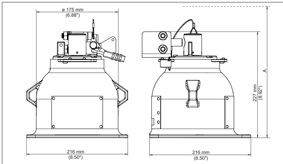
Fig. 39: Bronhouder VEGASOURCE 82, uitvoering X, C - handmatige omschakeling, met interlock-schakelaar
