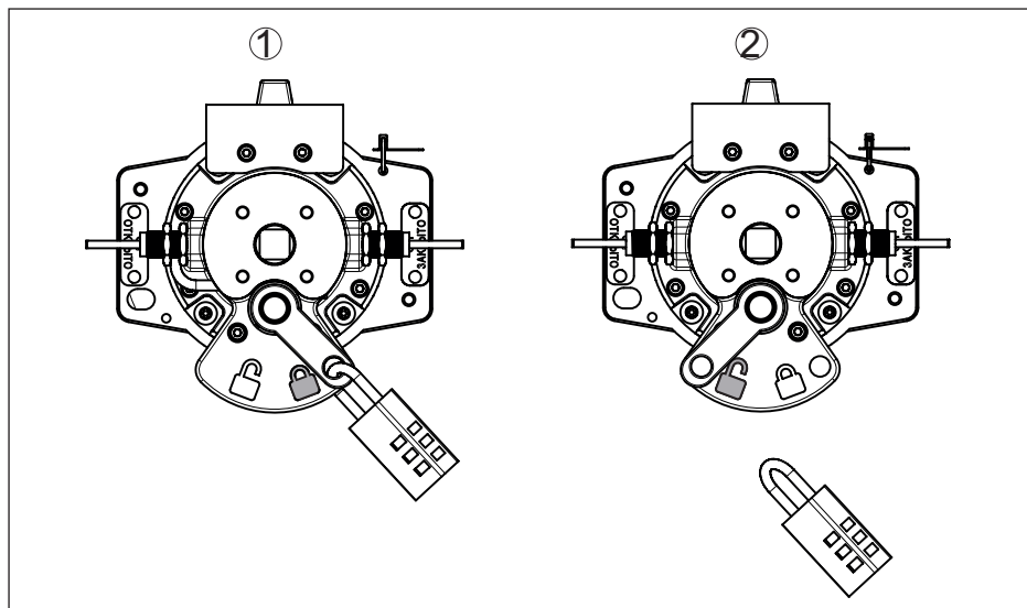
Fig. 28: Indicatie van de schakelstand bij VEGASOURCE 82 - uitvoering B, pneumatische omschakeling
