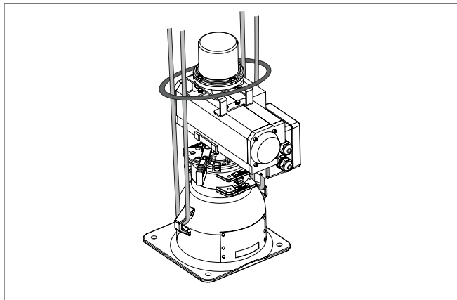
Fig. 8: Heffen van een bronhouder met pneumatische omschakeling
