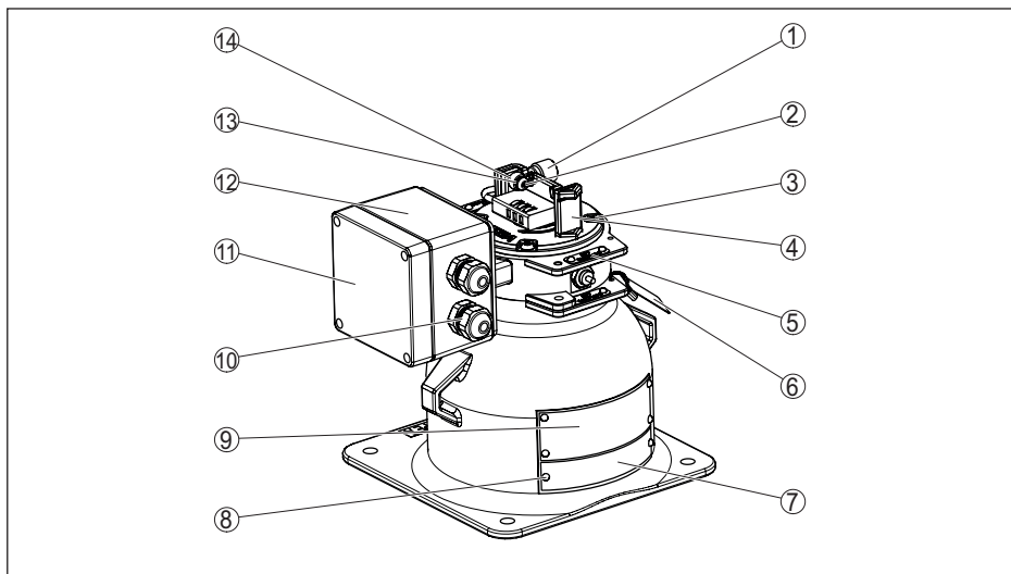
Fig. 32: Materialen VEGASOURCE 82 - uitvoering X, C, met ON/OFF-positieschakelaars
