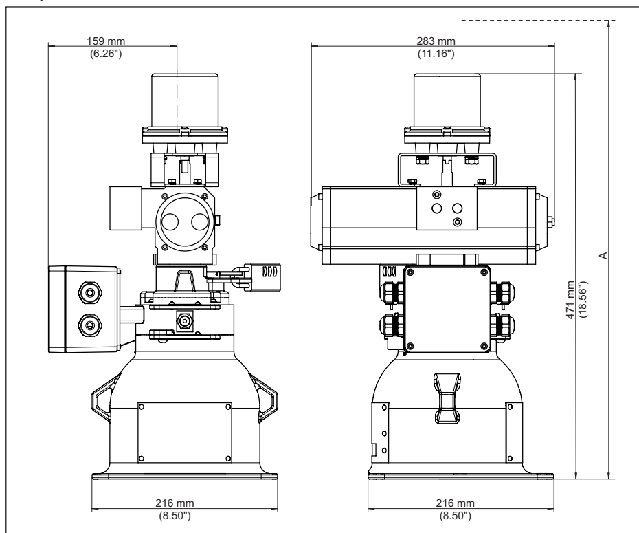
Fig. 41: Bronhouder VEGASOURCE 82, uitvoering B - pneumatische omschakeling met ON/OFF-positieschakelaars
