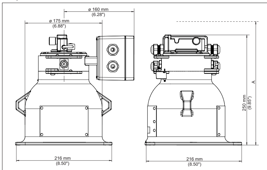
Fig. 38: Bronhouder VEGASOURCE 82, uitvoering X, C - handmatige omschakeling, met ON/OFF-positieschakelaars
