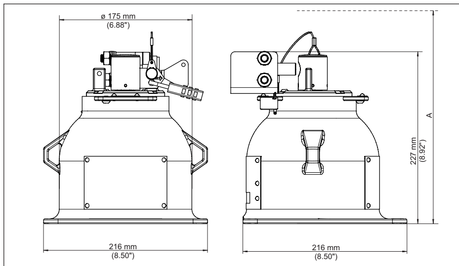
Fig. 40: Bronhouder VEGASOURCE 82, uitvoering X, C - handmatige ON/OFF-schakeling, met interlock-schakelaar
