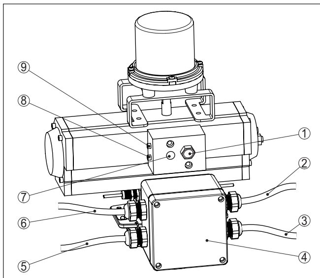
Fig. 23: Aansluiting van de persluchtleidingen op VEGASOURCE 82 - uitvoering B
