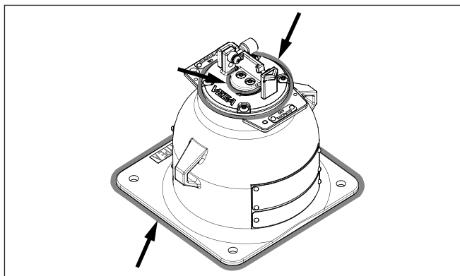
Fig. 32: Veegvlakken voor de contaminatiebeproeving - uitvoering X, C
