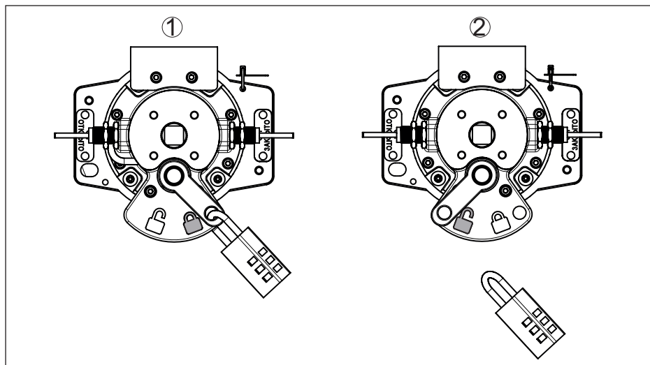
Fig. 30: Indicatie van de schakelstand bij VEGASOURCE 82 - uitvoering B, pneumatische ON/OFF-schakeling
