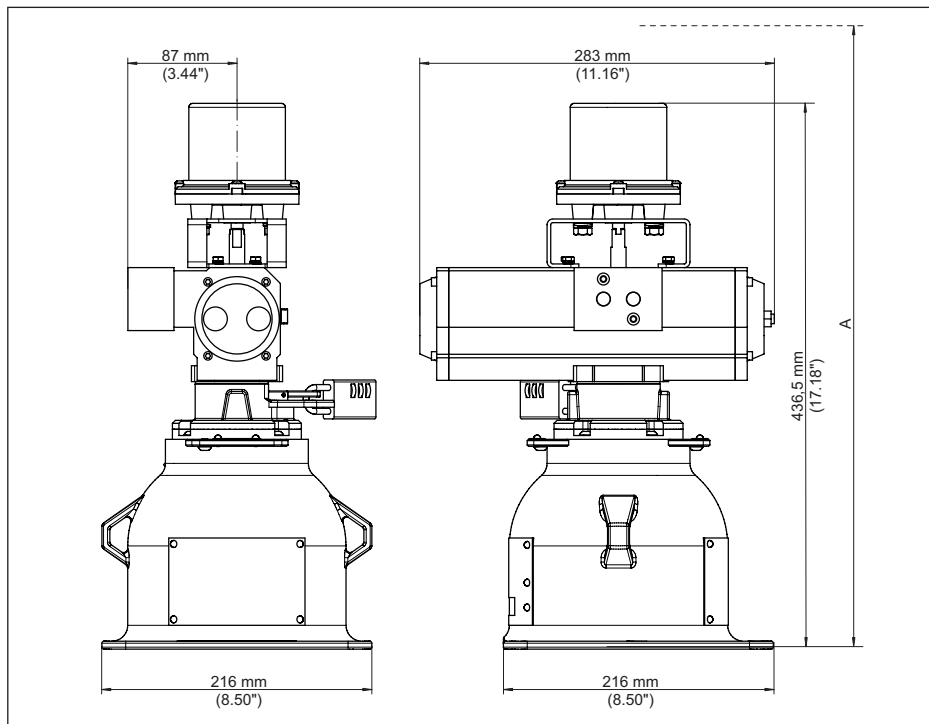
Fig. 41: Bronhouder VEGASOURCE 82, uitvoering B - pneumatische ON/OFF-schakeling
