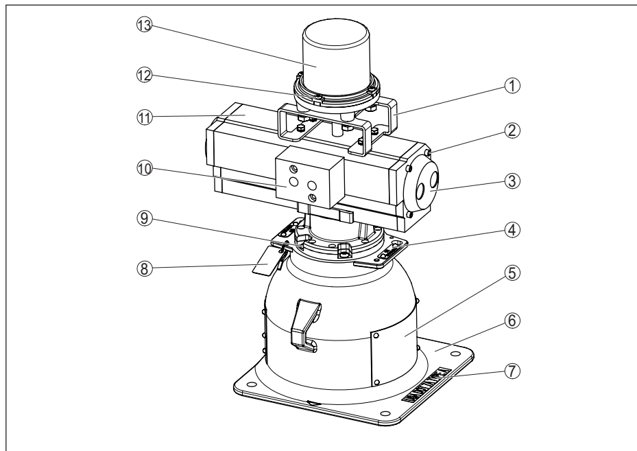
Fig. 36: Materialen VEGASOURCE 82 - uitvoering B
