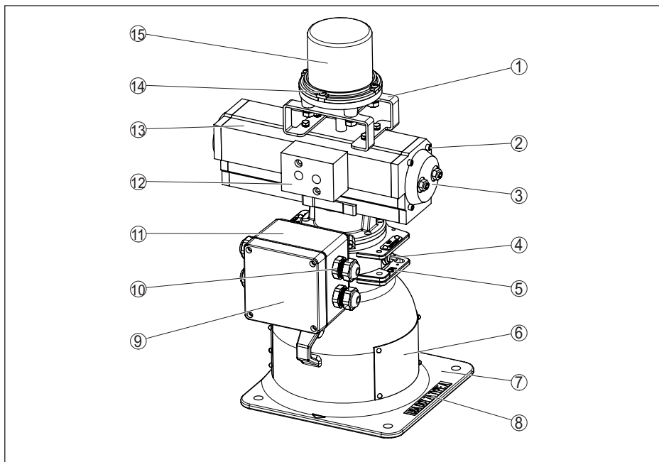
Fig. 37: Materialen VEGASOURCE 82 - uitvoering B, met ON/OFF-positieschakelaars
