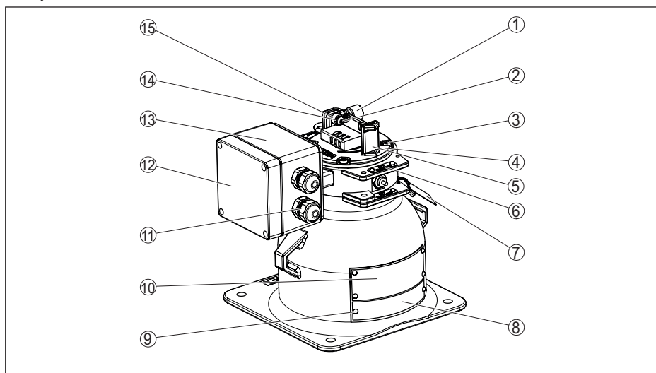
Fig. 34: Materialen VEGASOURCE 82 - uitvoering X, C, met ON-/OF-positieschakelaars
