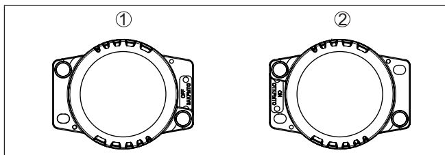
Fig. 29: Positie-indicatie met beschermkap - VEGASOURCE 82 uitvoering X, C
