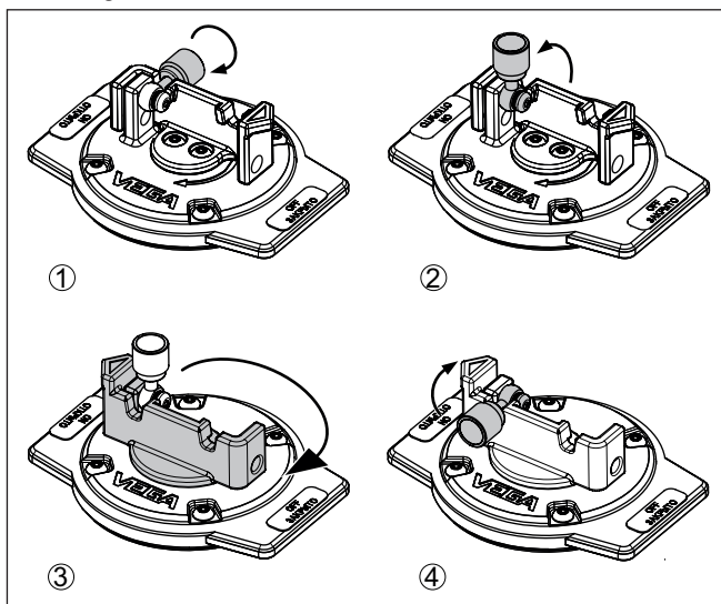
Fig. 26: Inschakelen van de straling - VEGASOURCE 82 uitvoering X, C
