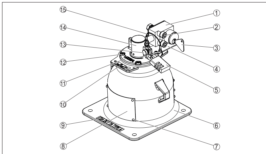
Fig. 35: Materialen VEGASOURCE 82 - uitvoering X, C, met interlock-schakelaar
