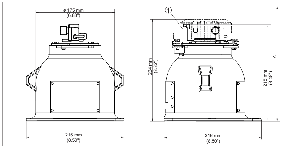
Fig. 38: Bronhouder VEGASOURCE 82, uitvoering X, C - handmatige ON/OFF-schakeling
