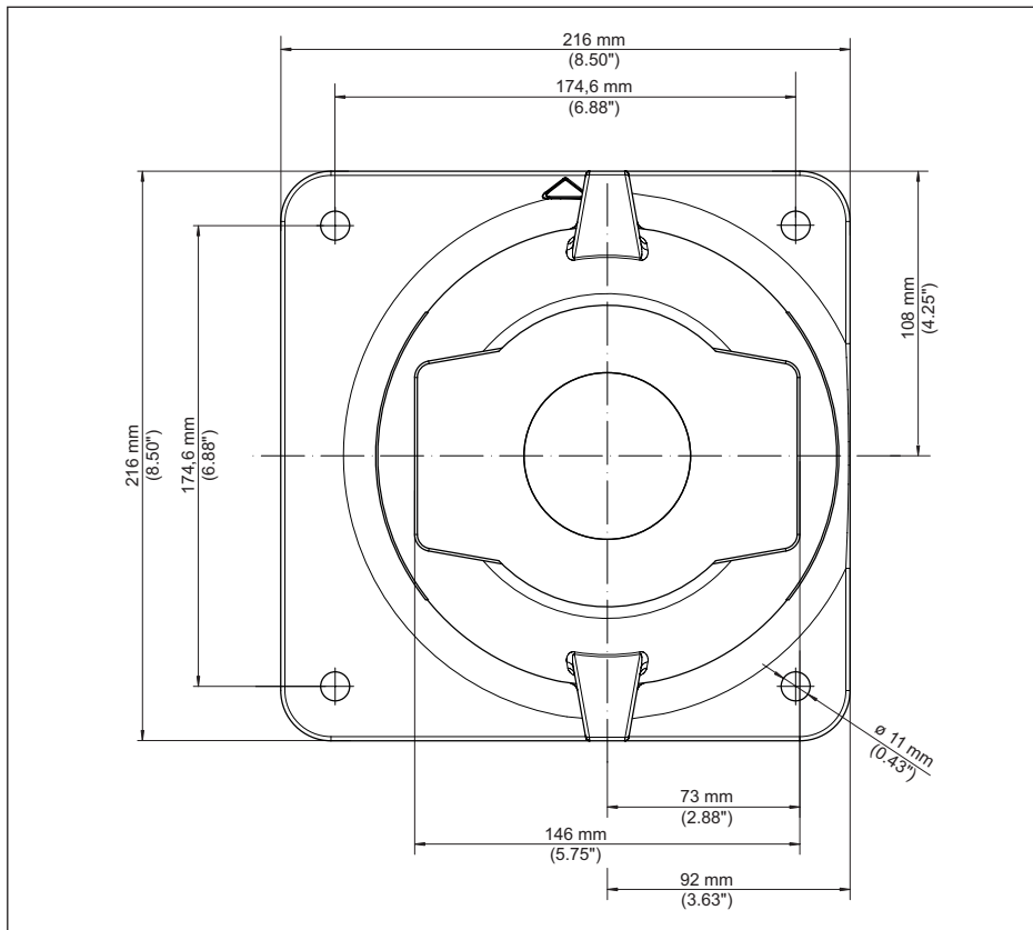
Fig. 44: Basisplaat met boringen (bijv. uitvoering X, C)
