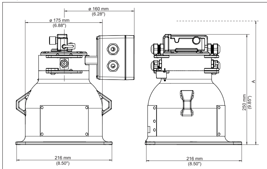
Fig. 39: Bronhouder VEGASOURCE 82, uitvoering X, C - handmatige ON/OFF-schakeling met ON/OFF-positieschakelaars
