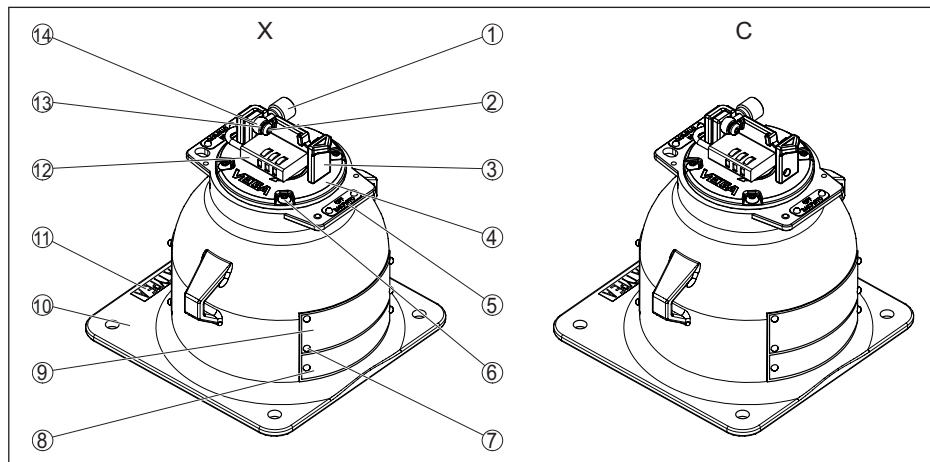
Fig. 33: Materialen VEGASOURCE 82 - uitvoering K, C
