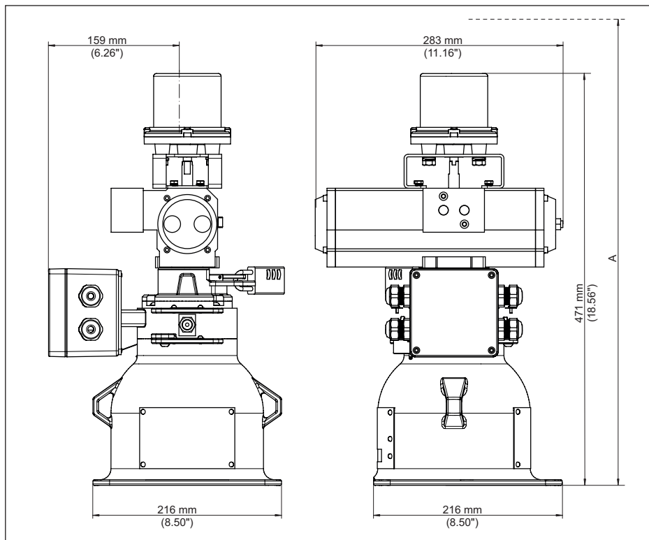
Fig. 42: Bronhouder VEGASOURCE 82, uitvoering B - pneumatische ON/OFF-schakeling met ON-/OFF-positieschakelaars
