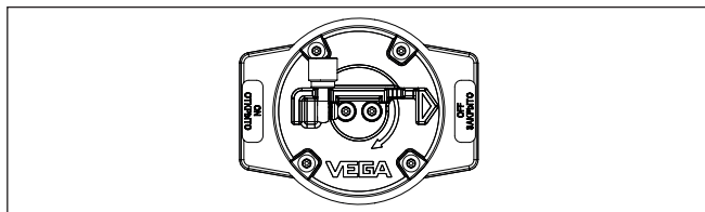
Fig. 28: Straling "OFF" - VEGASOURCE 82 uitvoering X, C
