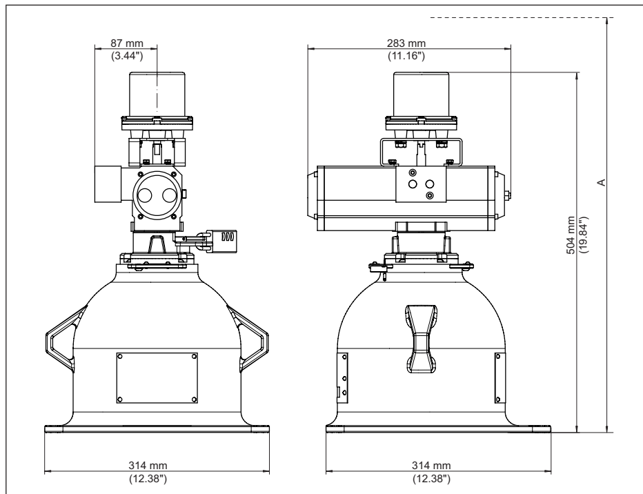
Fig. 41: Conteneur blindé VEGASOURCE 83, version B - Commutation MARCHE/ARRÊT pneumatique
