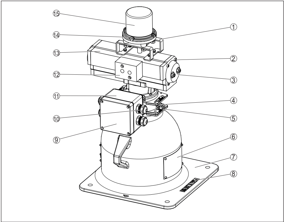
Fig. 37: Matériaux VEGASOURCE 83 - Version B - avec commutateurs de position ON/OFF
