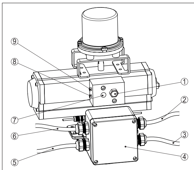
Fig. 23: Raccordement des conduites d'air comprimé sur le VEGASOURCE 83 - Version B
