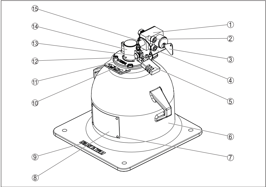
Fig. 35: Matériaux VEGASOURCE 83 - Version X, C - avec commutateur Interlock
