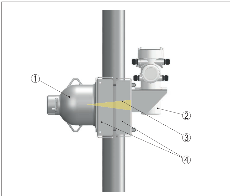
Fig. 47: Dispositif de fixation KV 31 pour le montage sur tuyauterie de 50 à 220 mm (1.97 ... 8.66 in) avec rayonnement diagonal de 30°
