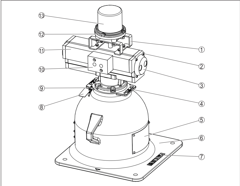
Fig. 36: Matériaux VEGASOURCE 83 - version B
