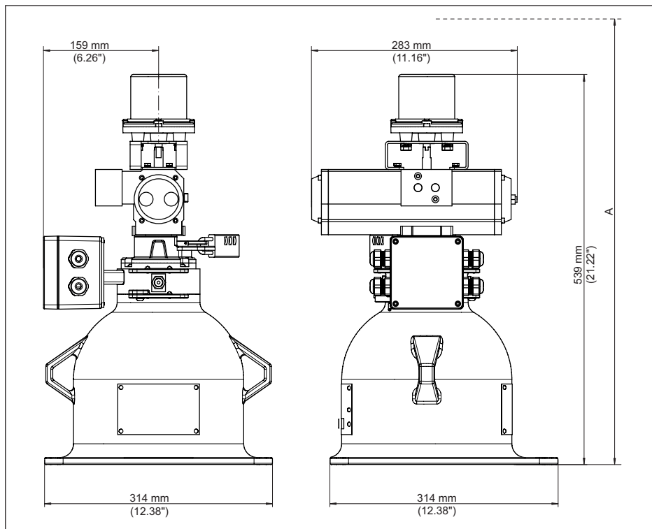
Fig. 42: Conteneur blindé VEGASOURCE 83, version B - Commutation MARCHE/ARRÊT pneumatique avec commutateurs MARCHE/ARRÊT
