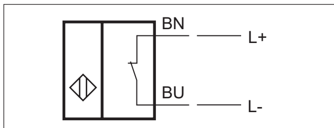
Fig. 25: Schéma de raccordement - Commutateur de position ON/OFF - NAMUR
