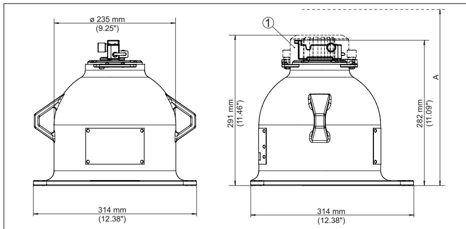
Fig. 38: Conteneur blindé VEGASOURCE 83, version X, C - commutation MARCHE/ARRÊT manuelle
