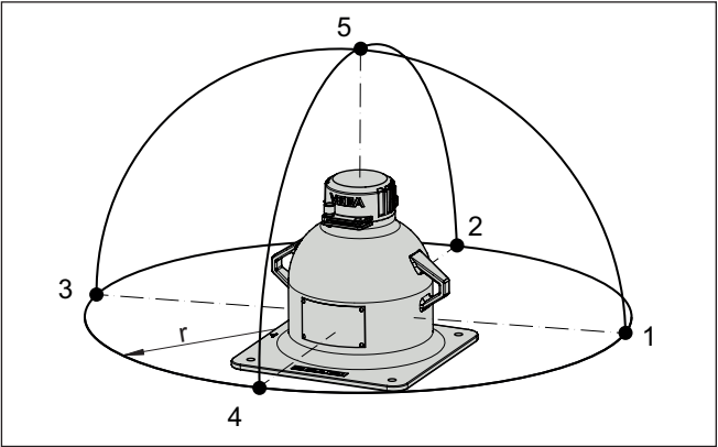
Fig. 31: Points de mesure pour la mesure de débit de dose locale r Distance par rapport au conteneur blindé 1-5 Points de mesure
