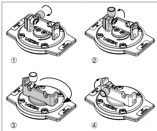
Fig. 26: Mise en marche du rayonnement - VEGASOURCE 83 Version X, C
