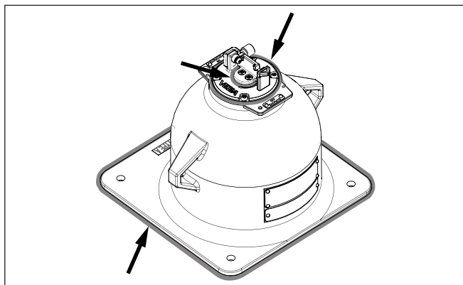
Fig. 32: Surfaces d'essuyage pour le contrôle de la contamination - Version X, C
