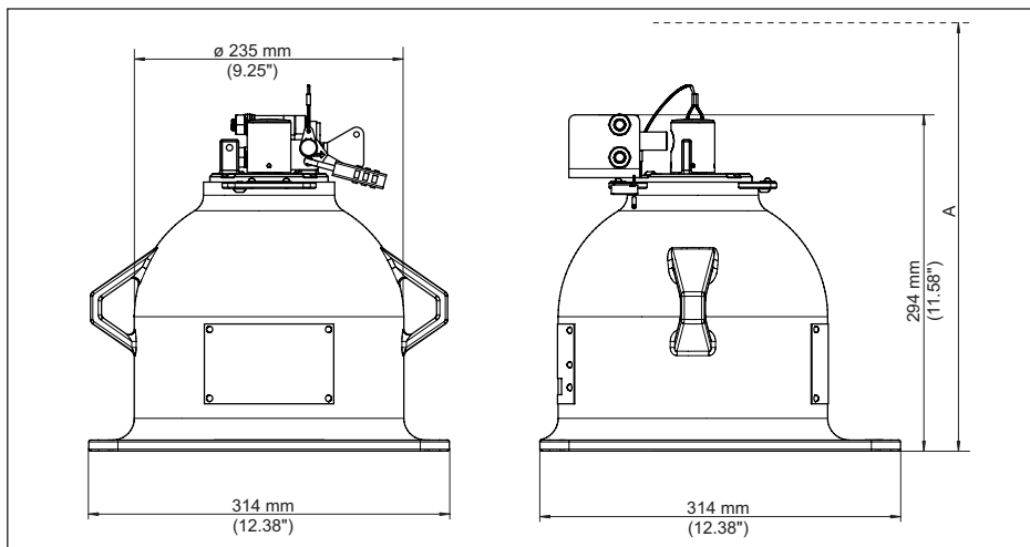
Fig. 40: Conteneur blindé VEGASOURCE 83, version X, C - Commutation MARCHÉ/ARRÊT manuelle avec commutateurs Interlock
