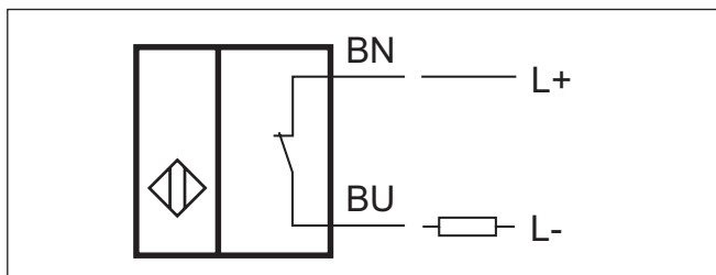
Fig. 22: Schéma de raccordement - Commutateur de position ON/OFF
