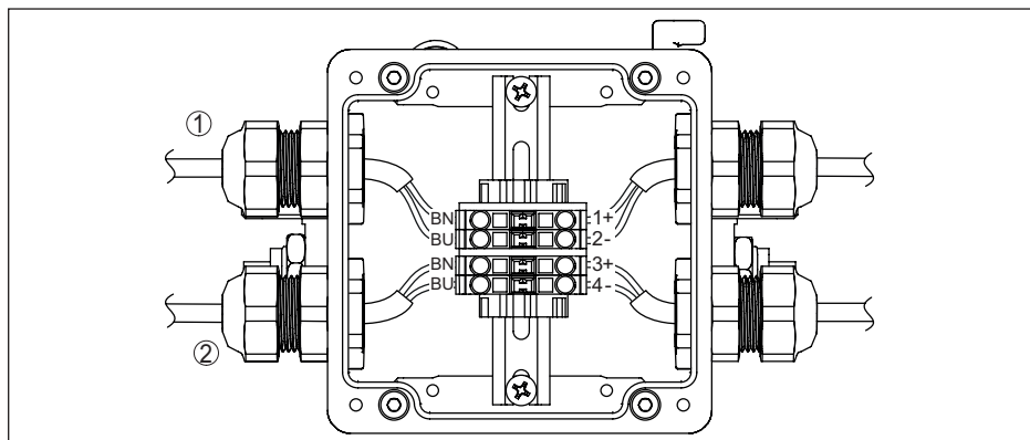
Fig. 24: Boîte à bornes de raccordement du commutateur de position ON/OFF
