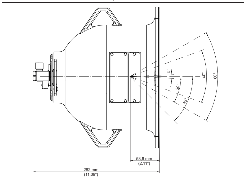
Fig. 43: Canal de sortie des rayonnements (par ex. version X, C)
