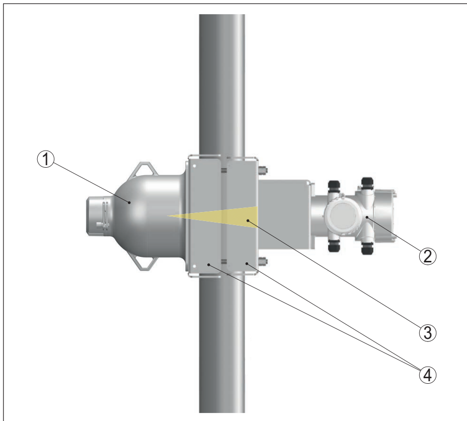
Fig. 48: Dispositif de fixation pour le montage sur une tuyauterie de 50 à 220 mm (1.97 ... 8.66 in)
