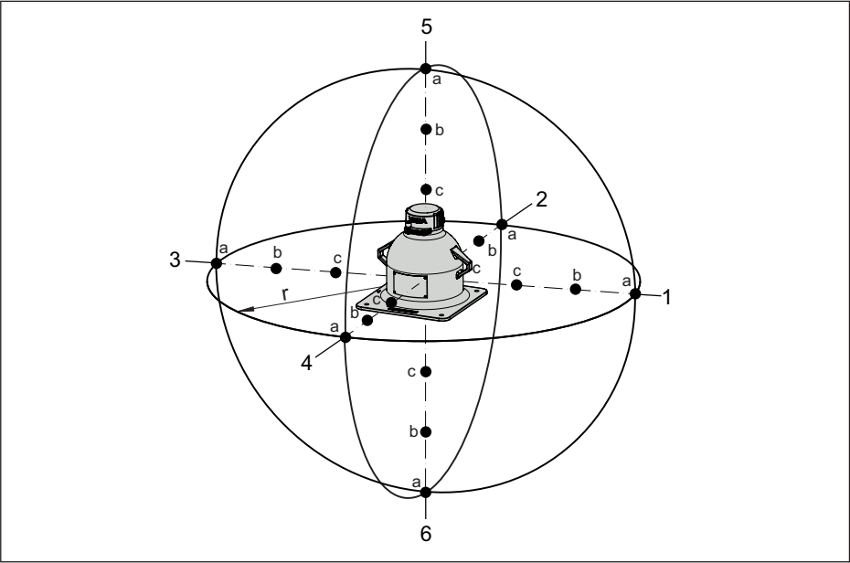
Fig. 36: Iso-afstandscurve (afstand: 1 m) - voorbeeld: bronhouder VEGASOURCE 83 met Cs-137, 5000 mCi (185 GBq)
