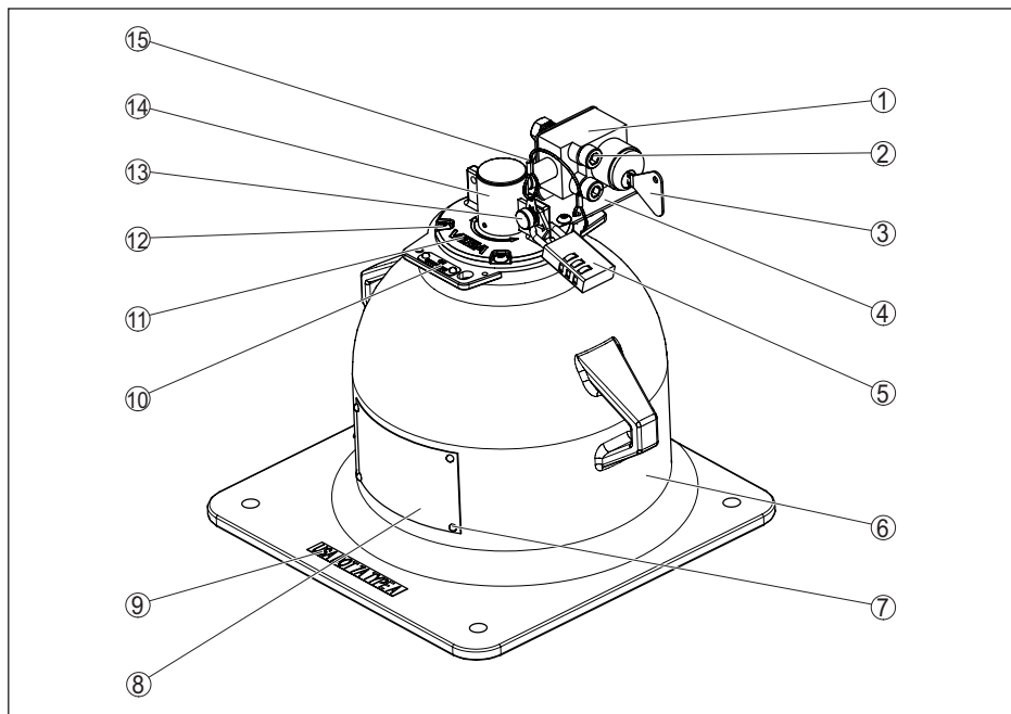
Fig. 33: Materialen VEGASOURCE 83 - uitvoering X, C, met interlock-schakelaar
