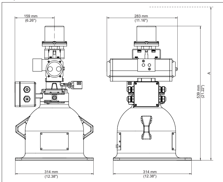
Fig. 41: Bronhouder VEGASOURCE 83, uitvoering B - pneumatische omschakeling met ON/OFF-positieschakelaars
