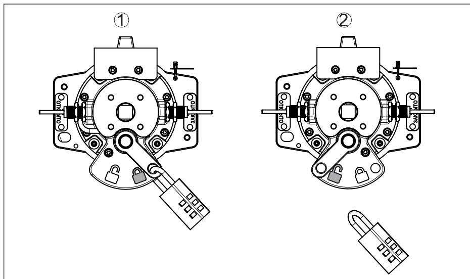
Fig. 28: Indicatie van de schakelstand bij VEGASOURCE 83 - uitvoering B, pneumatische omschakeling
