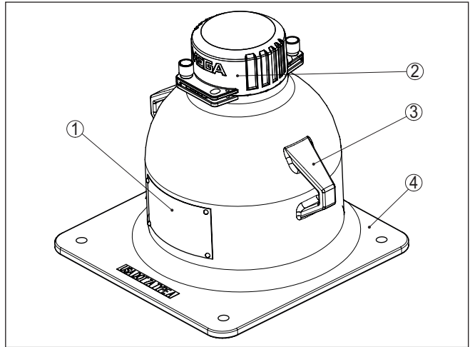
Fig. 6: Stralingsbronhouder VEGASOURCE 83
