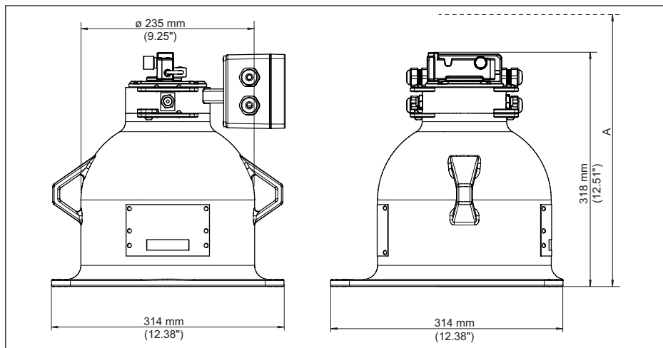
Fig. 38: Bronhouder VEGASOURCE 83, uitvoering X, C - handmatige omschakeling, met ON/OFF-positieschakelaars
