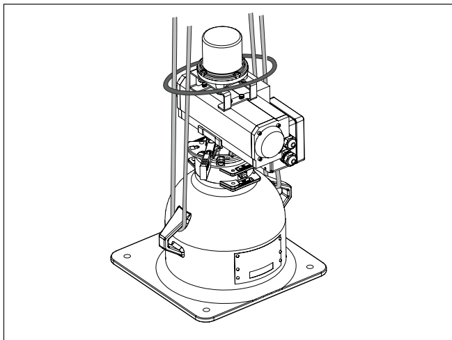
Fig. 8: Heffen van een bronhouder met pneumatische omschakeling
