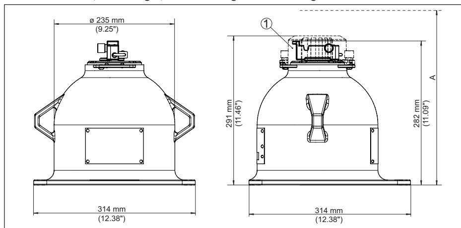
Fig. 37: Bronhouder VEGASOURCE 83, uitvoering X, C - handmatige omschakeling
