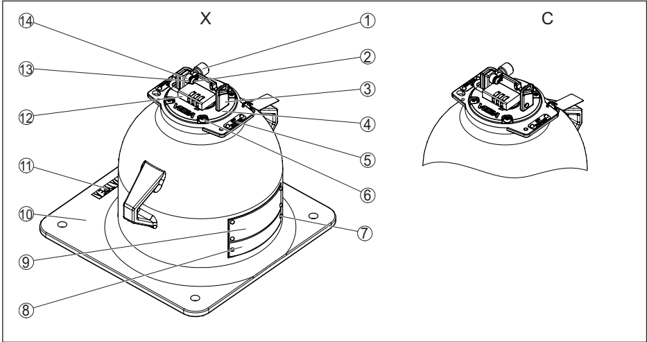
Fig. 31: Materialen VEGASOURCE 83 - uitvoering K, C
