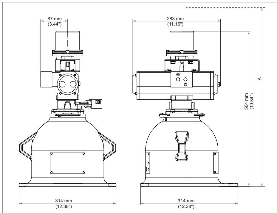
Fig. 40: Bronhouder VEGASOURCE 83, uitvoering B - pneumatische omschakeling
