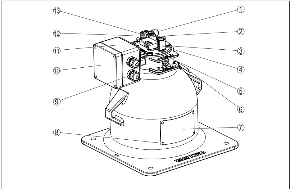
Fig. 32: Materialen VEGASOURCE 83 - uitvoering X, C, met ON/OFF-positieschakelaars
