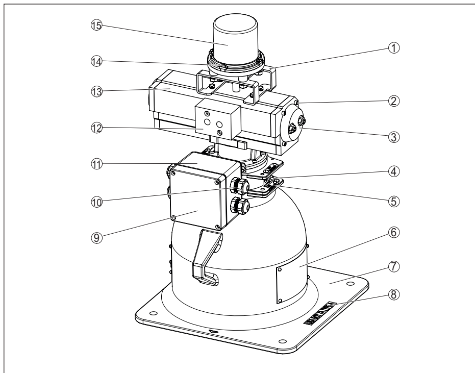
Fig. 35: Materialen VEGASOURCE 83 - uitvoering B, met ON/OFF-positieschakelaars
