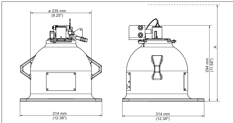
Fig. 39: Bronhouder VEGASOURCE 83, uitvoering X, C - handmatige omschakeling, met interlock-schakelaar
