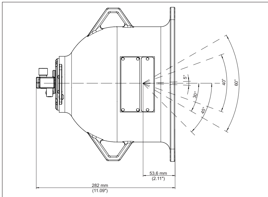
Fig. 42: Stralingskanaal (bijv. uitvoering X, C)
