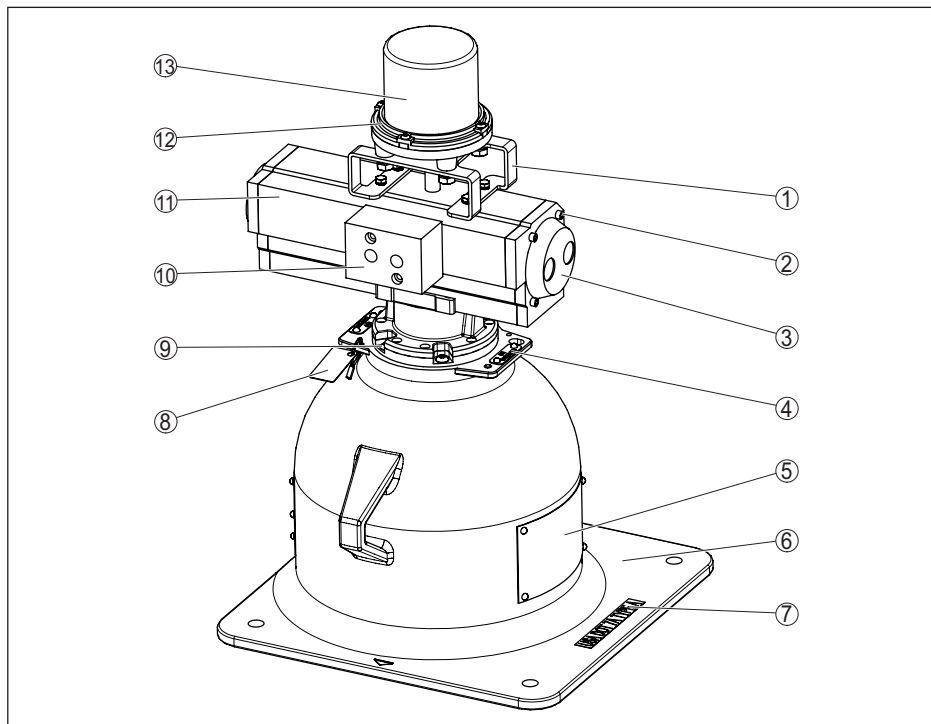
Fig. 34: Materialen VEGASOURCE 83 - uitvoering B
