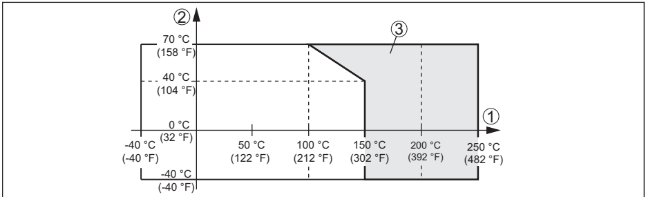
插图. 1: 环境温度 - 过程温度
