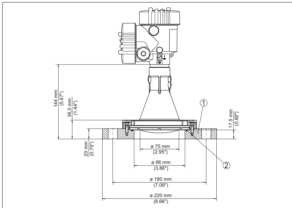
Fig. 82: VEGAPULS 6X avec bride d'adaptation DN 100 PN 6
