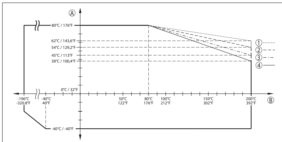
Fig. 71: Derating température ambiante, bride avec système d'antenne encapsulé -196 ... +200 °C (-320,8 ... +392 °F)
