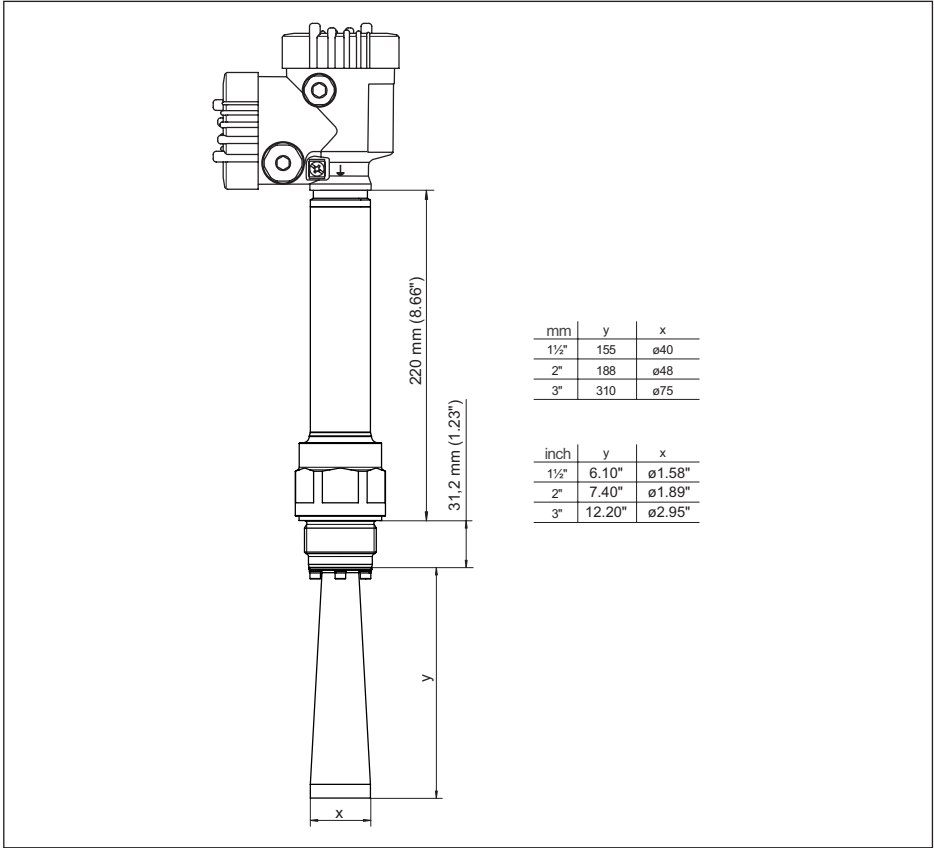
Fig. 89: VEGAPULS 6X, filetage avec antenne cône version 450 °C
