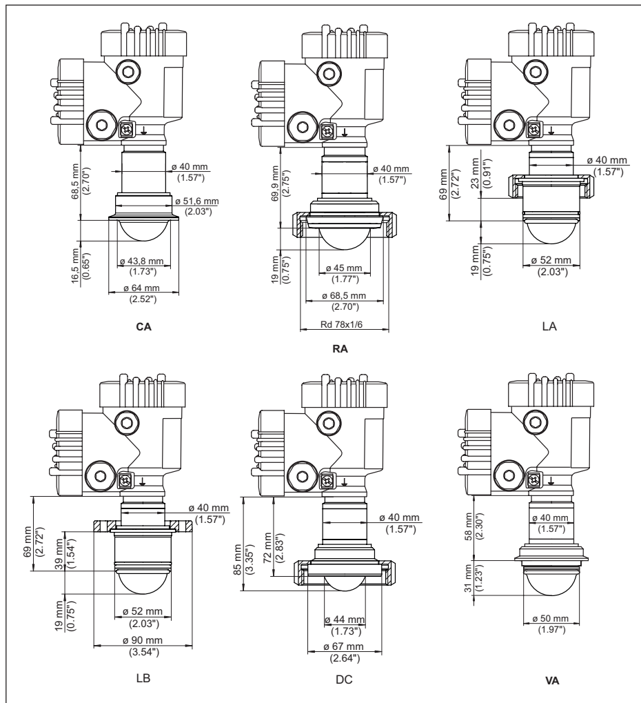
Fig. 94: VEGAPULS 6X, raccord aseptique
