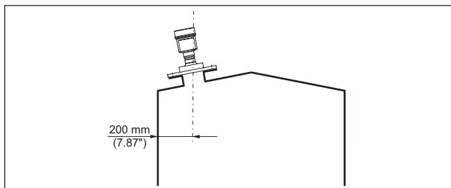
Fig. 18: Montage du capteur radar sur le toit de la cuve
