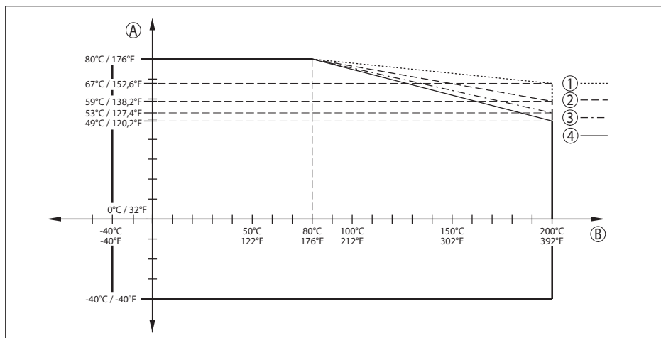
Fig. 66: Derating température ambiante, filetage avec système d'antenne intégré jusqu'à +200 °C (+392 °F)
