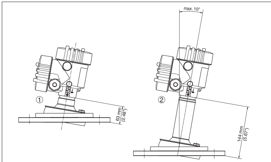
Fig. 98: VEGAPULS 6X, bride avec antenne lentille et rotule d'orientation
