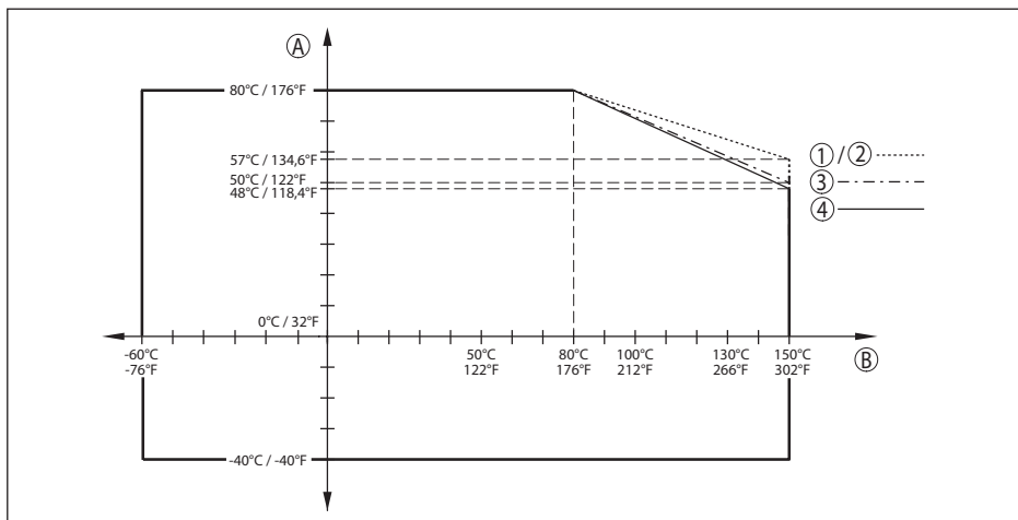
Fig. 69: Derating température ambiante, bride avec système d'antenne encapsulé -60 ... +150 °C (-76 ... +302 °F)
