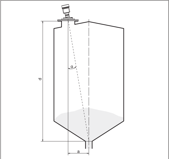
Fig. 32: Détermination de l'angle d'inclinaison pour l'alignement du VEGAPULS 6X
