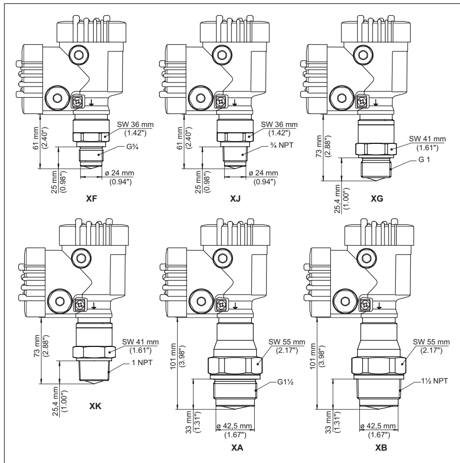
Fig. 86: VEGAPULS 6X, filetage avec système d'antenne intégré jusqu'à +150 °C (+302 °F)
