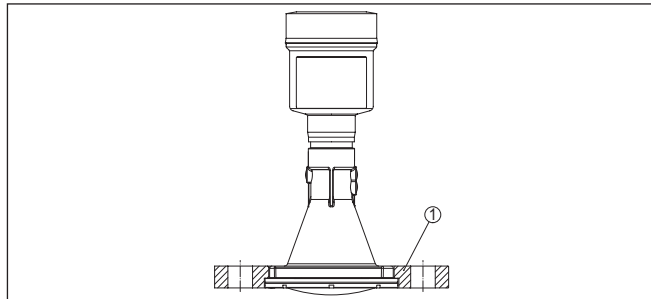
Fig. 13: Bride tournante combinée
