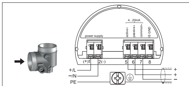
Fig. 46: Compartiment de raccordement boîtier deux chambres pour tension de réseau
