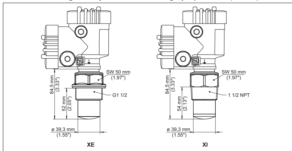
Fig. 85: VEGAPULS 6X, filetage avec système d'antenne intégré jusqu'à +80 °C (+176 °F)
