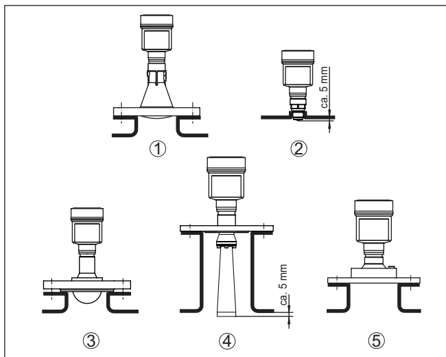
Fig. 23: Montage de rehausse recommandé sur différentes versions du VEGA-PULS 6X
