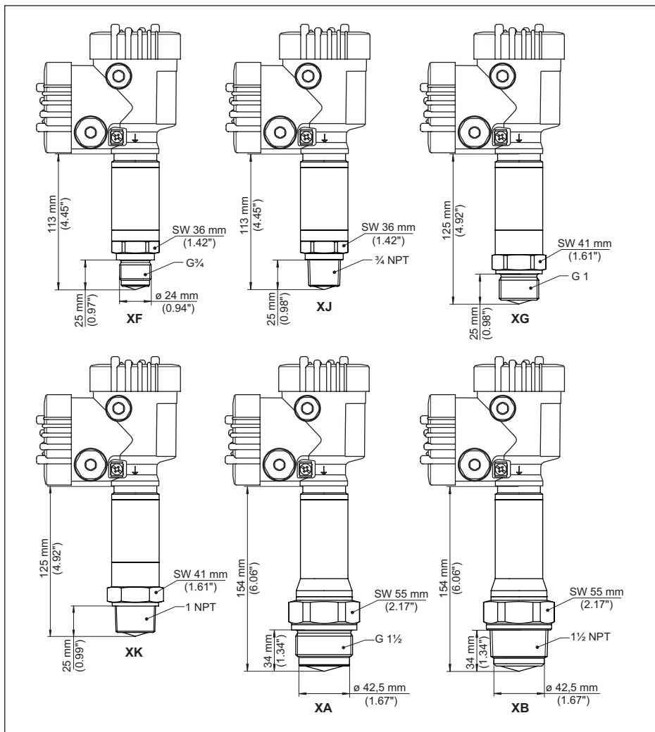
Fig. 87: VEGAPULS 6X, filetage avec système d'antenne intégré jusqu'à +200 °C (+392 °F) et +250 °C (+482 °F)
