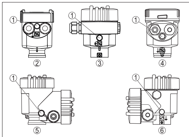
Fig. 4: Position du filtre en fonction du boîtier
