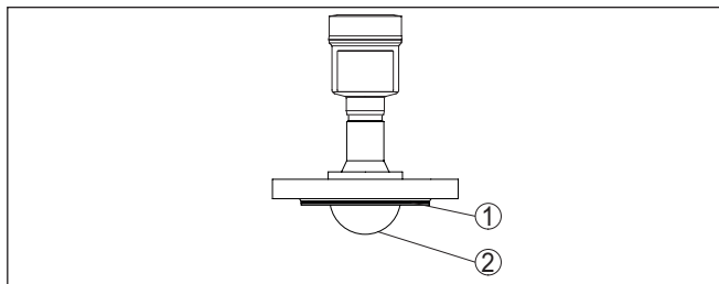
Fig. 25: VEGAPULS 6X avec bride et système d'antenne encapsulé
