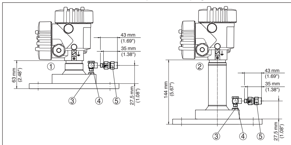
Fig. 97: VEGAPULS 6X, bride avec antenne lentille et prise d'air de purge
