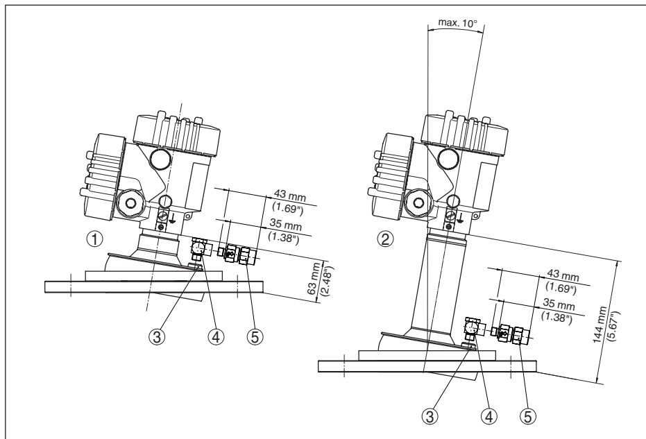
Fig. 99: VEGAPULS 6X, bride avec antenne lentille, rotule d'orientation et prise d'air de purge
