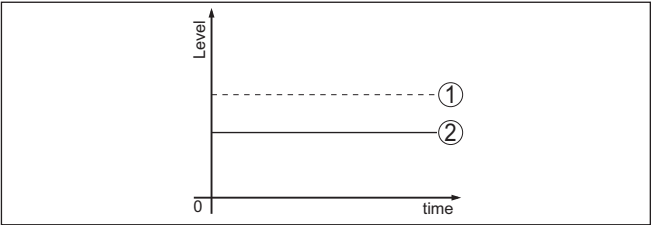
Fig. 61: Représentation des images d'erreur
