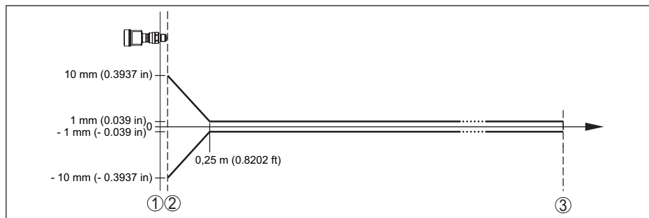
Fig. 63: Écart de mesure sous les conditions de référence (exemple filetage avec système d'antenne intégré, s'applique en conséquence pour toutes les versions) 25)
