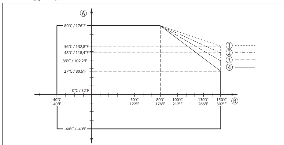
Fig. 75: Derating température ambiante, raccord hygiénique jusqu'à +150 °C (+302 °F)
