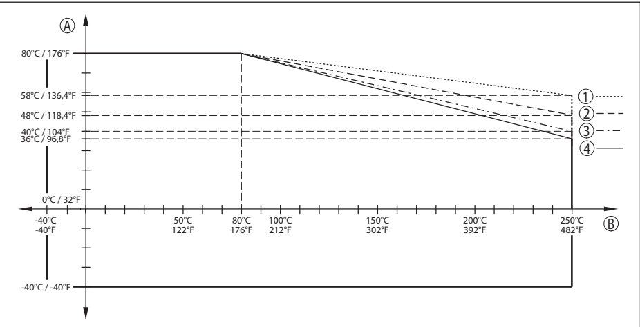
Fig. 78: Derating température ambiante, bride avec antenne cône jusqu'à +250 °C (+482 °F)
