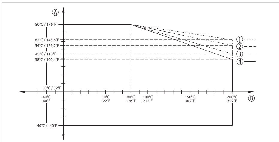
Fig. 70: Derating température ambiante, bride avec système d'antenne encapsulé jusqu'à +200 °C (+392 °F)
