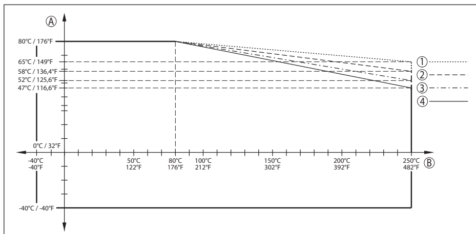
Fig. 74: Derating température ambiante, bride avec antenne lentille jusqu'à +250 °C (+482 °F)
