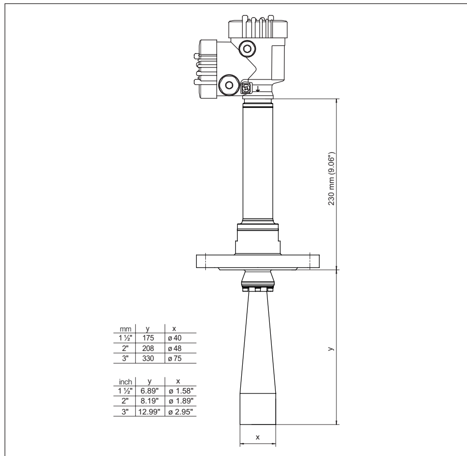
Fig. 90: VEGAPULS 6X, bride avec antenne cône version 450 °C
