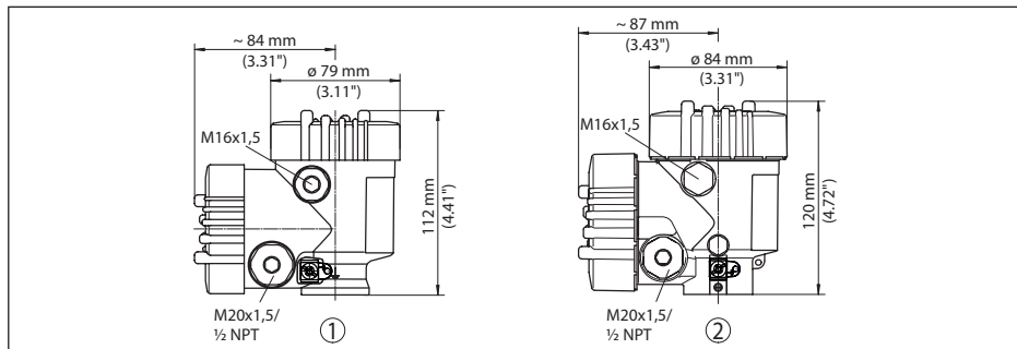
Fig. 79: VEGAPULS 6X ; avec module de réglage et d'affichage intégré, la hauteur du boîtier augmente de 9 mm (0.35 in)
