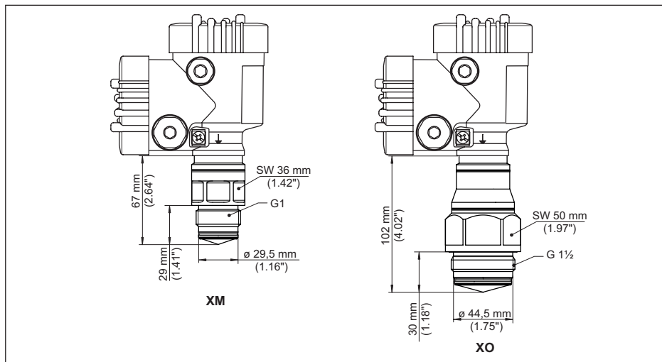
Fig. 93: VEGAPULS 6X, filetage pour adaptateur hygiénique
