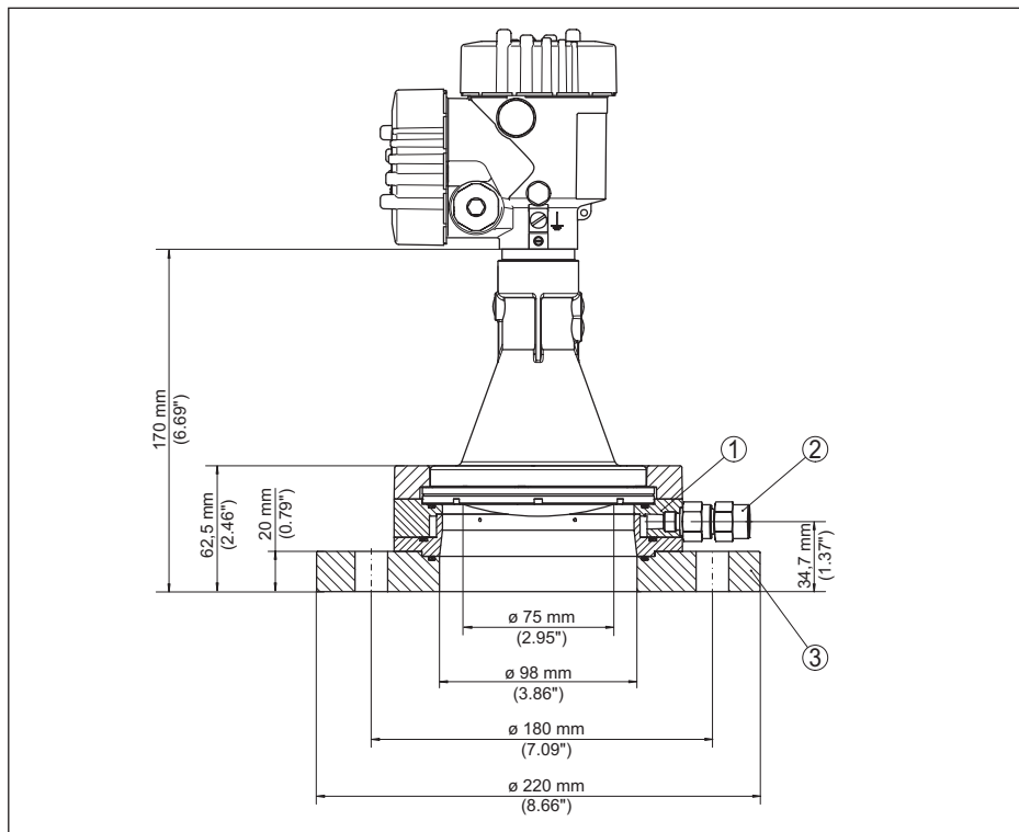
Fig. 83: VEGAPULS 6X, bride d'adaptation et prise d'air de purge DN 100 PN 6
