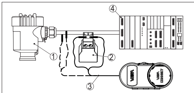
Fig. 58: Raccordement du PC à la ligne signal via HART
