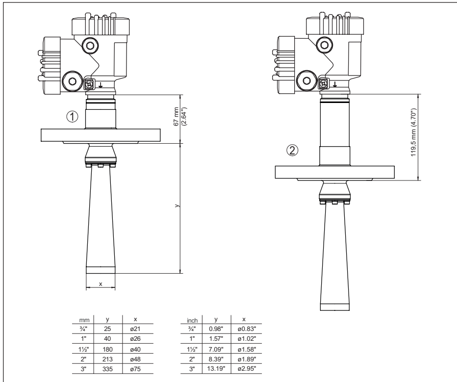
Fig. 88: VEGAPULS 6X, bride avec antenne cône jusqu'à +150 °C (+302 °F)/+250 °C (+482 °F)
