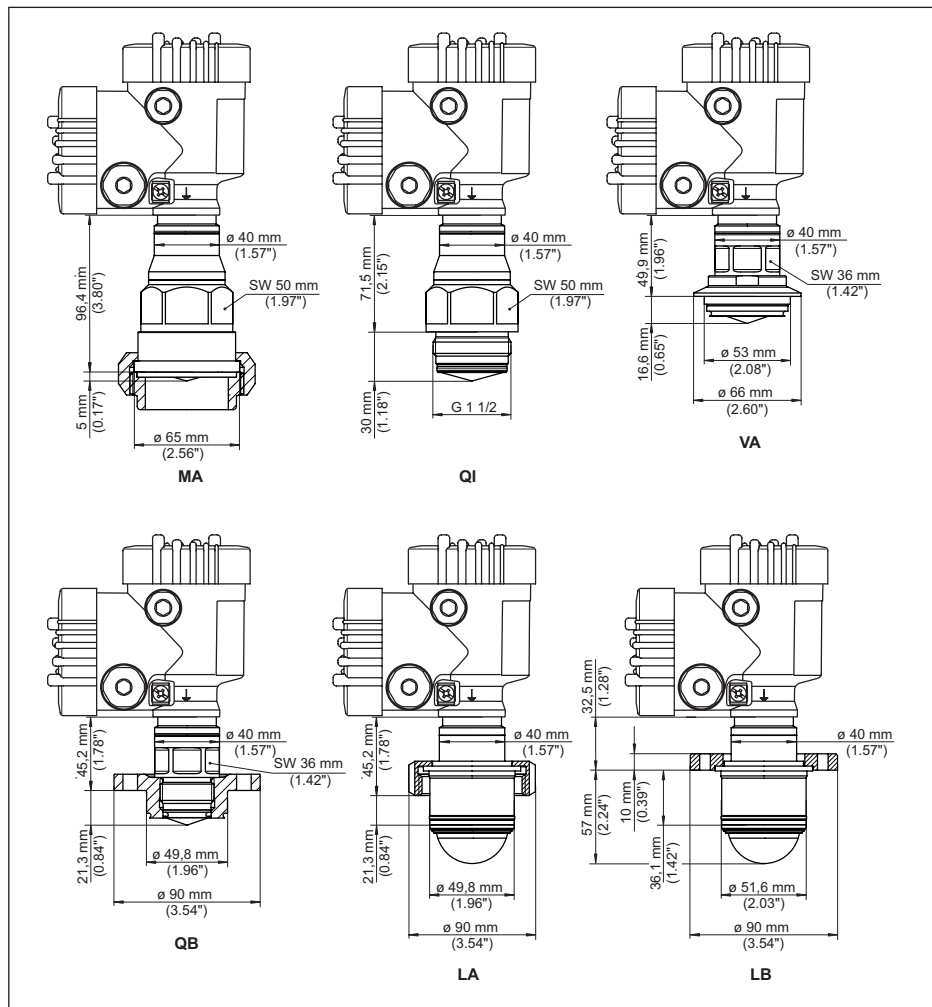
Fig. 95: VEGAPULS 6X, raccord aseptique
