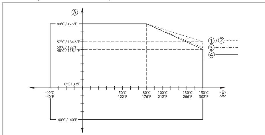
Fig. 68: Derating température ambiante, bride avec système d'antenne encapsulé jusqu'à +150 °C (+302 °F)
