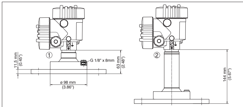
Fig. 96: VEGAPULS 6X, bride avec antenne lentille (épaisseur de la bride cf. schéma, cote de la bride selon DIN, ASME, JIS)
