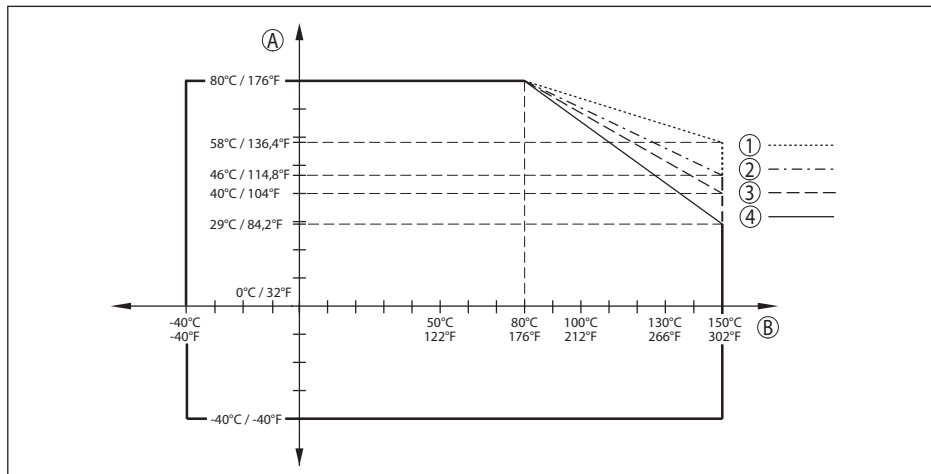
Fig. 76: Derating température ambiante, bride avec antenne cône jusqu'à +150 °C (+302 °F)
