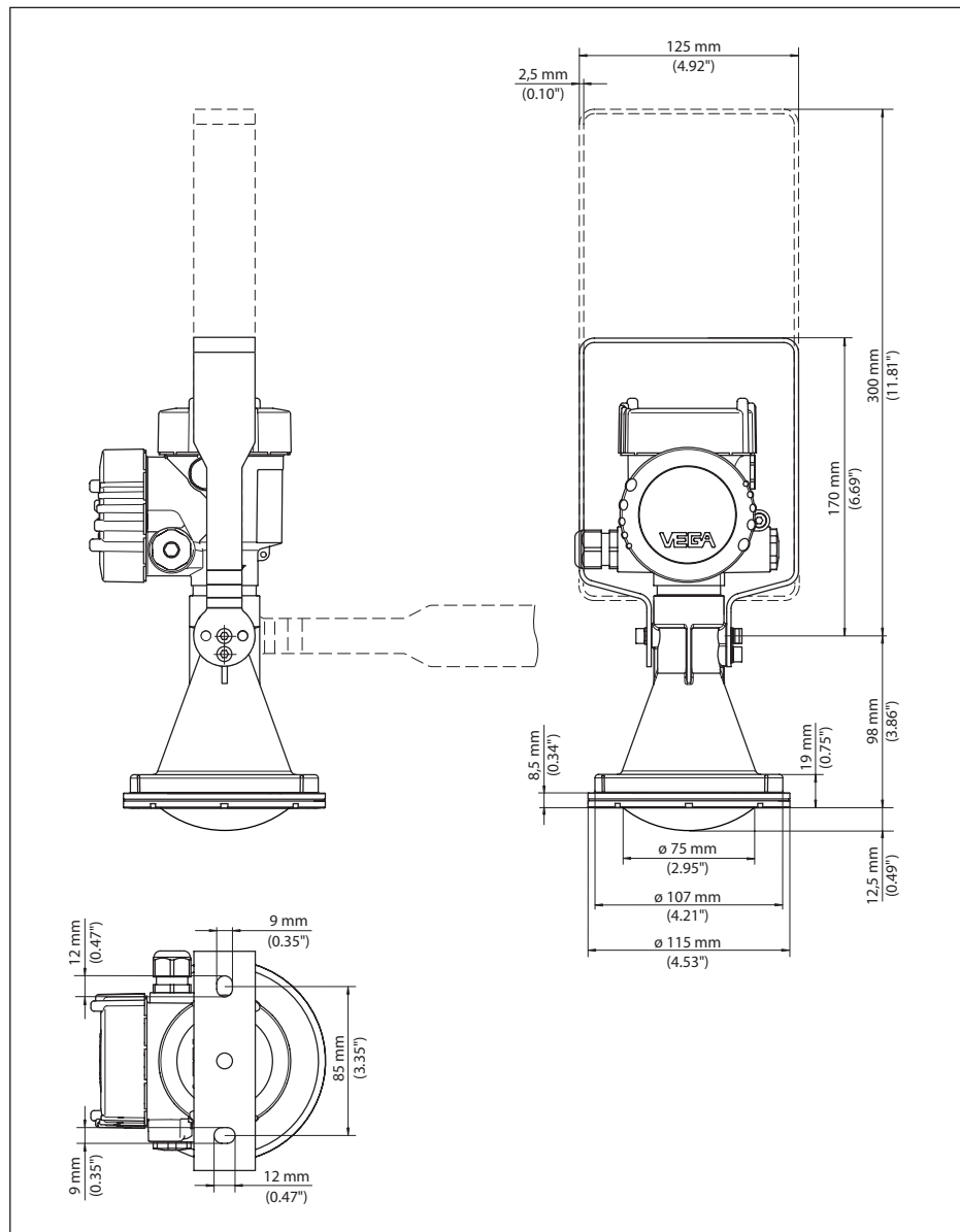
Fig. 84: VEGAPULS 6X, antenne cône en plastique, support de montage en 170 ou 300 mm de longueur
