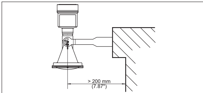
Fig. 11: Montage mural horizontal via l'étrier de montage avec une longueur de 170 mm
