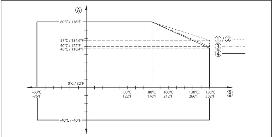
插图. 70: 环境温度降额, 带塑料天线系统的法兰 -60 ... +150 °C (-76 ... +302 °F)
