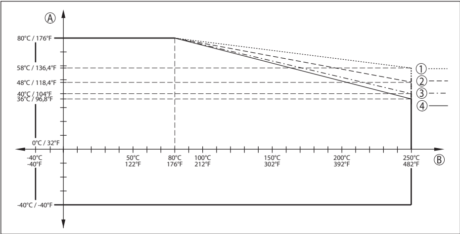
插图. 79: 环境温度降额，带喇叭口天线的法兰，至 +250 °C (+482 °F)
