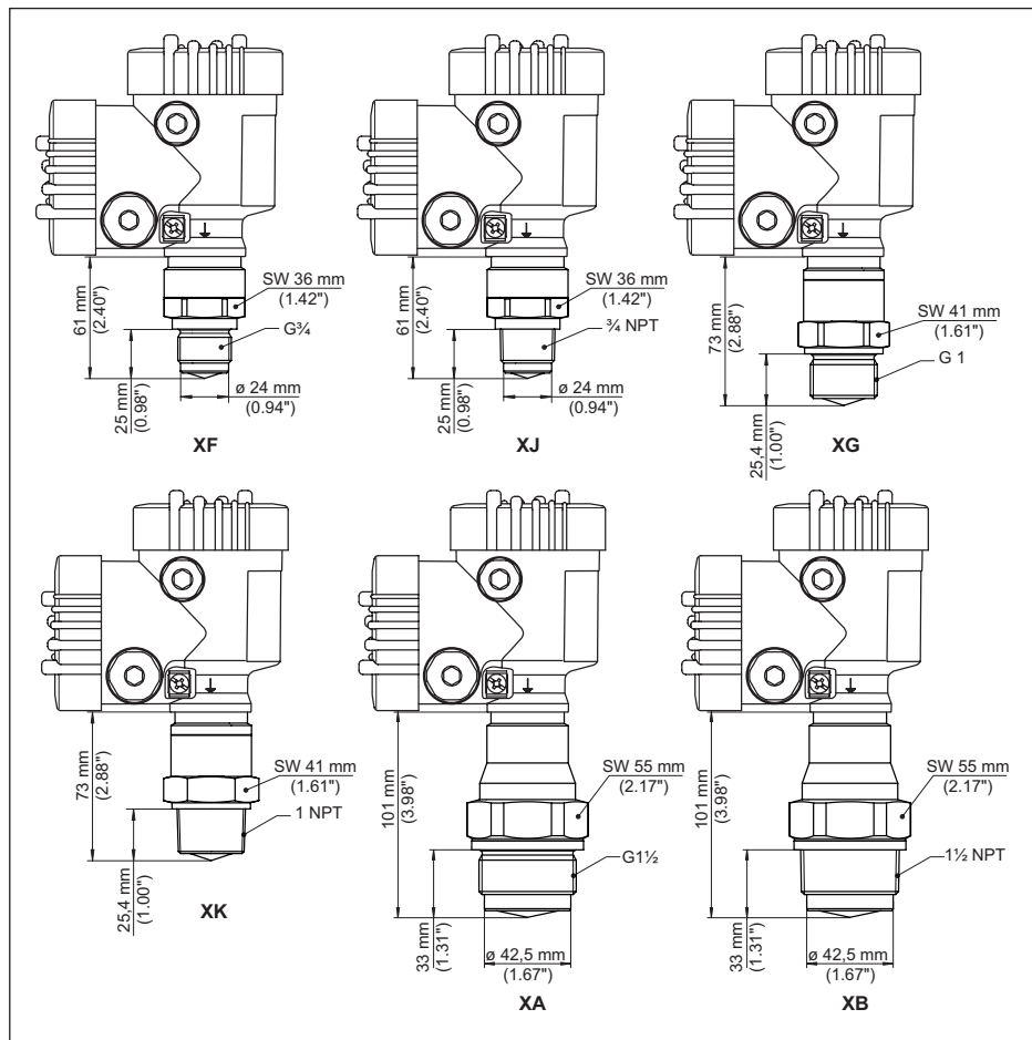
插图. 87: VEGAPULS 6X, 带有内置天线系统的螺纹, 至 +150 °C (+302 °F)
