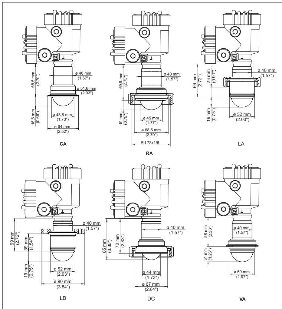
插图: 95: VEGAPULS 6X, 卫生型接口
