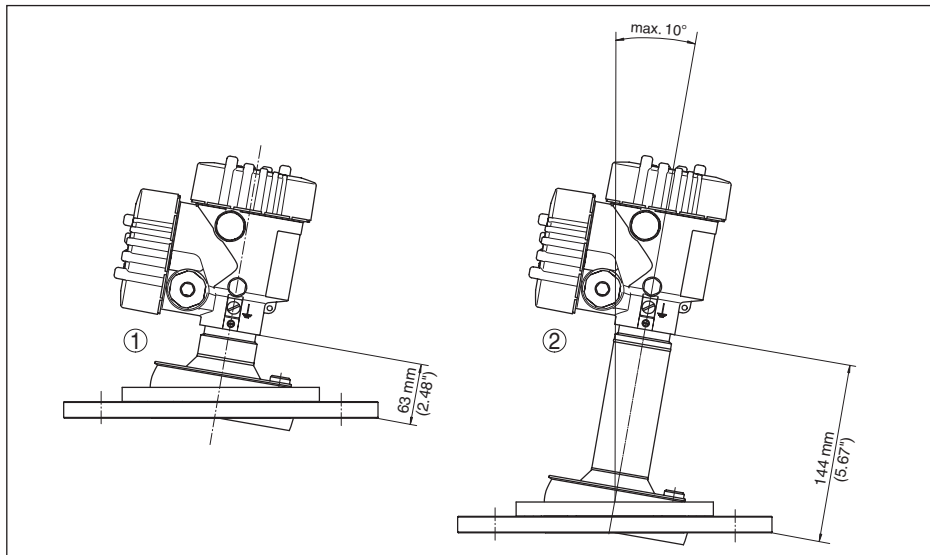
插图. 99: VEGAPULS 6X, 带有透镜天线和万向节的法兰
