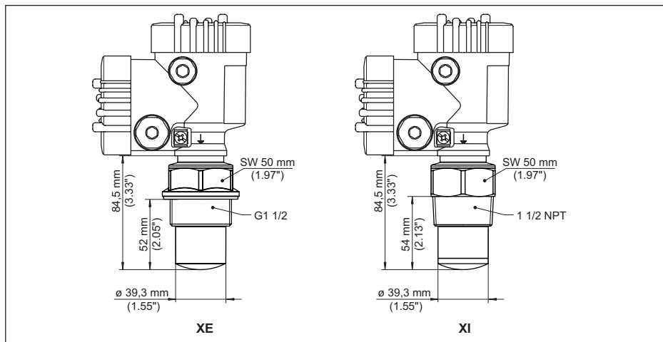
插图. 86: VEGAPULS 6X, 带有内置天线系统的螺纹, 至 +80 °C (+176 °F)
