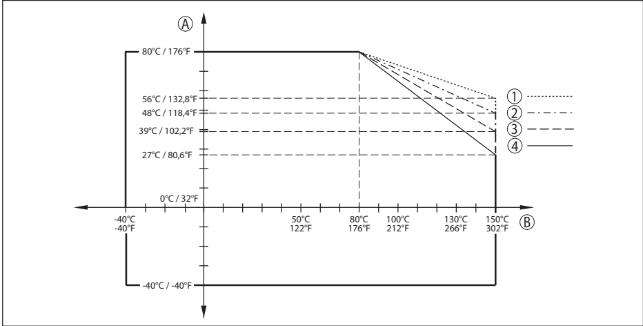
插图. 76: Derating Umgebungstemperatur, Hygieneanschluss bis +150 °C (+302 °F)
