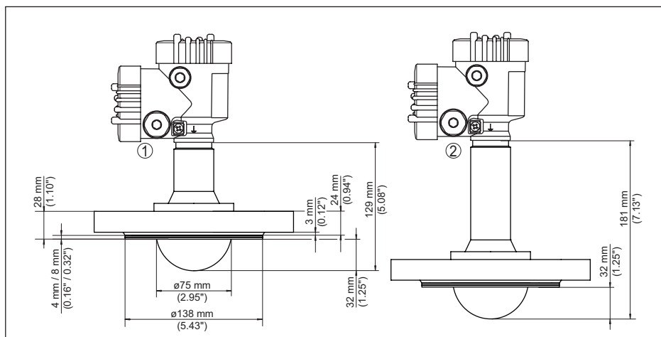
插图 93: VEGAPULS 6X, 封装天线系统 DN 80 PN 40
