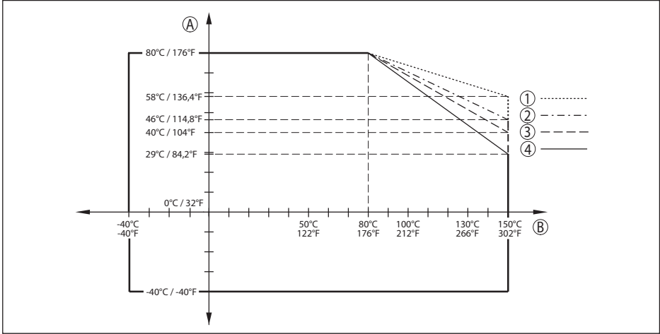
插图. 66: 环境温度降额, 带内置天线系统的螺纹, 至 +150 °C (+302 °F)
