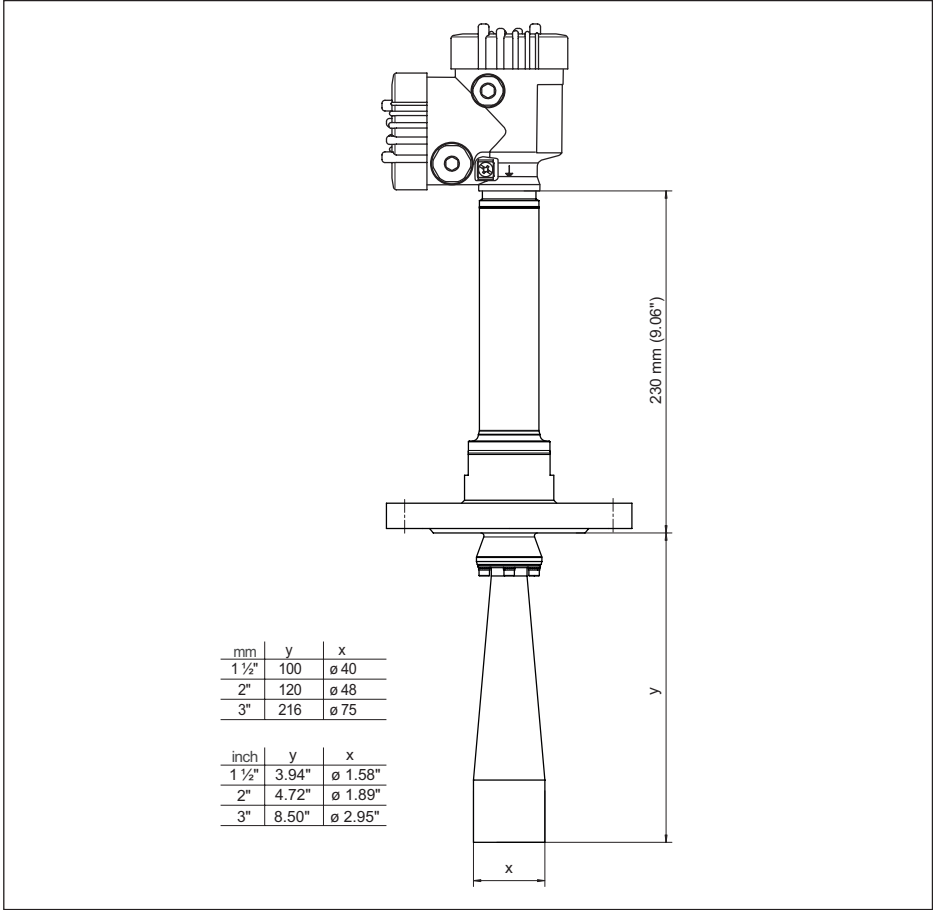
插图. 91: VEGAPULS 6X, 带有号角天线的法兰, 450 °C 型
