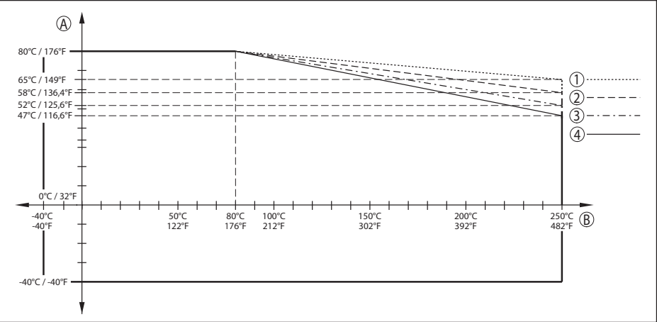
插图. 75: 环境温度降额, 带透镜天线的法兰, 至 +250 °C (+482 °F)
