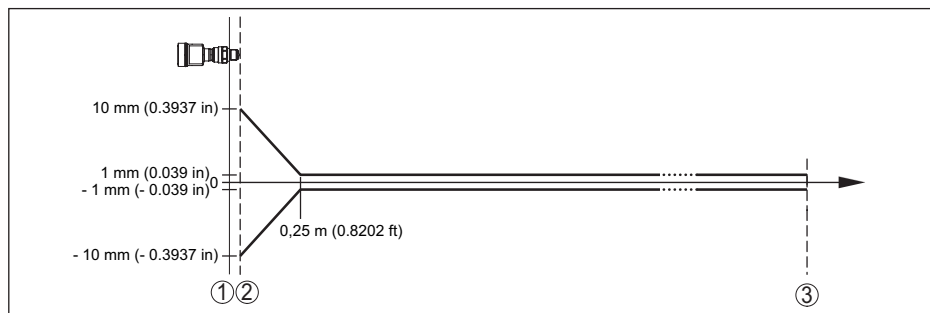
插图 64: 基准条件下的测量误差 (以带有内置天线系统的螺纹为例, 相应地适用于所有版本) 26)
