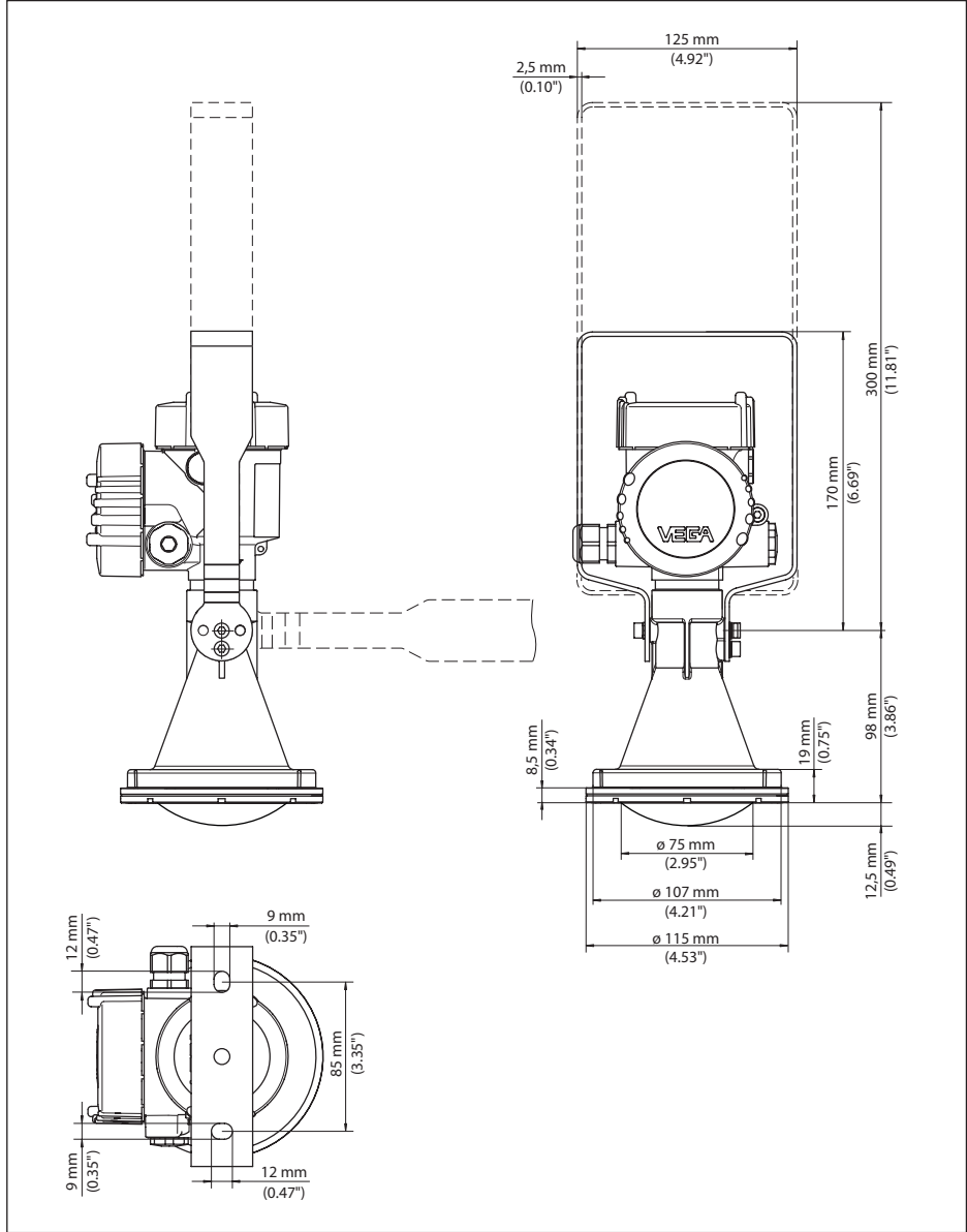
插图. 85: VEGAPULS 6X, 塑料号角天线, 龙门框, 长度为 170 或 300 mm
