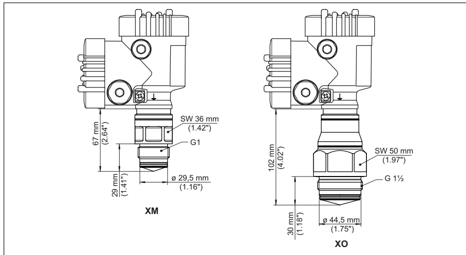
插图. 94: VEGAPULS 6X，用于卫生型适配器的螺纹
