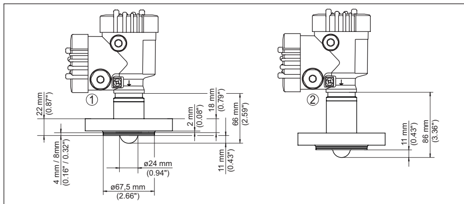
插图 92: VEGAPULS 6X, 封装天线系统 DN 25 PN 40
