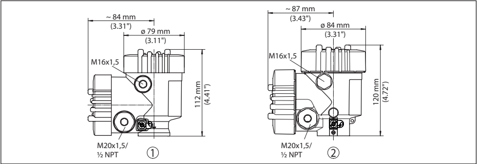
插图. 80: VEGAPULS 6X；带内装的显示和调整模块，能将壳体高度增加 9 mm (0.35 in)
