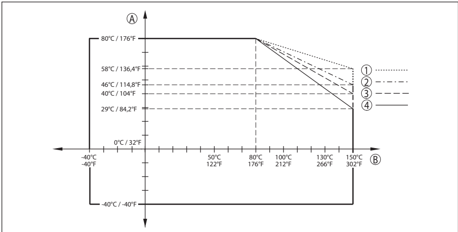
插图. 77: 环境温度降额, 带喇叭口天线的法兰, 至 +150 °C (+302 °F)
