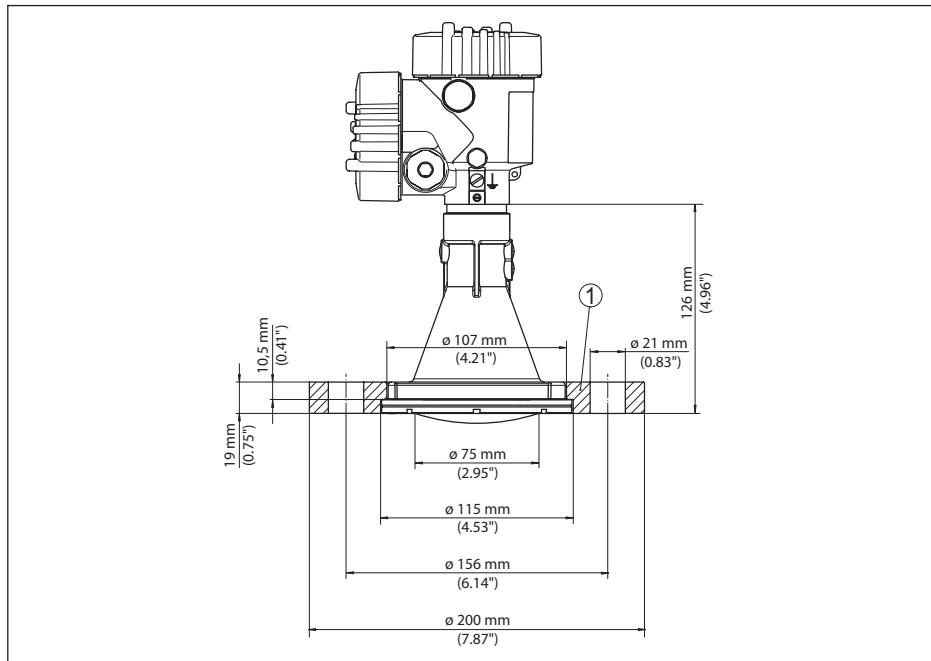
插图. 81: VEGAPULS 6X 带有锁紧法兰, 适用于法兰 3" 150 lbs, DN 80 PN 16
