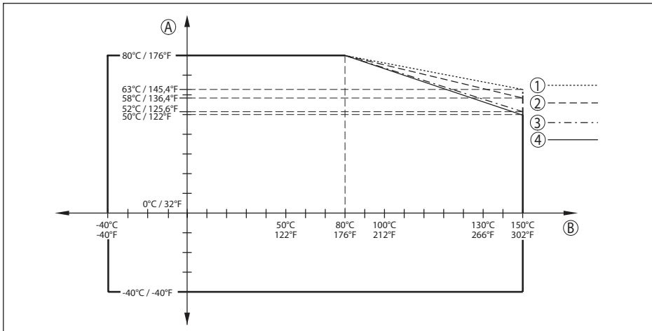
插图. 73: 环境温度降额, 带透镜天线的法兰, 至 +150 °C (+302 °F)
