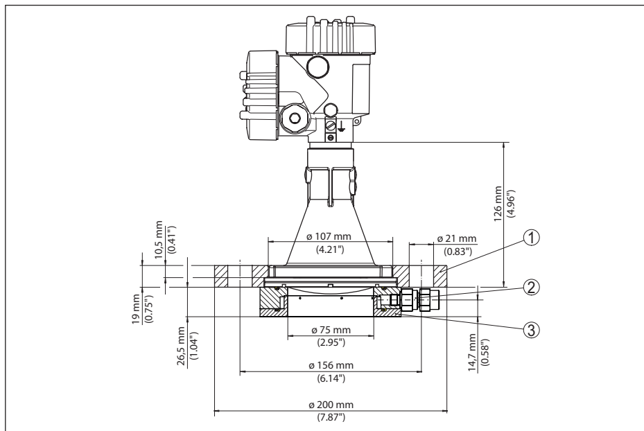
插图. 82: VEGAPULS 6X, 带有锁紧法兰和吹气接口, 适用于 3" 150 lbs, DN 80 PN 16
