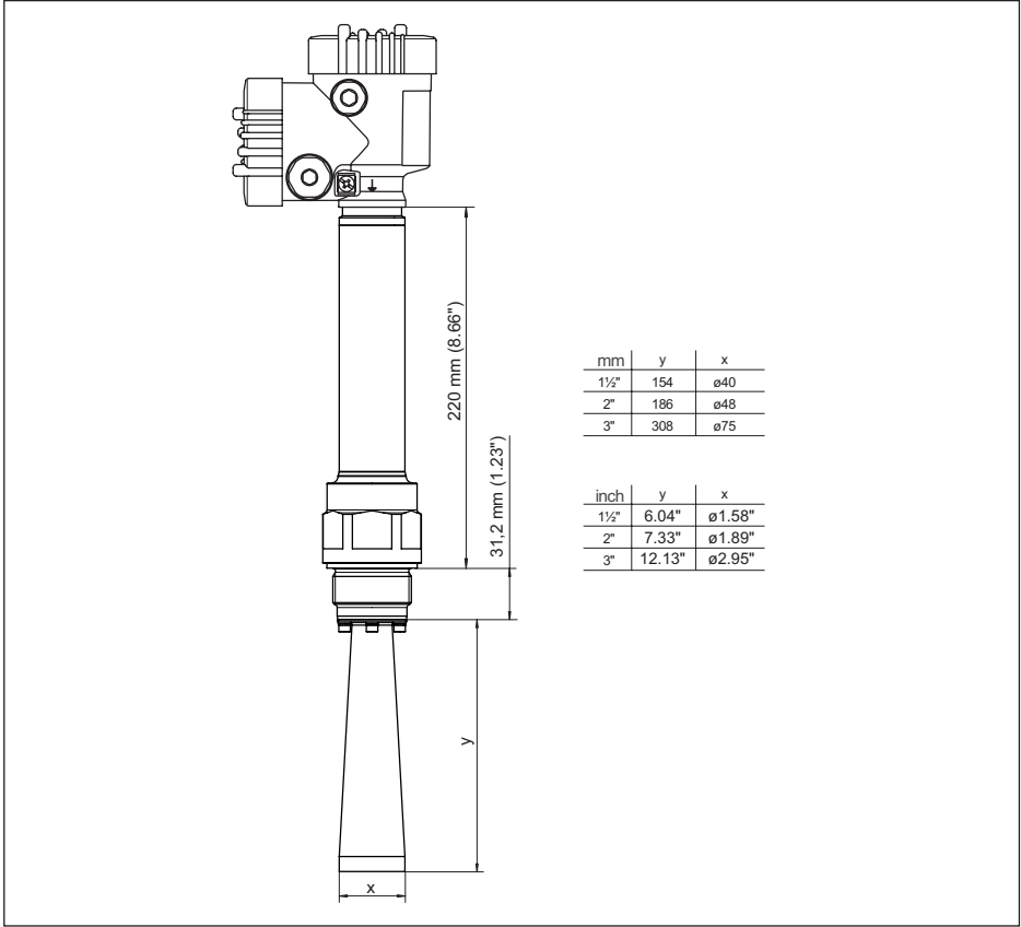
插图. 90: VEGAPULS 6X, 带有号角天线的螺纹, 450 °C 型
