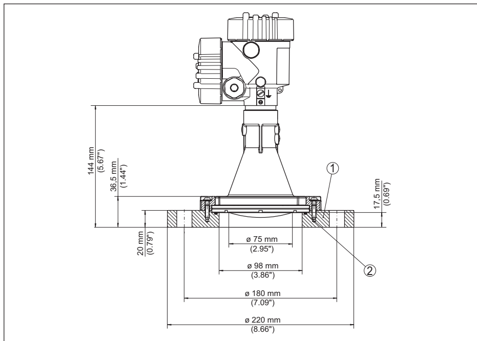
插图. 83: VEGAPULS 6X, 带适配法兰 DN 100 PN 6
