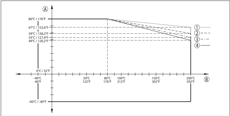
插图. 67: 环境温度降额, 带内置天线系统的螺纹, 至 +200 °C (+392 °F)
