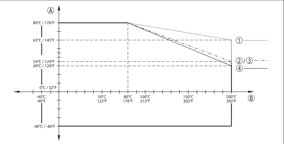
插图. 74: 环境温度降额, 带透镜天线的法兰, 至 +200 °C (+392 °F)
