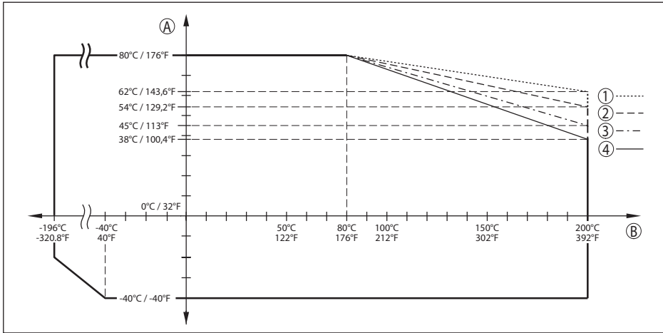
插图. 72: 环境温度降额, 带密封天线系统的法兰 -196 ... +200 °C (-320.8 ... +392 °F)
