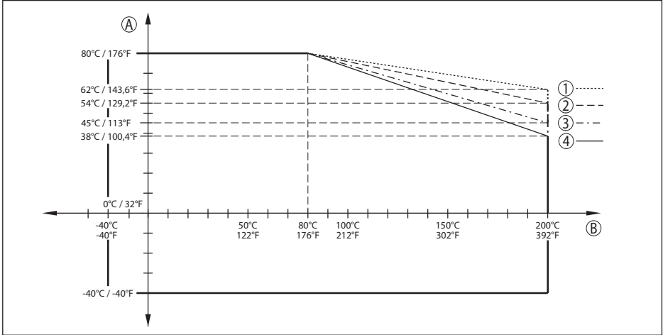
插图. 71: 环境温度降额, 带塑料天线系统的法兰, 至 +200 °C (+392 °F)
