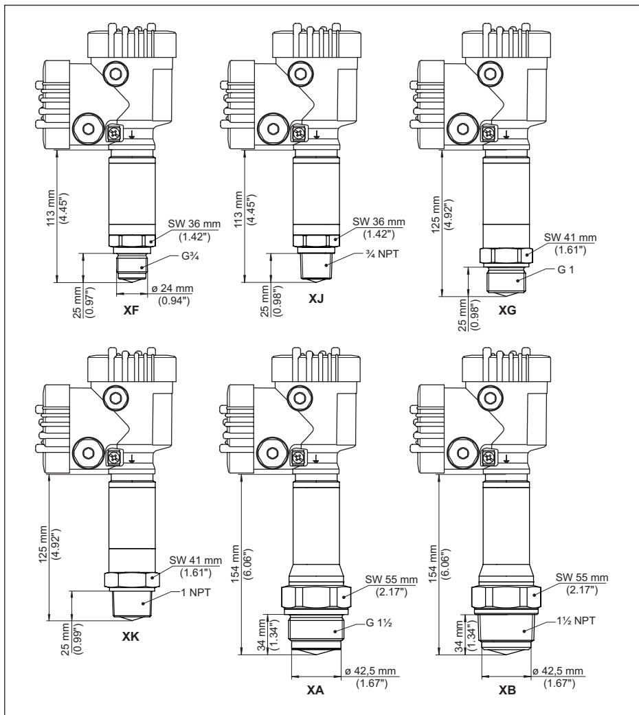
插图 88: VEGAPULS 6X, 带有内置天线系统的螺纹至 +200 °C (+392 °F) 和 +250 °C (+482 °F)
