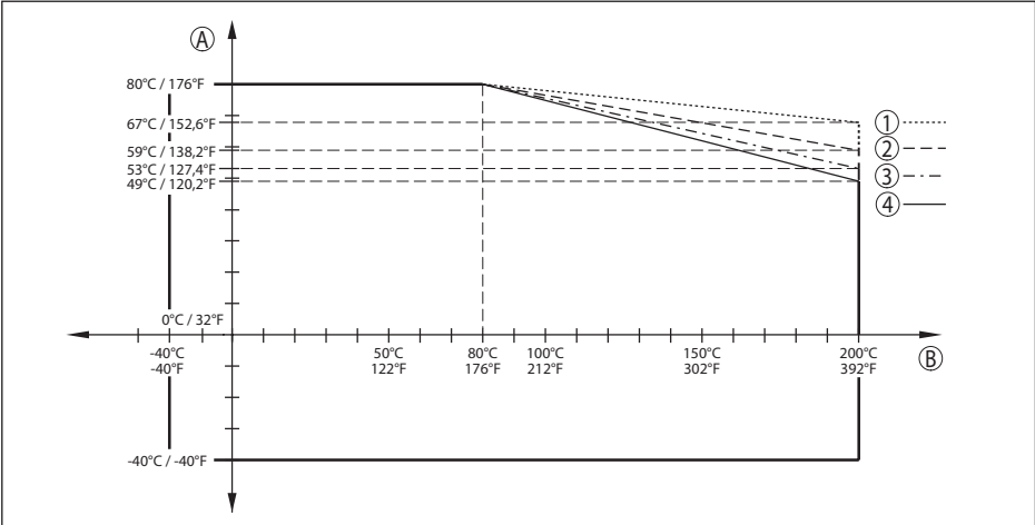
插图. 78: 环境温度降额，带喇叭口天线的法兰，至 +200 °C (+392 °F)
