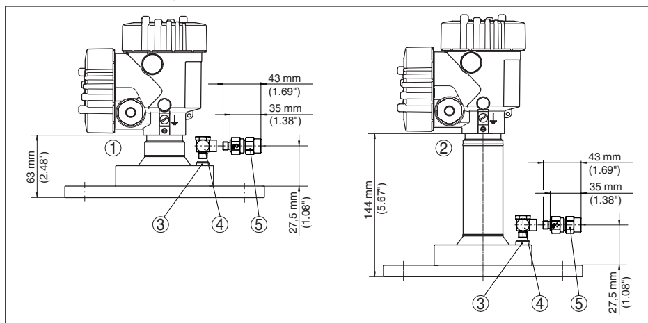
插图 98: VEGAPULS 6X, 带有透镜天线和吹气接口的法兰
