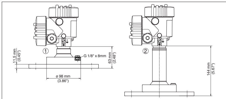
插图 97: VEGAPULS 6X, 带有透镜天线的法兰 (法兰厚度参见图纸, 法兰尺寸根据 DIN, ASME, JIS)
