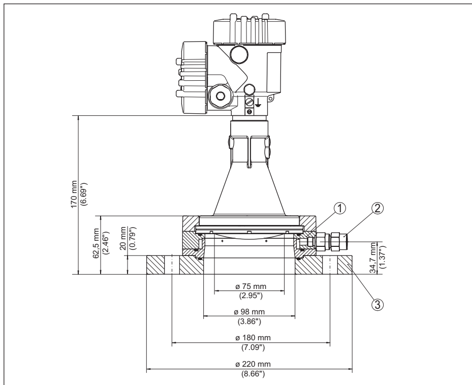
插图. 84: VEGAPULS 6X, 适配法兰和吹气接口 DN 100 PN 6
