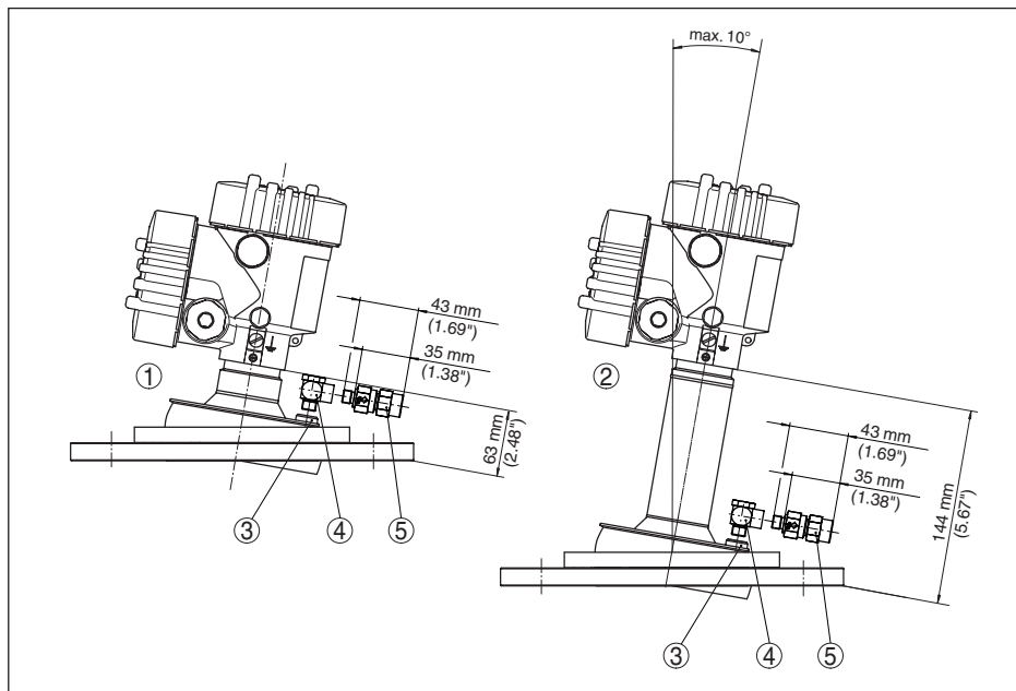
插图. 100: VEGAPULS 6X, 带有透镜天线、万向节和吹气接口的法兰
