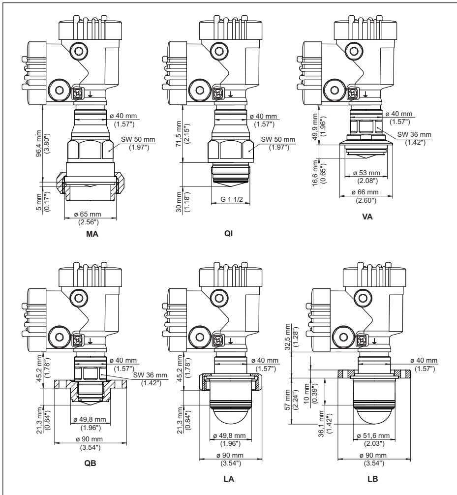
插图 96: VEGAPULS 6X, 卫生型接口
