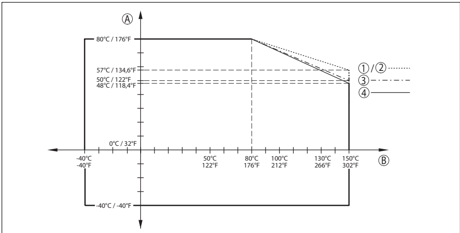
插图. 69: 环境温度降额, 带塑封天线系统的法兰, 至 +150 °C (+302 °F)
