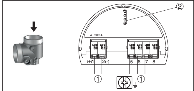
插图. 7: 双腔式外壳的电子部件腔
