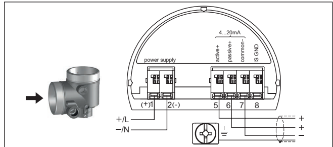
插图. 8: 小电压供电时双腔式外壳的接线腔
