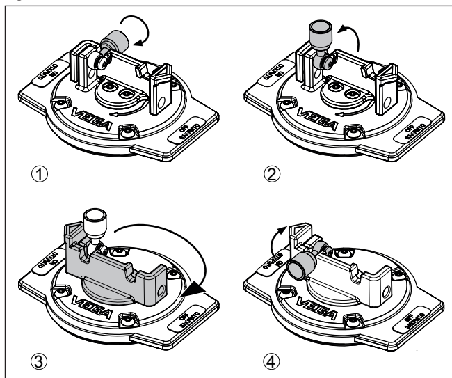
Fig. 16: Conexión de la radiación - VEGASOURCE 85 versión X, C
