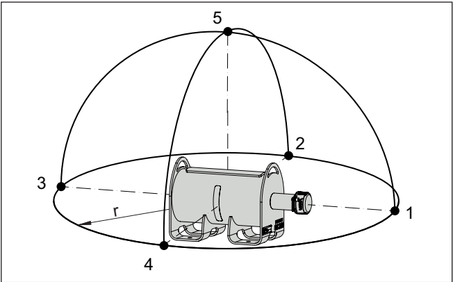
Fig. 21: Puntos de medición para medición de la tasa de dosis local r Distancia al contenedor de protección de fuente radiactiva 1-5 Puntos de medición
