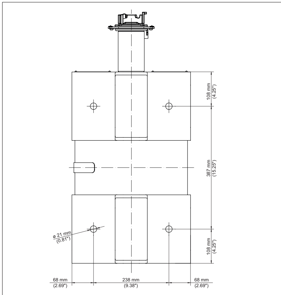
Fig. 26: Placa de montaje con orificios (p. Ej. Versión X, C)
