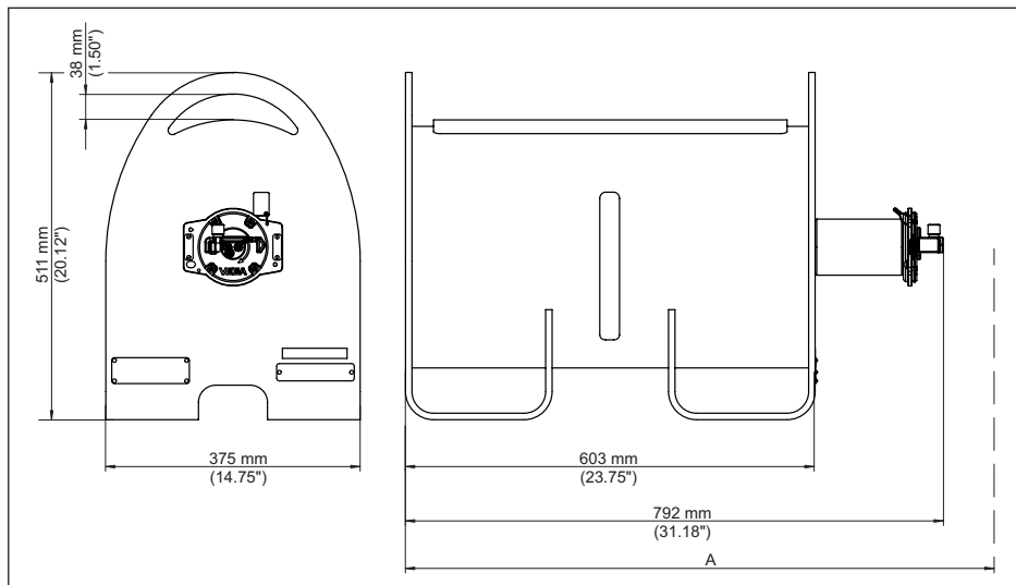
Fig. 24: Contenedor de protección de fuente radiactiva VEGASOURCE 85, versión X, C - Conmutación manual ON/OFF
