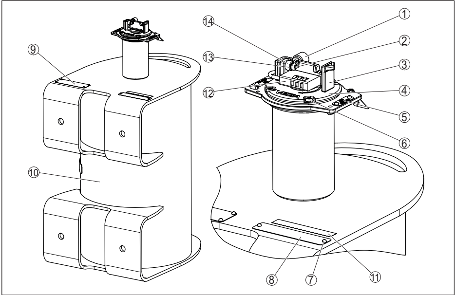
Fig. 23: Materiales VEGASOURCE 85 - versión K, C
