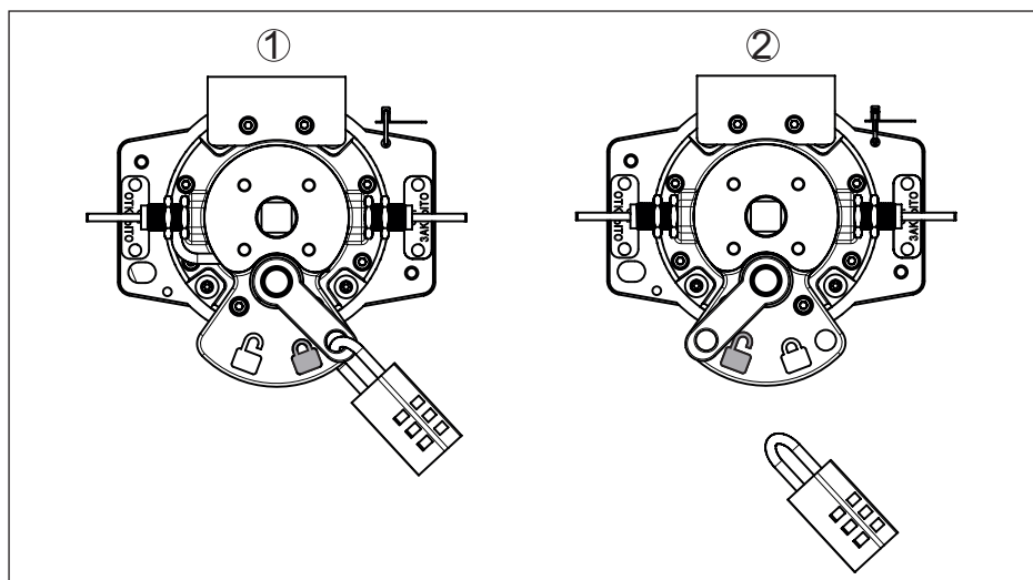
Fig. 18: Affichage de l'état de commutation sur VEGASOURCE 86 - Version B - Commutation MARCHE/ARRÊT pneumatique
