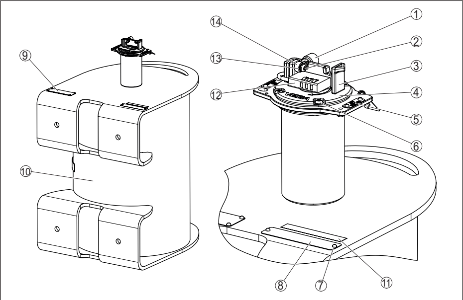
Fig. 21: Matériaux VEGASOURCE 86 - version X, C
