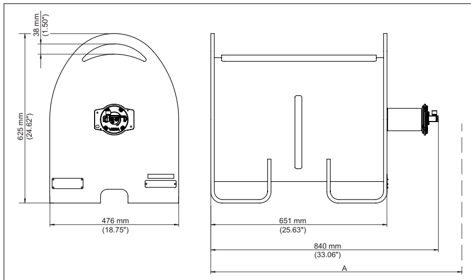
Fig. 22: Conteneur blindé VEGASOURCE 86, version X, C - commutation MARCHE/ARRÊT manuelle
