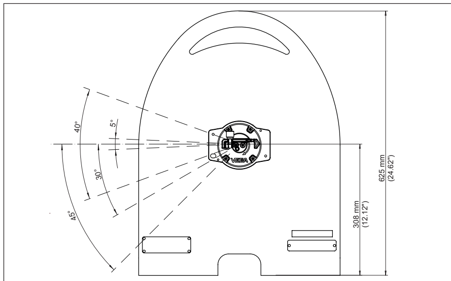
Fig. 25: Canal de sortie des rayonnements (par ex. version X, C)
