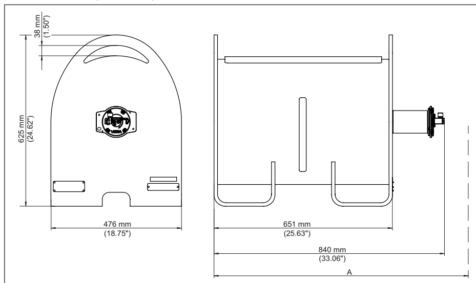
Fig. 24: Conteneur blindé VEGASOURCE 86, version X, C - commutation MARCHE/ARRÊT manuelle
