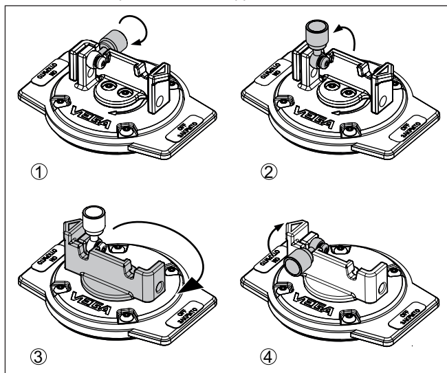
Fig. 16: Mise en marche du rayonnement - VEGASOURCE 86 Version X, C
