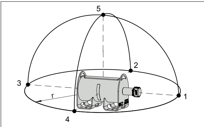
Fig. 21: Points de mesure pour la mesure de débit de dose locale r Distance par rapport au conteneur blindé 1-5 Points de mesure
