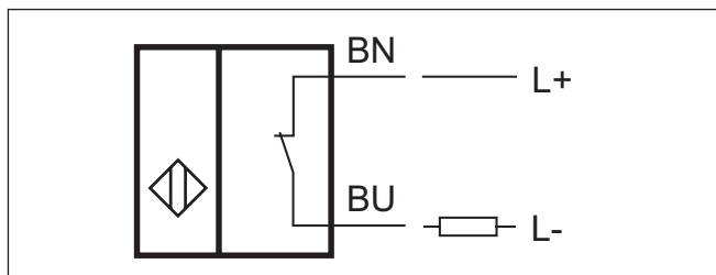
Fig. 12: Esquema de conexión - Interruptor de posición ON/OFF
