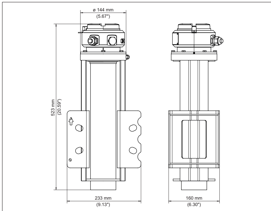
Fig. 27: Modulador gamma para la medición continua, incluso en caso de radiación externa
