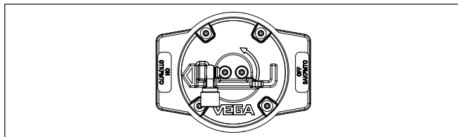
Fig. 17: Radiación "ON" - VEGASOURCE 86 Versión X, C
