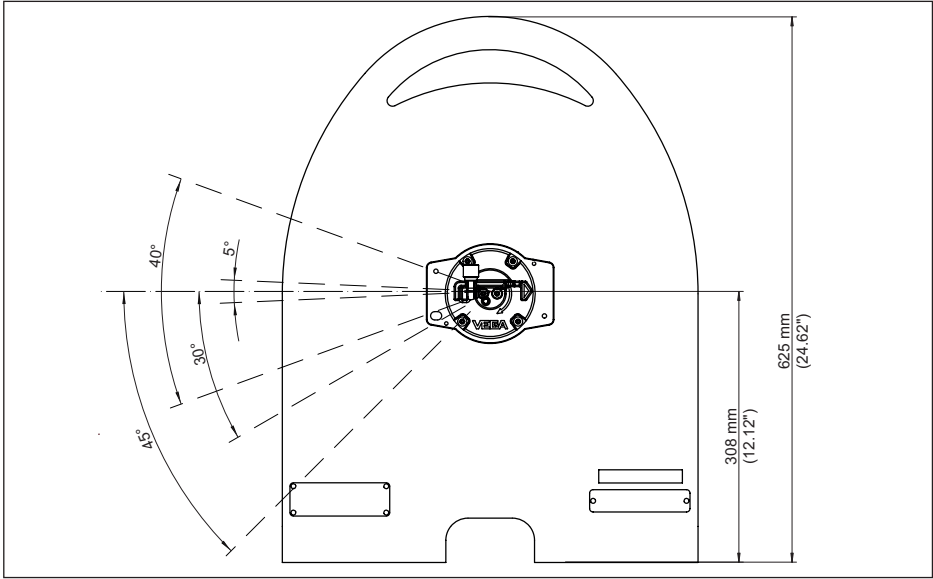
Fig. 25: Canal de salida de radiación (p. Ej. versión X, C)
