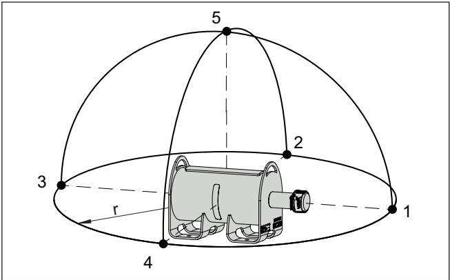
Fig. 21: Puntos de medición para medición de la tasa de dosis local r Distancia al contenedor de protección de fuente radiactiva 1-5 Puntos de medición
