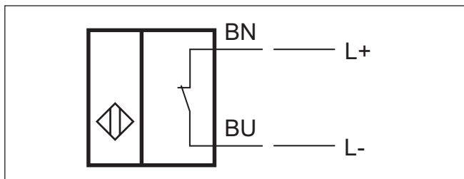
Fig. 15: Esquema de conexión - Interruptor de posición ON/OFF - NAMUR
