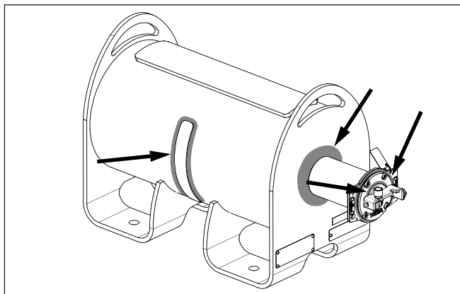
Fig. 22: Superficies de limpieza para la prueba de contaminación - Versión X, C
