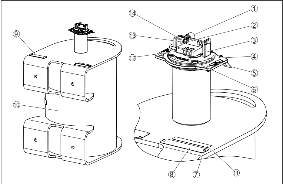
Fig. 23: Materiales VEGASOURCE 86 - versión K, C
