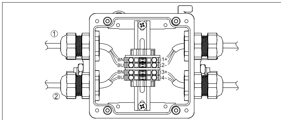
Fig. 14: Caja de bornes de conexión de los interruptores de posición ON/OFF
