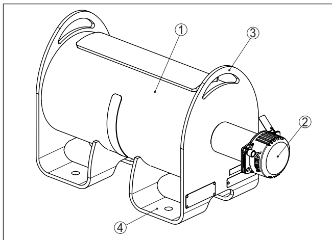
Fig. 4: Contenedor de protección de fuente radiactiva VEGASOURCE 86
