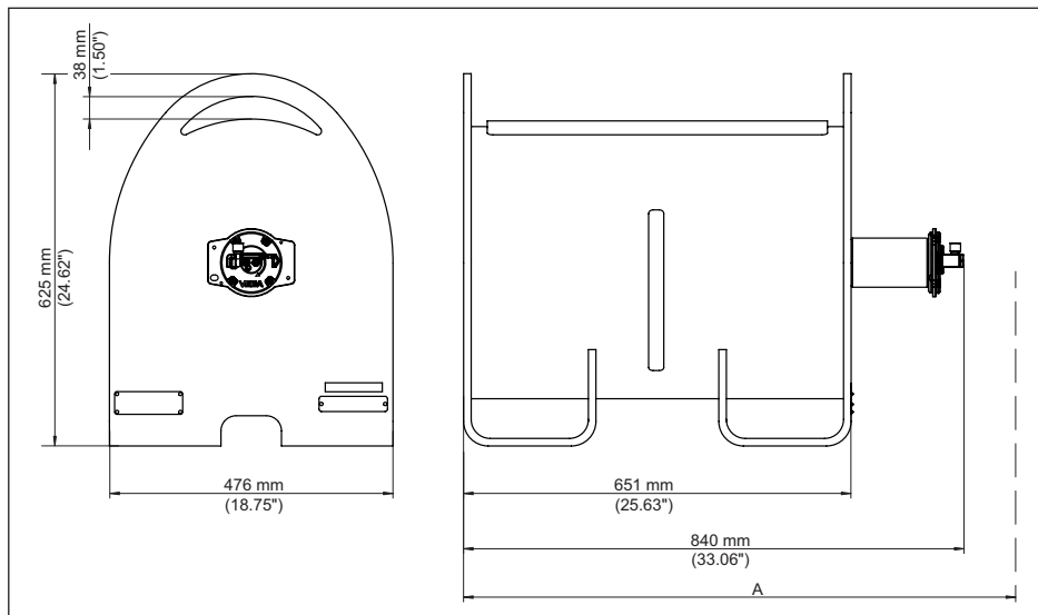
Fig. 24: Contenedor de protección de fuente radiactiva VEGASOURCE 86, versión X, C - Conmutación manual ON/OFF
