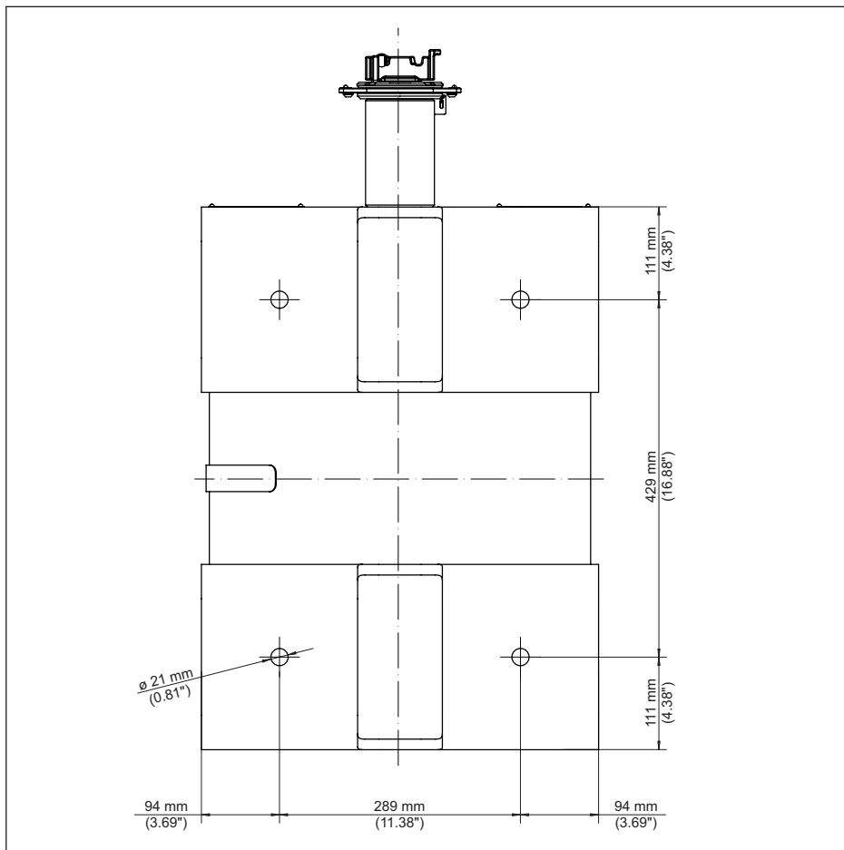
Fig. 26: Placa de montaje con orificios (p. Ej. Versión X, C)
