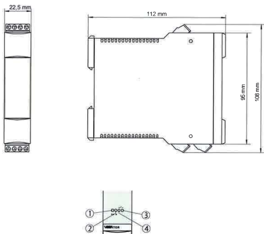
VEGATOR 632. CA
