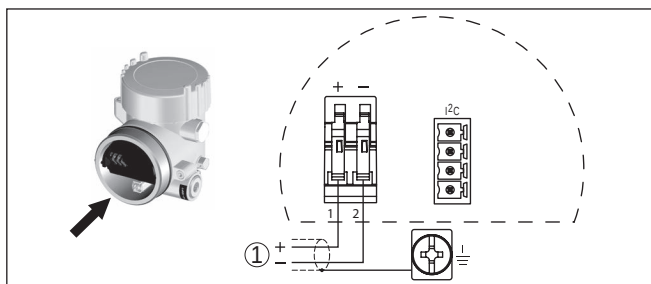
Fig. 27: Aansluitschema - tweekamerbehuizing
