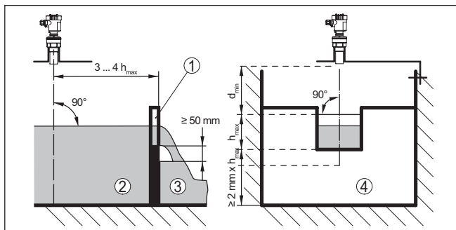
Fig. 18: Flowmeting met rechthoekig overstortschot: d_{\min} = blokaafstand van de sensor (zie hoofdstuk "Technische gegevens"); h_{\max} = max. vulhoogte rechthoekige overstortschot
