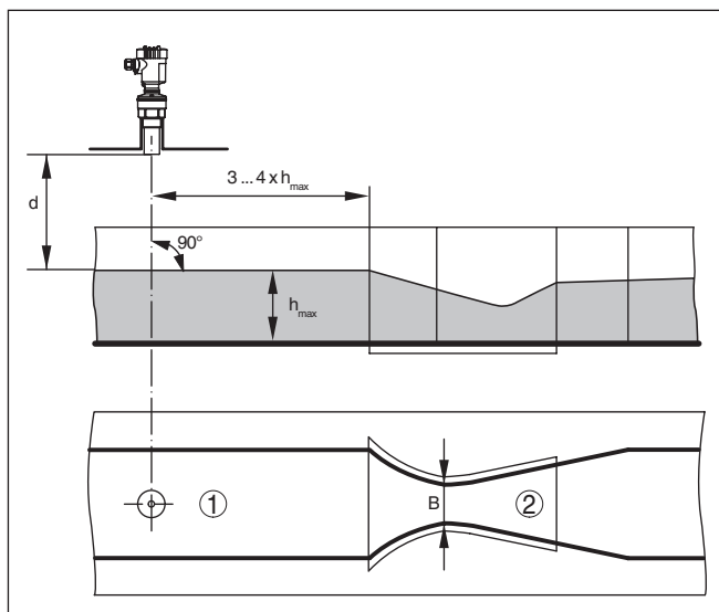
Fig. 19: Flowmeting met Khafagi-venturigoot: d = blokafstand van de sensor; h_{max} = max. vulgraad van de goot; B = grootste insnoering van de goot
