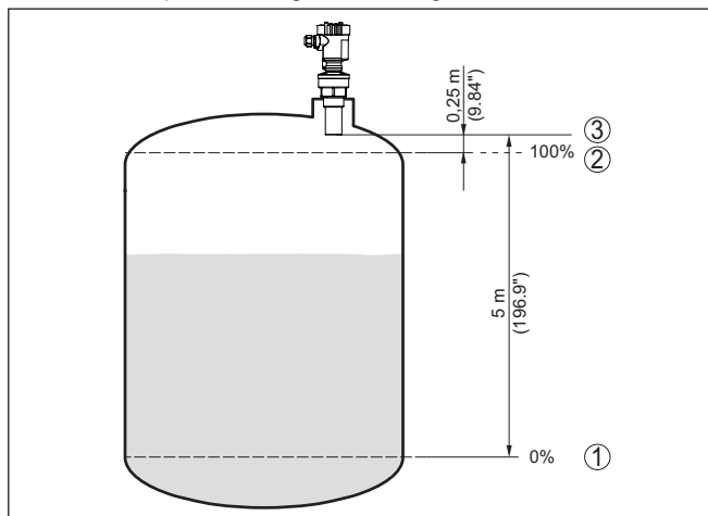
Fig. 31: Parametreervoorbeeld min.-/max.-inregeling
