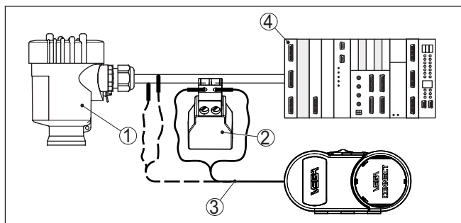
Fig. 34: Aansluiting van de PC via HART op de signaalkabel
