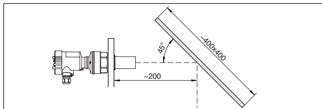
Fig. 13: Spiegel
