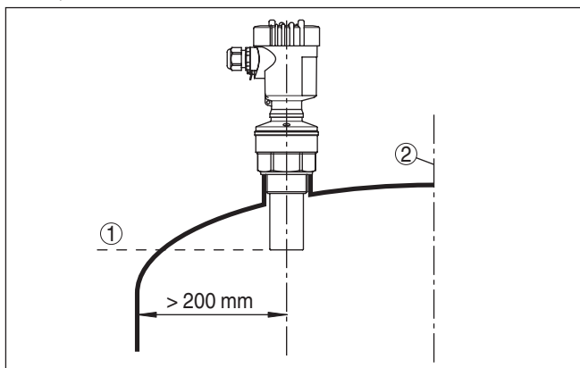
Fig. 8: Montage op ronde tankdaken
