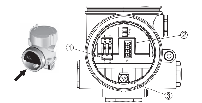
Fig. 26: Aansluitruimte - tweekamerbehuizing
