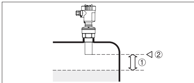
Fig. 6: Blokafstand tot max. vulhoogte
