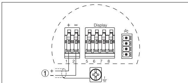
Fig. 23: Aansluitschema - eenkamerbehuizing
