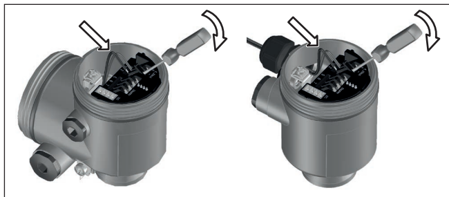
Figura 17: Operazioni di collegamento 6 e 7
