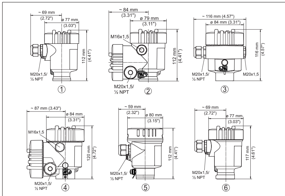
Figura 35: Differenti custodie con grado di protezione IP66/IP68 (0,2 bar), (con tastierino di taratura con display incorporato l'altezza della custodia aumenta di 9 mm/0.35 in, in caso di custodie di metallo di 18 mm/0.71 in)
