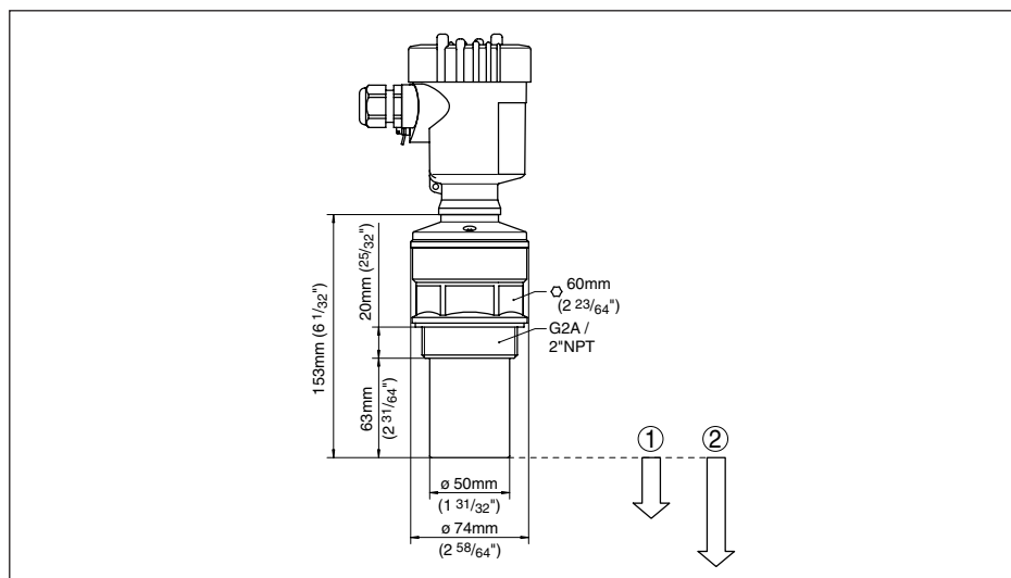
Figura 37: VEGASON 62
