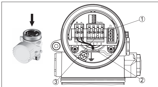
Figura 22: Vano dell'elettronica - custodia a due camere
