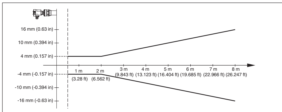
Figura 34: Scostamento di misura VEGASON 62
