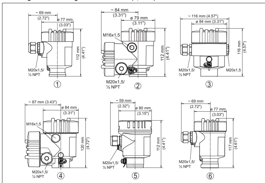
Fig. 34: Huisuitvoeringen in beschermingsklasse IP66/IP68, (0,2 bar), (met ingebouwde display- en bedieningsmodule wordt het huis 9 mm/0,35 in hoger, bij metalen behuizingen 18 mm/0.71 in)
