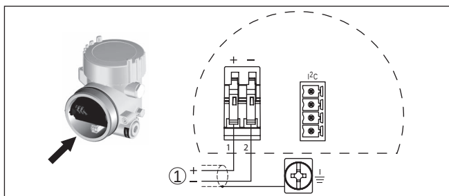
Fig. 22: Aansluitschema - tweekamerbehuizing
