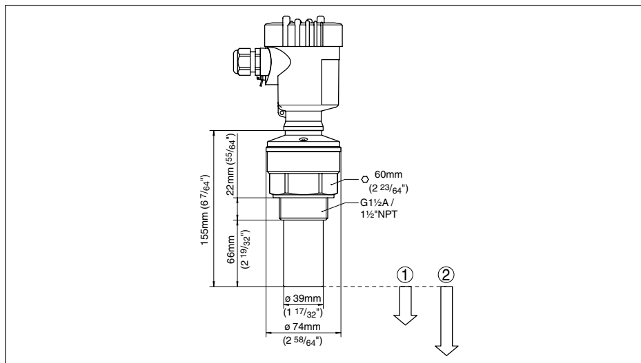
Fig. 36: VEGASON 61
