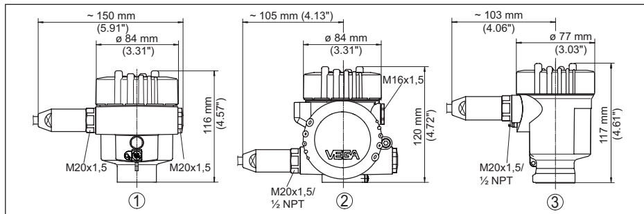
Fig. 35: Huisuitvoeringen in beschermingsklasse IP66/IP68 (1 bar), (met ingebouwde display- en bedieningsmodule wordt het huis 18 mm/0.71 in hoger)
