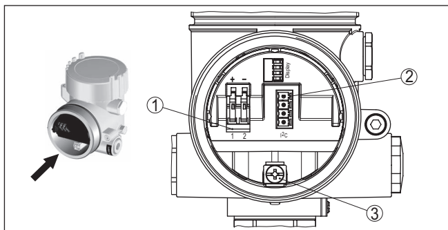
Fig. 21: Aansluitruimte - tweekamerbehuizing
