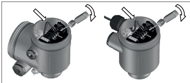
Fig. 15: Aansluitstappen 6 en 7
