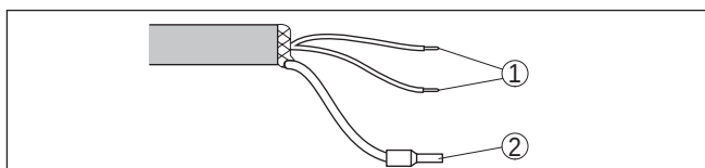
Fig. 23: Aderbezetting aansluitkabel
