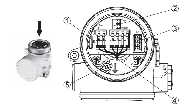
Fig. 20: Elektronicar ruimte - tweekamerbehuizing
