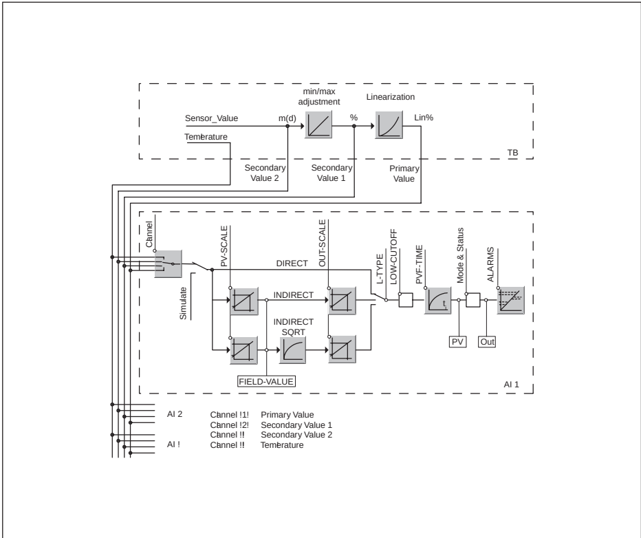
Fig. 32: Meetwaardeverwerking VEGASON 61
