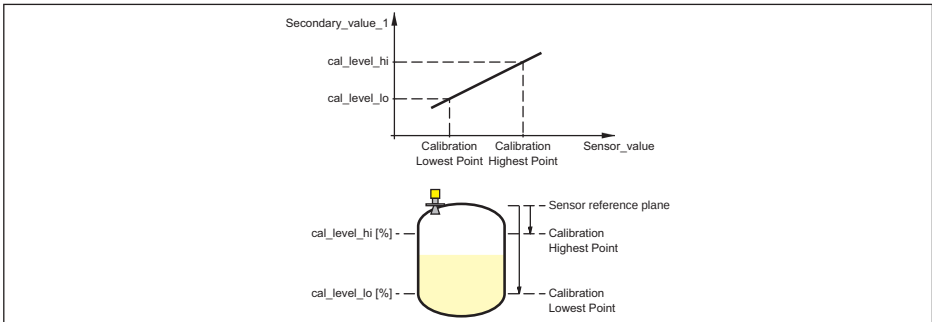
Fig. 33: Inregeling VEGASON 61
