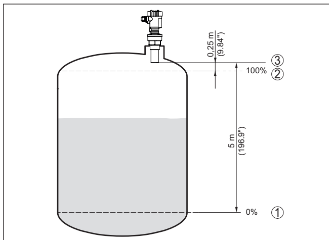
Fig. 27: Parametreevoorbeeld min.-/max.-inregeling
