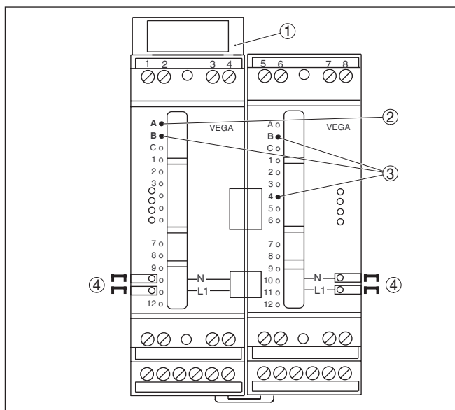
Fig. 2: Klemsokkel VEGAMET 624
