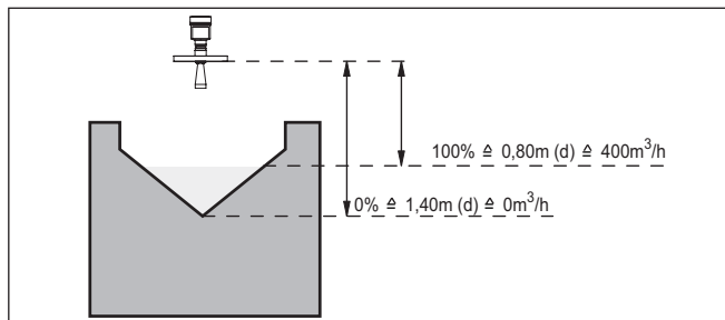
Fig. 14: Inregeling doorstroommeting met driehoekig overstortschot
