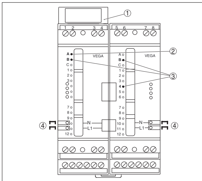
Fig. 2: Klemsokkel VEGAMET 624
