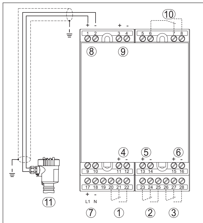
Rys. 3: Schemat przyłączy VEGAMET 624 dla sondy 2-przewodowej
