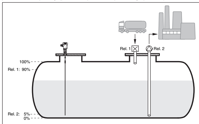
Rys. 11: Przykład pomiaru poziomu napełnienia zbiornika walcowego w pozycji leżącej
