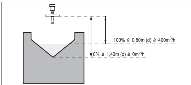
Rys. 14: Kompensacja pomiaru natężenia przepływu z przelewem trójkątnym
