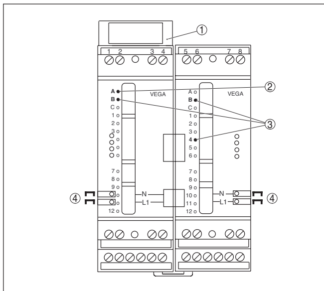
Fig. 2: Klemsokkel VEGAMET 625
