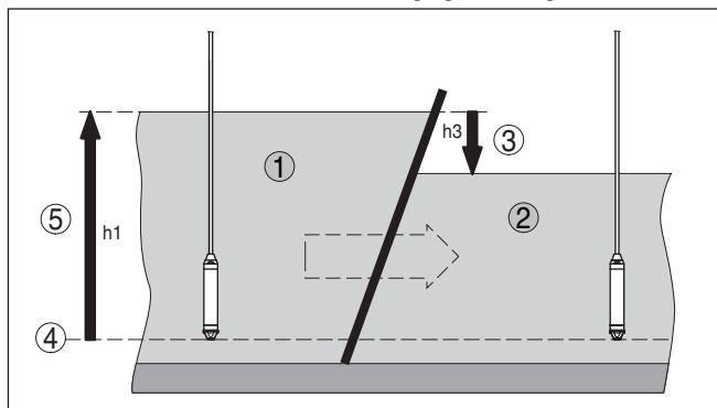
Fig. 12: Verschilmeting roosterbesturing
