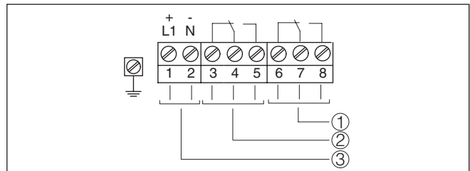
Fig. 9: Esquema de ligações da caixa de uma câmara
