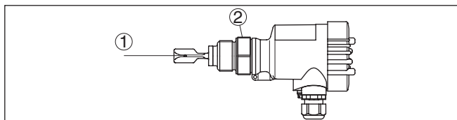
Rys. 4: Montaż poziomy (zalecane położenie montażowe, szczególnie w wypadku mediów o skłonnościach do przyklejania)
