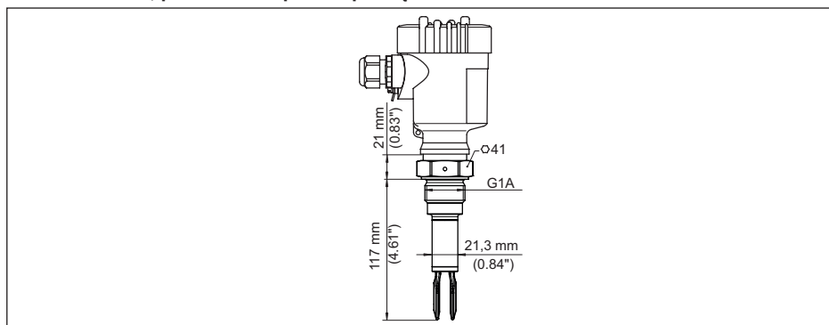
Rys. 20: Przedłużenie punktu przełączenia - do łatwej wymiany VEGASWING 81 lub 81 A
