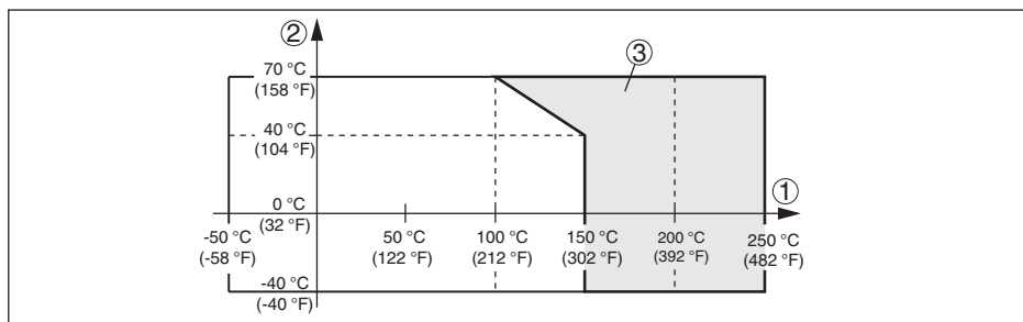
Rys. 14: Temperatura otoczenia - temperatura procesu technologicznego
