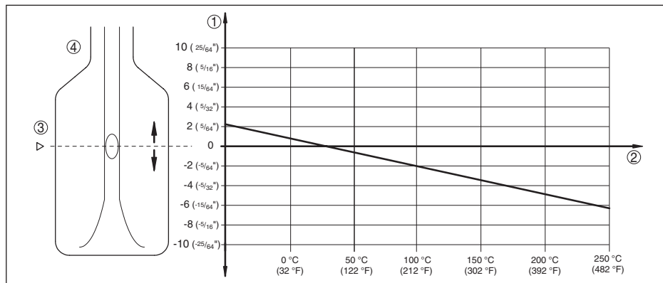
Rys. 11: Wpływ temperatury procesu na punkt przełączenia
