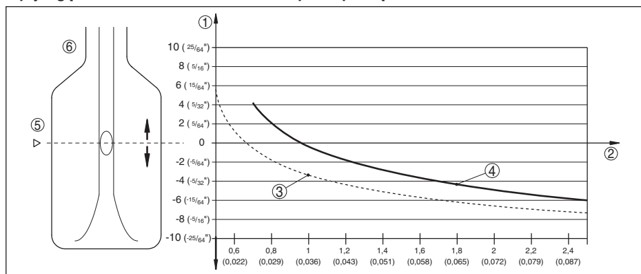
Rys. 12: Wpływ gęstości materiału w zbiorniku na punkt przełączenia
