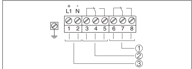
Rys. 9: Schemat przyłączy dla budowy jednokomorowej
