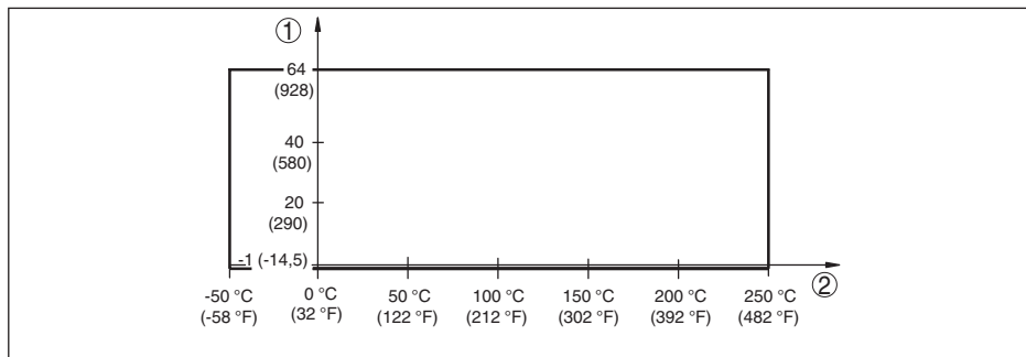
Rys. 15: Temperatura technologiczna - ciśnienie technologiczne przy położeniu przełącznika \geq 0,7 \text{ g/cm}^3 (przełącznik czułości)
