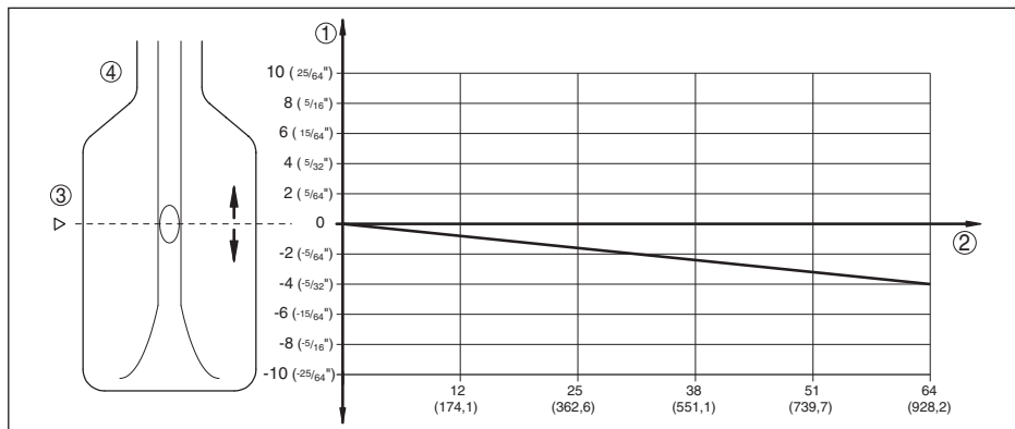
Rys. 13: Wpływ ciśnienia procesu na punkt przełączenia
