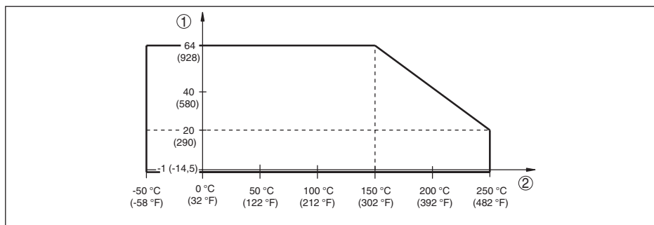
Rys. 16: Temperatura technologiczna - ciśnienie technologiczne przy położeniu przełącznika \geq 0,5 \text{ g/cm}^3 (przełącznik czułości)
