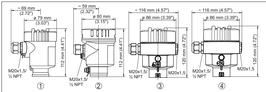
Rys. 17: Wersje wykonania obudowy
