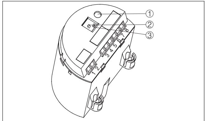
Rys. 10: Moduł elektroniczny SWE60R - wyjście przekaźnikowe
