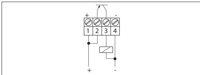
Fig. 10: PNP action
