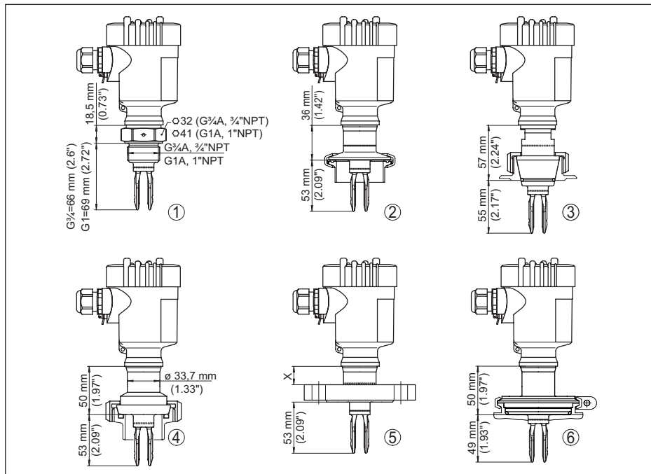
Fig. 21: VEGASWING 61
