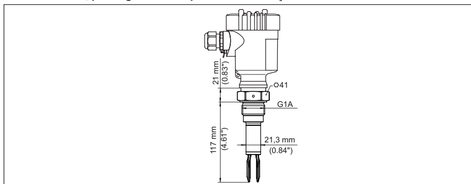
Fig. 23: Prolongamento do ponto de comutação - para trocar facilmente o VEGASWING ou 81 A
