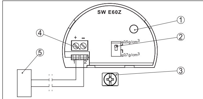
Fig. 8: Compartimento do sistema eletrônico e de conexão
