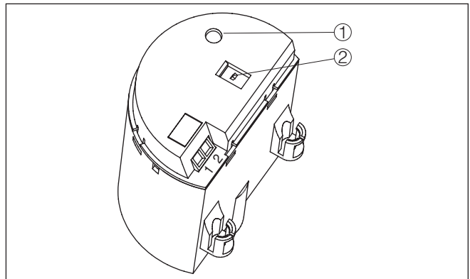
Fig. 11: Módulo eletrônico SWE60Z - Saída de dois condutores
