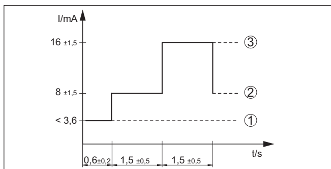
Fig. 12: Diagrama do teste de funcionamento
