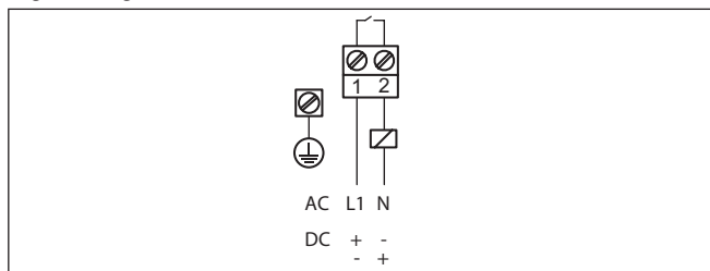
Fig. 11: Schéma de raccordement boîtier à chambre unique
