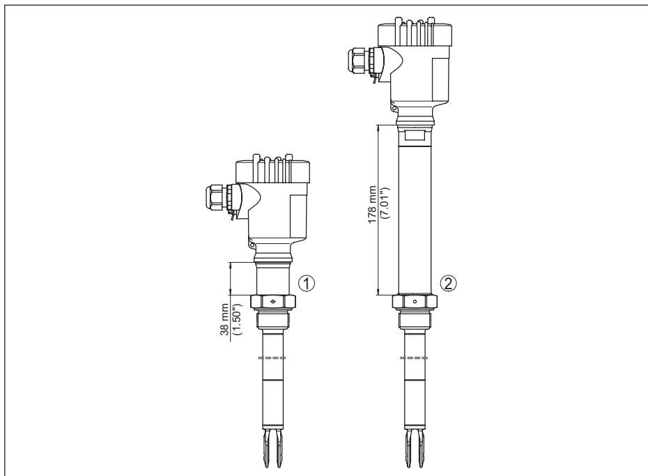
Fig. 21: Options 1)
