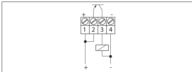
Fig. 12: PNP action
