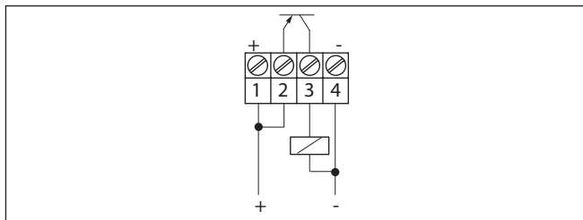
Fig. 12: Comportement PNP
