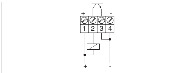
Fig. 11: Comportement NPN
